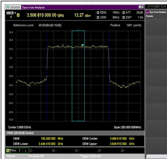
NTNV_N78-3450-3550_PC2_30_100_L_TID1_Ant1#1
