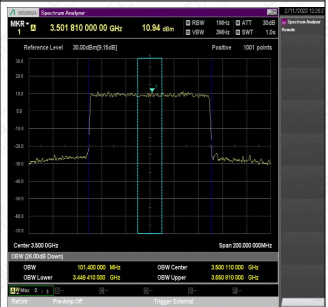
NTNV_N78-3450-3550_PC2_30_100_L_TID8_Ant1#1
