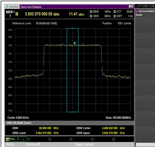
NTNV_N78-3450-3550_PC2_30_90_M_TID7_Ant1#1
