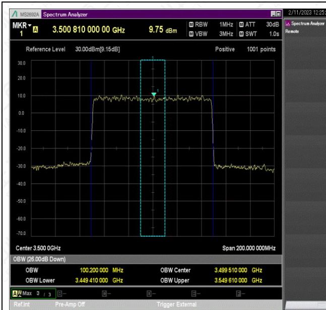
NTNV_N78-3450-3550_PC2_30_100_L_TID5_Ant1#1
