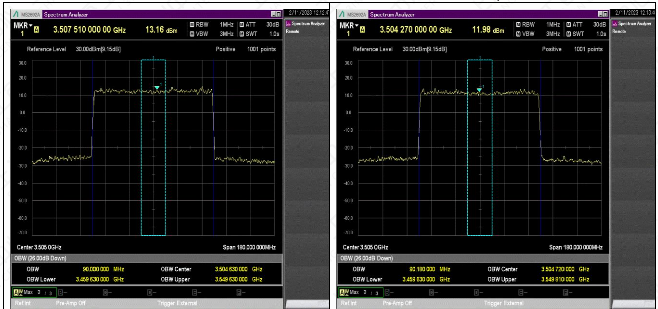
NTNV_N78-3450-3550_PC2_30_90_H_TID2_Ant1#1
