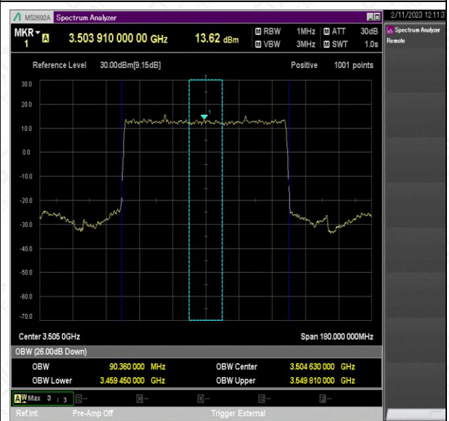
NTNV_N78-3450-3550_PC2_30_90_H_TID1_Ant1#1
