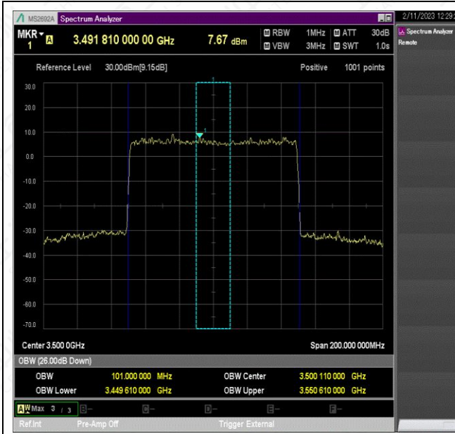
NTNV_N78-3450-3550_PC2_30_100_L_TID9_Ant1#1
