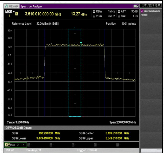
NTNV_N78-3450-3550_PC2_30_100_H_TID2_Ant1#1
