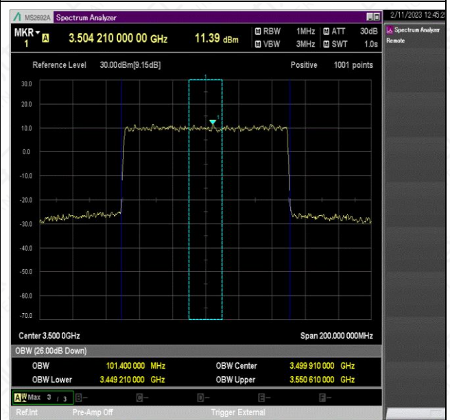
NTNV_N78-3450-3550_PC2_30_100_H_TID6_Ant1#1
