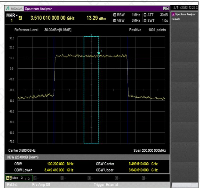
NTNV_N78-3450-3550_PC2_30_100_L_TID2_Ant1#1
