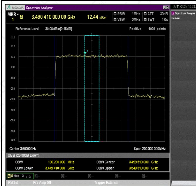
NTNV_N78-3450-3550_PC2_30_100_L_TID3_Ant1#1
