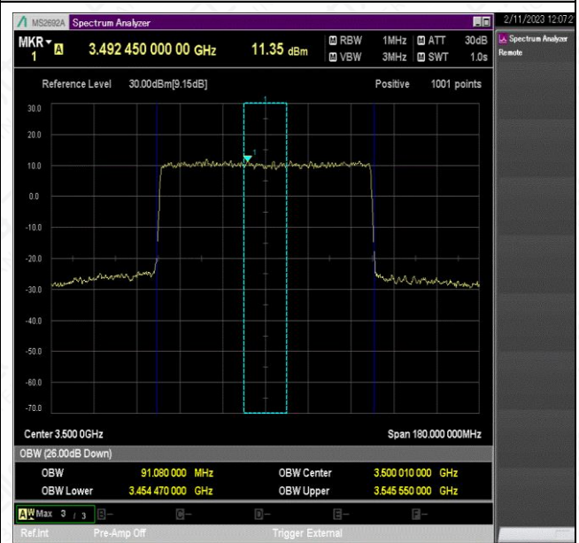
NTNV_N78-3450-3550_PC2_30_90_M_TID6_Ant1#1
