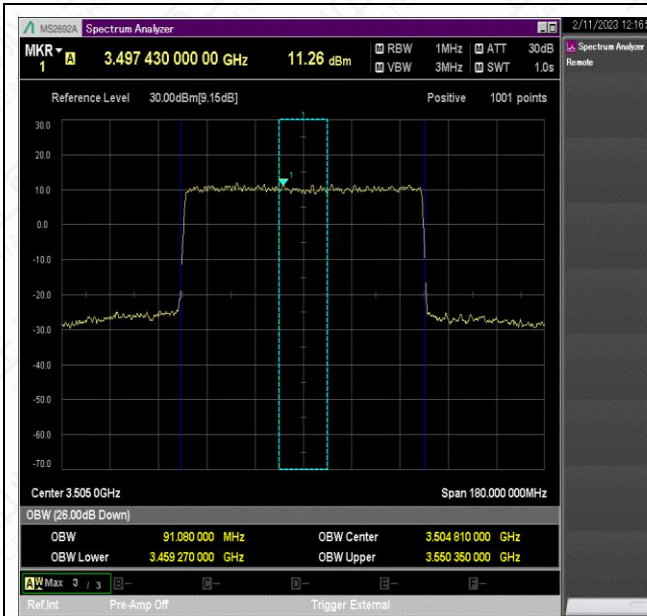
NTNV_N78-3450-3550_PC2_30_90_H_TID6_Ant1#1
