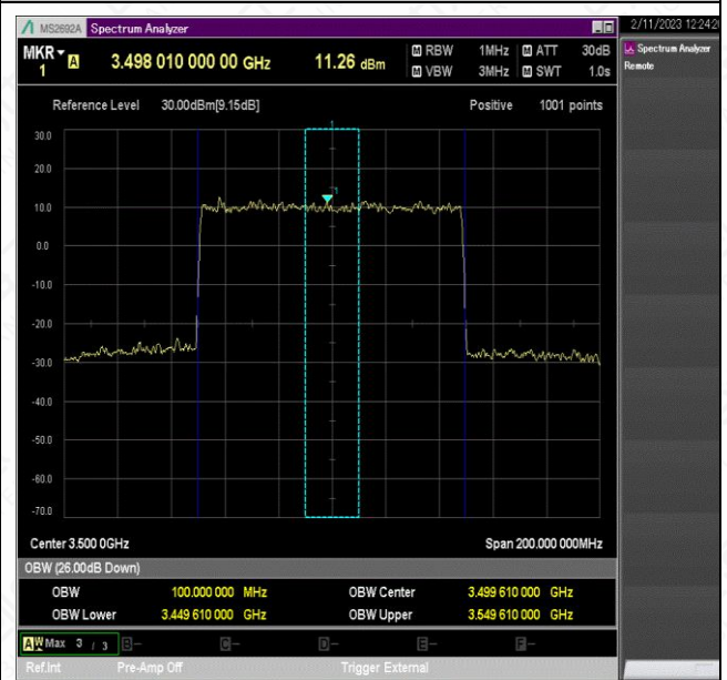
NTNV_N78-3450-3550_PC2_30_100_L_TID4_Ant1#1
