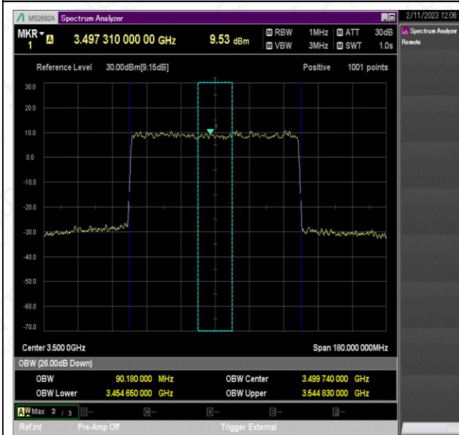
NTNV_N78-3450-3550_PC2_30_90_M_TID5_Ant1#1
