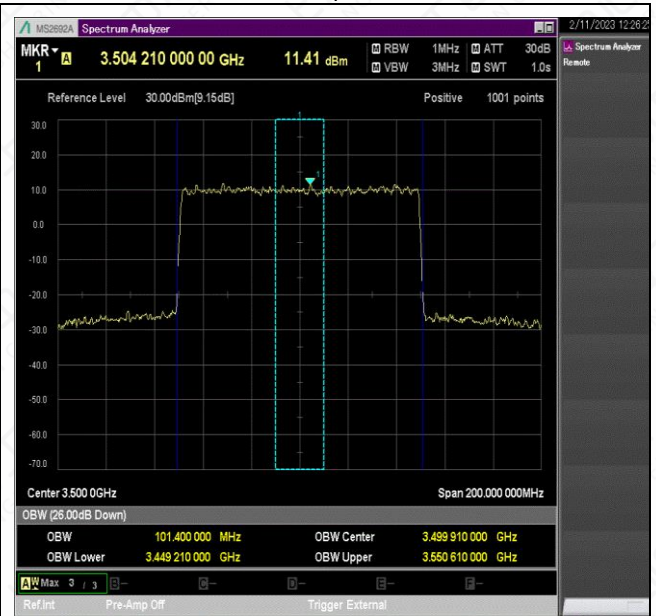
NTNV_N78-3450-3550_PC2_30_100_L_TID6_Ant1#1
