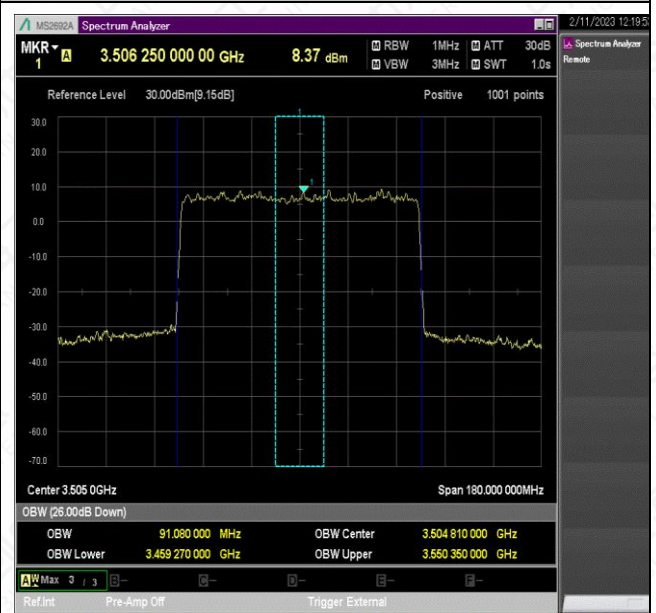
NTNV_N78-3450-3550_PC2_30_90_H_TID9_Ant1#1
