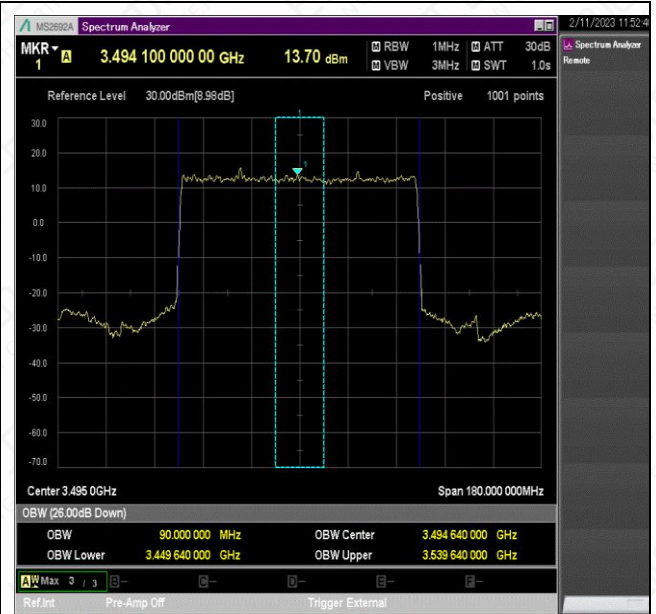
NTNV_N78-3450-3550_PC2_30_90_L_TID1_Ant1#1
