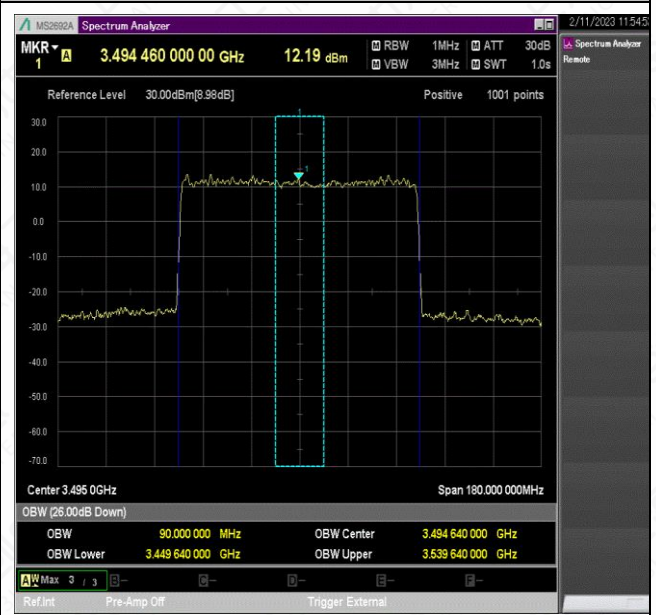
NTNV_N78-3450-3550_PC2_30_90_L_TID3_Ant1#1
