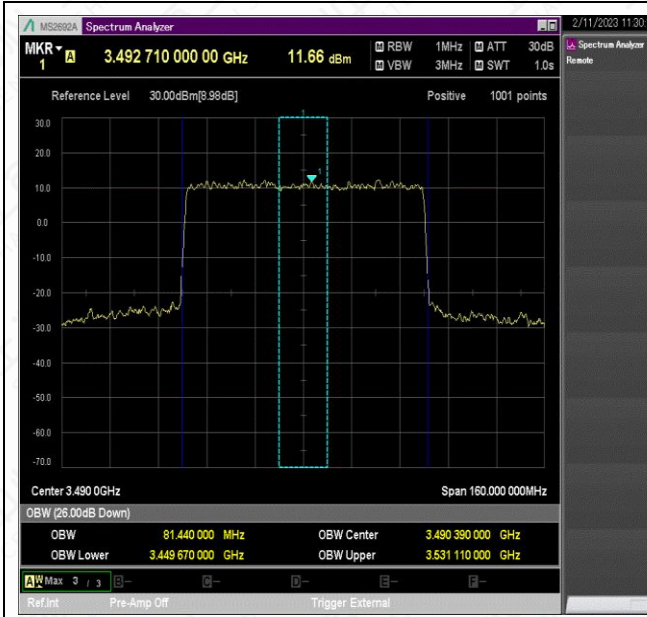
NTVN_N78-3450-3550_PC2_30_80_L_TID7_Ant1#1
