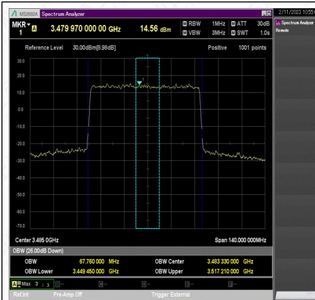
NTNV_N78-3450-3550_PC2_30_70_L_TID2_Ant1#1
