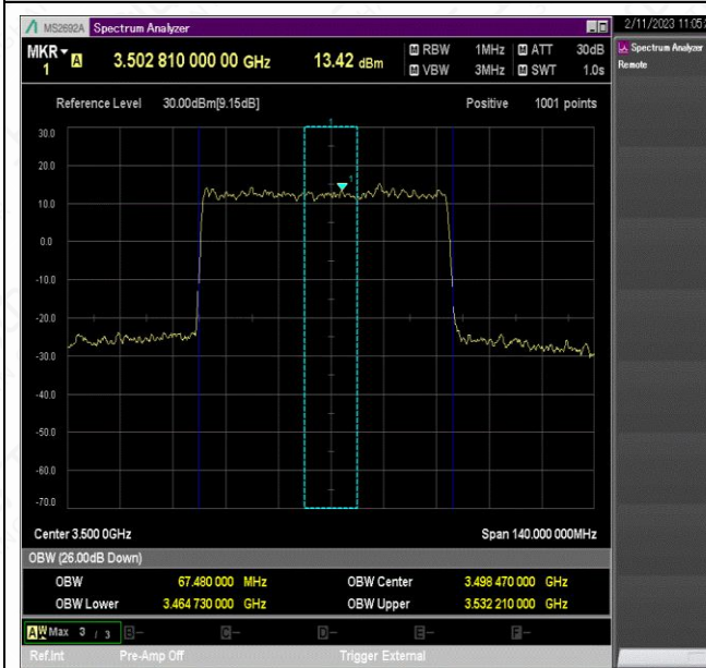
NTNV_N78-3450-3550_PC2_30_70_M_TID3_Ant1#1
