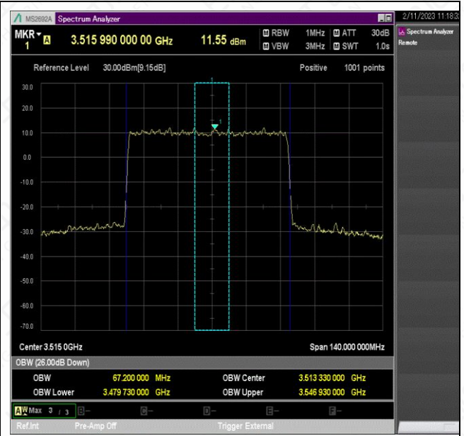
NTNV_N78-3450-3550_PC2_30_70_H_TID5_Ant1#1
