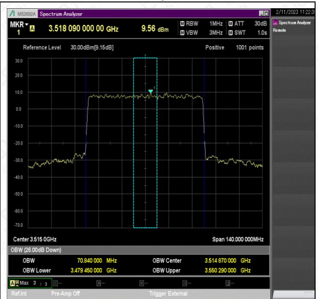
NTNV_N78-3450-3550_PC2_30_70_H_TID9_Ant1#1
