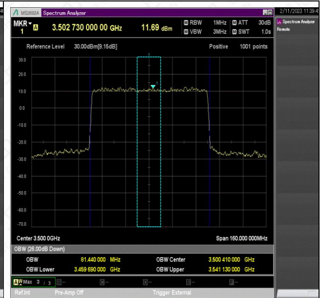
NTV_N78-3450-3550_PC2_30_80_M_TID7_Ant1#1
