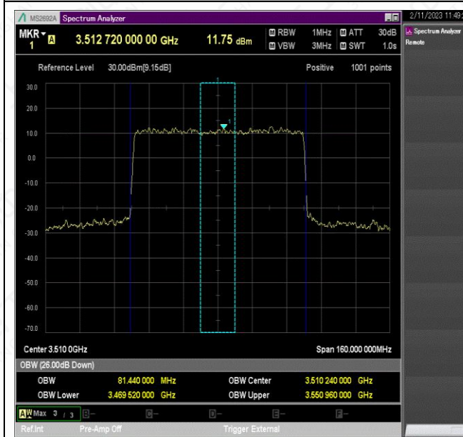
NTNV_N78-3450-3550_PC2_30_80_H_TID7_Ant1#1
