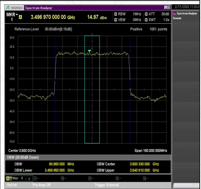
NTVN_N78-3450-3550_PC2_30_80_M_TID1_Ant1#1
