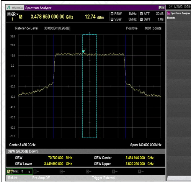
NTNV_N78-3450-3550_PC2_30_70_L_TID6_Ant1#1
