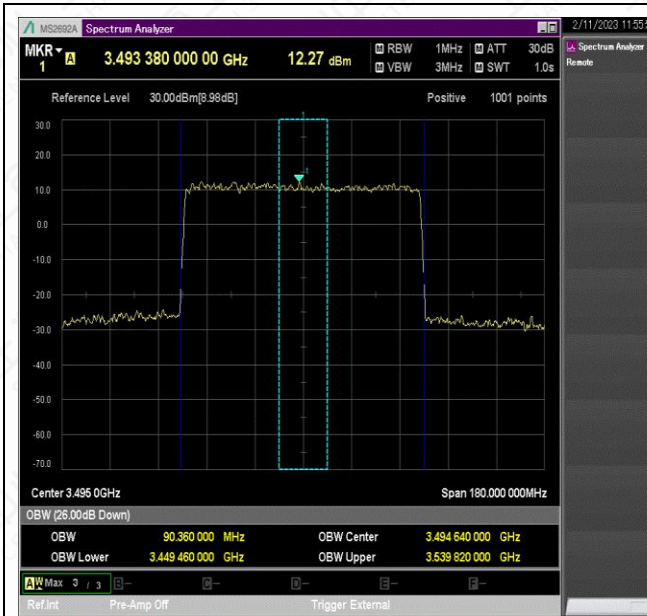
NTNV_N78-3450-3550_PC2_30_90_L_TID4_Ant1#1
