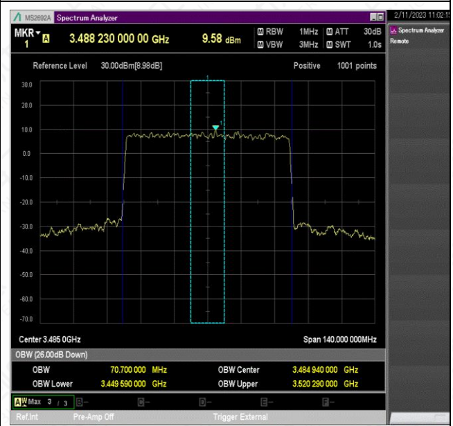
NTNV_N78-3450-3550_PC2_30_70_L_TID9_Ant1#1
