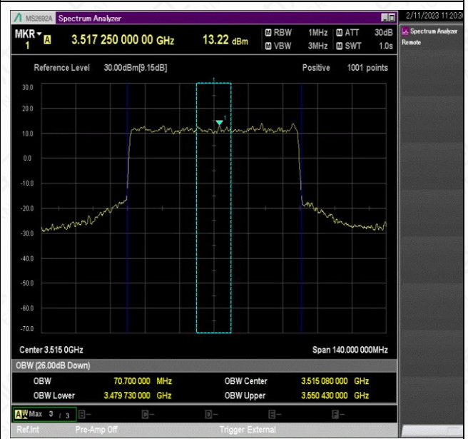
NTNV_N78-3450-3550_PC2_30_70_H_TID7_Ant1#1
