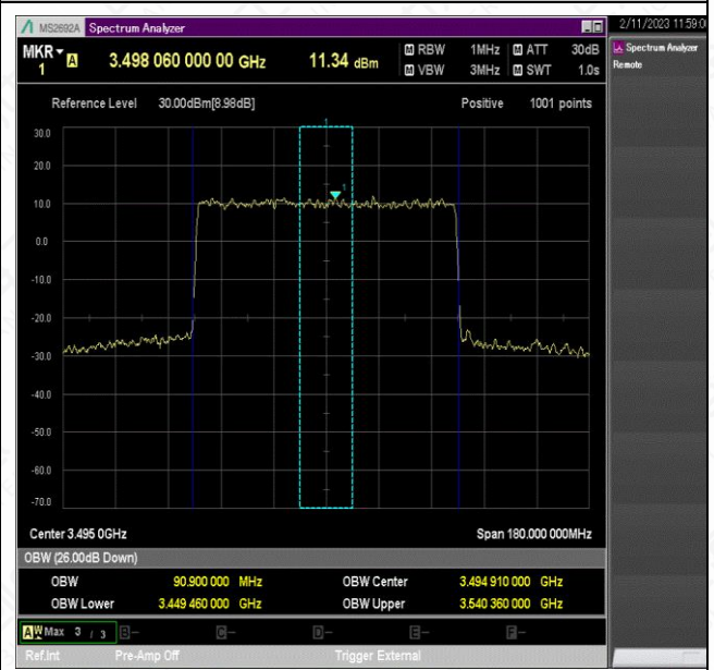
NTNV_N78-3450-3550_PC2_30_90_L_TID7_Ant1#1
