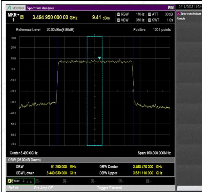
NTVN_N78-3450-3550_PC2_30_80_L_TID9_Ant1#1
