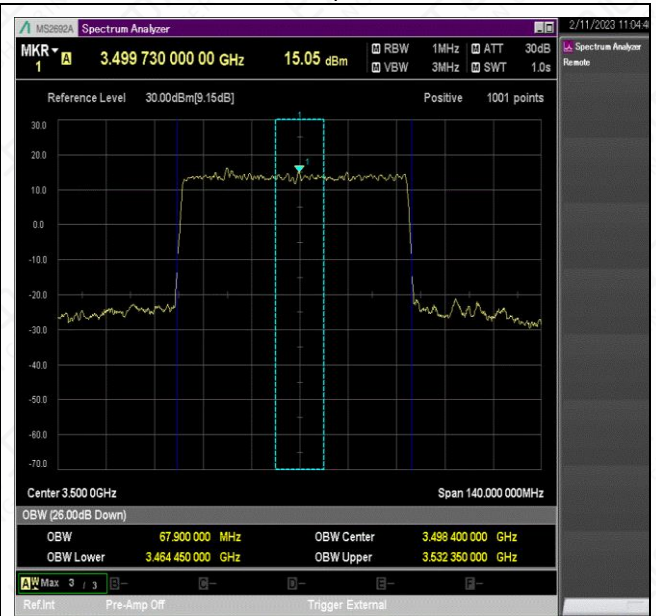
NTNV_N78-3450-3550_PC2_30_70_M_TID2_Ant1#1
