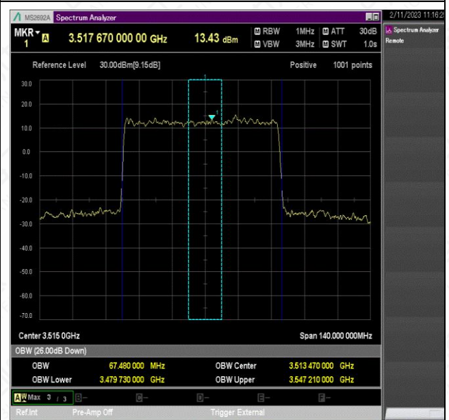
NTNV_N78-3450-3550_PC2_30_70_H_TID3_Ant1#1
