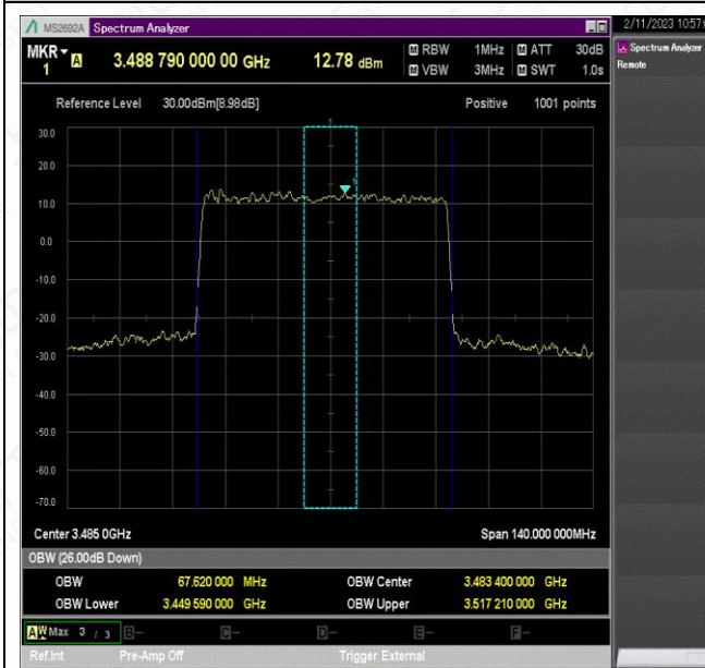
NTNV_N78-3450-3550_PC2_30_70_L_TID4_Ant1#1
