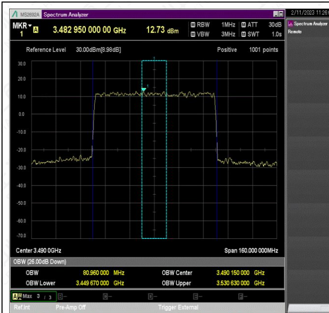
NTNV_N78-3450-3550_PC2_30_80_L_TID3_Ant1#1
