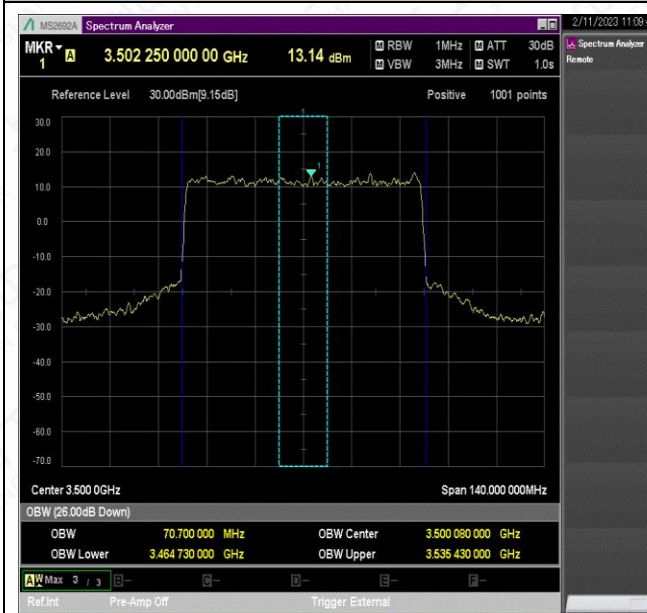
NTV_N78-3450-3550_PC2_30_70_M_TID7_Ant1#1
