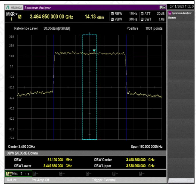
NTNV_N78-3450-3550_PC2_30_80_L_TID2_Ant1#1
