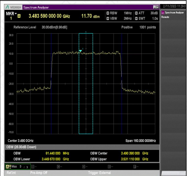
NTNV_N78-3450-3550_PC2_30_80_L_TID6_Ant1#1
