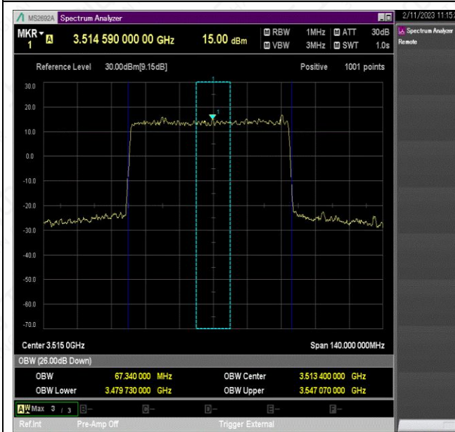
NTNV_N78-3450-3550_PC2_30_70_H_TID2_Ant1#1
