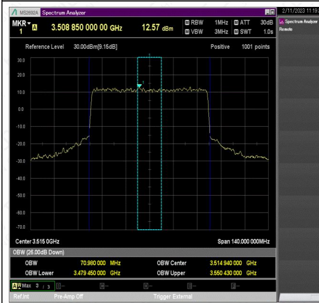
NTNV_N78-3450-3550_PC2_30_70_H_TID6_Ant1#1
