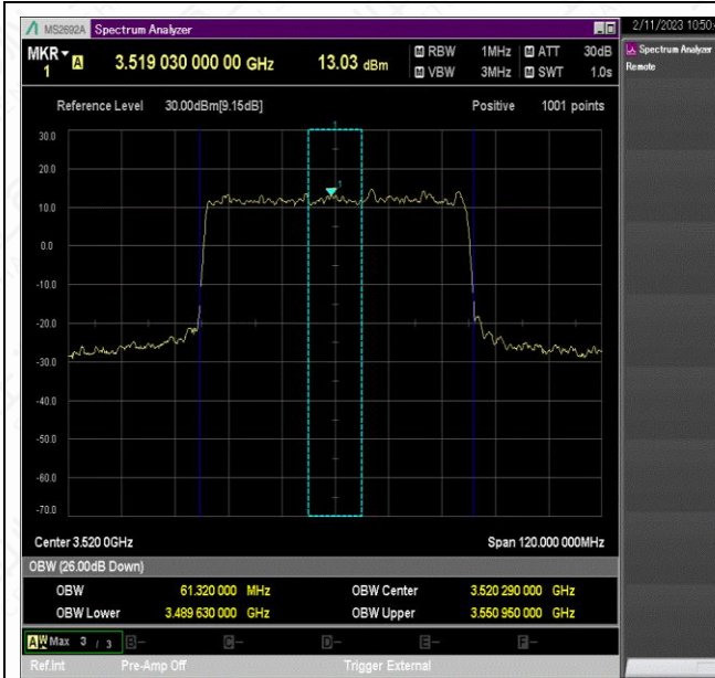
NTNV_N78-3450-3550_PC2_30_60_H_TID7_Ant1#1
