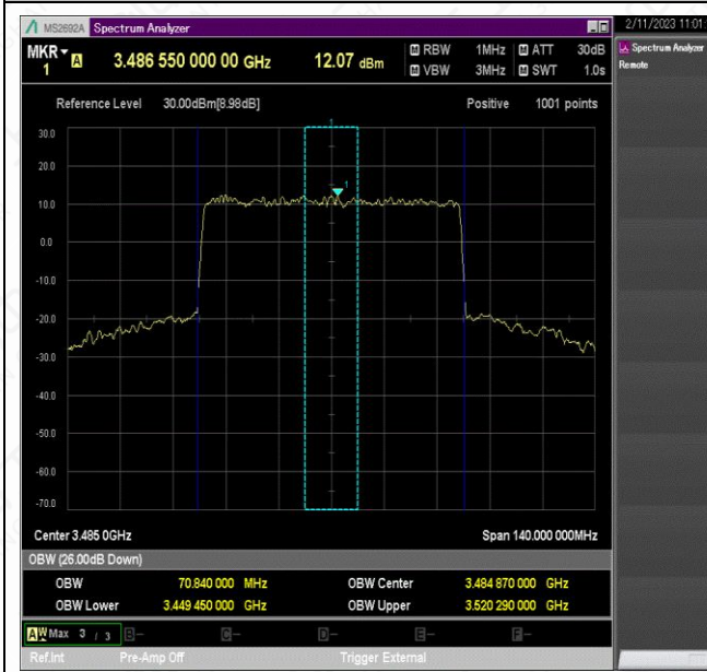
NTNV_N78-3450-3550_PC2_30_70_L_TID8_Ant1#1
