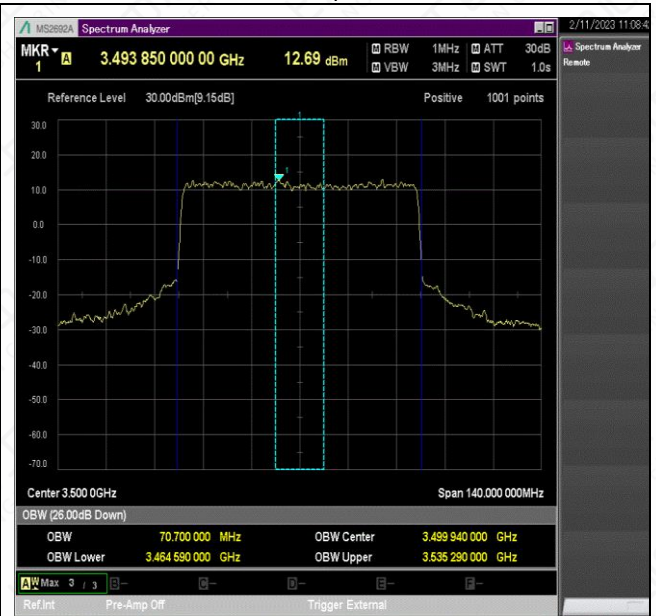
NTV_N78-3450-3550_PC2_30_70_M_TID6_Ant1#1
