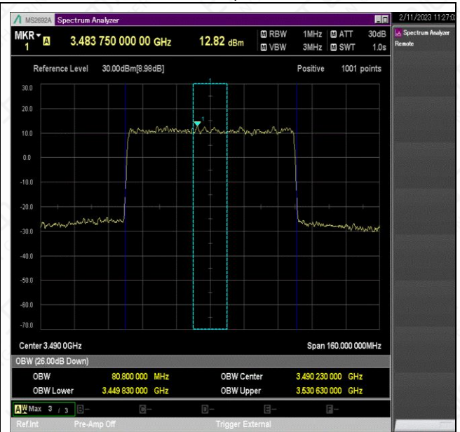
NTNV_N78-3450-3550_PC2_30_80_L_TID4_Ant1#1
