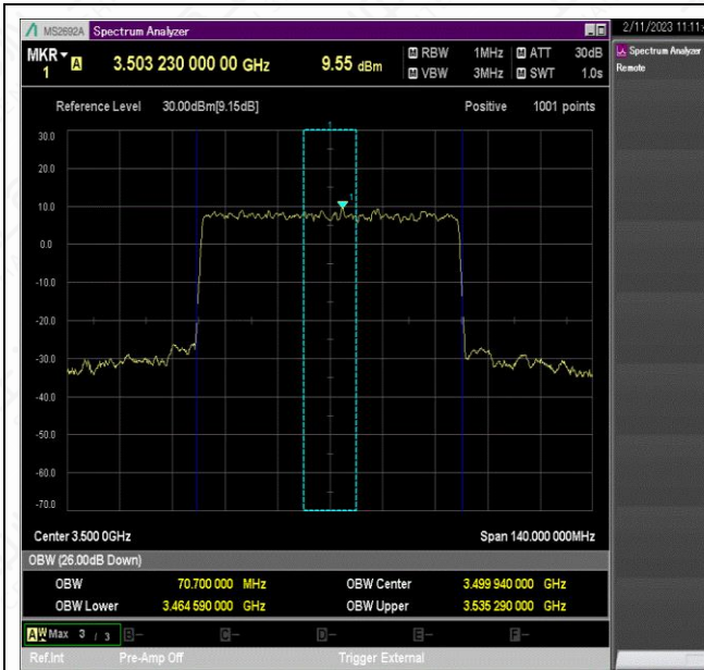
NTNV_N78-3450-3550_PC2_30_70_M_TID9_Ant1#1
