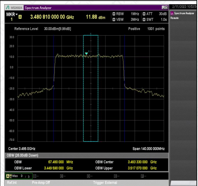
NTNV_N78-3450-3550_PC2_30_70_L_TID1_Ant1#1
