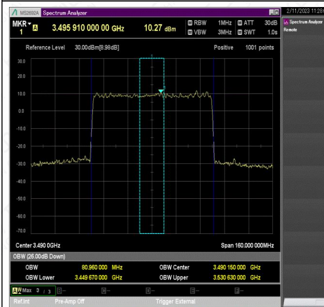
NTNV_N78-3450-3550_PC2_30_80_L_TID5_Ant1#1
