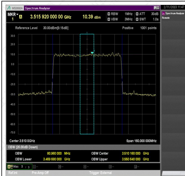
NTNV_N78-3450-3550_PC2_30_80_H_TID5_Ant1#1
