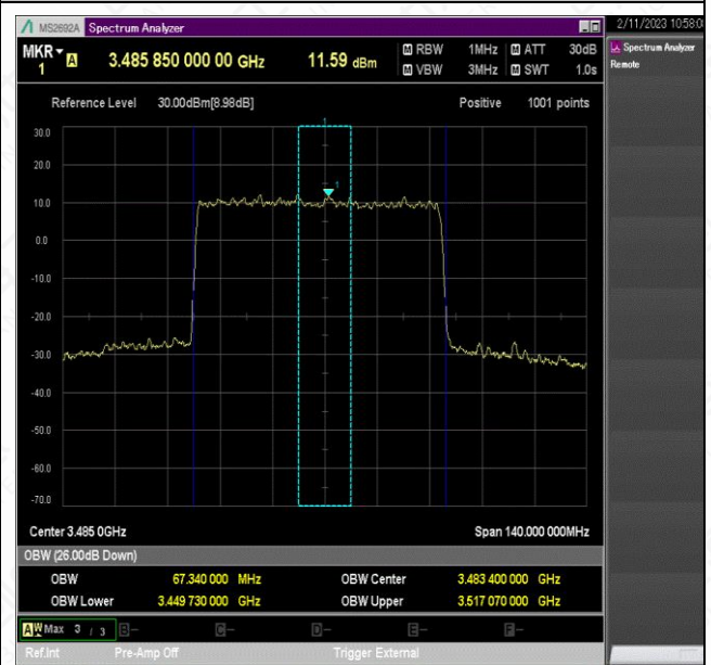
NTNV_N78-3450-3550_PC2_30_70_L_TID5_Ant1#1
