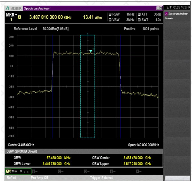
NTNV_N78-3450-3550_PC2_30_70_L_TID3_Ant1#1
