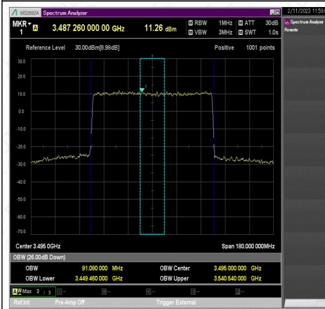
NTNV_N78-3450-3550_PC2_30_90_L_TID6_Ant1#1
