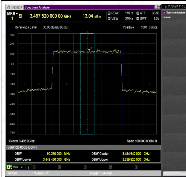
NTNV_N78-3450-3550_PC2_30_90_L_TID2_Ant1#1
