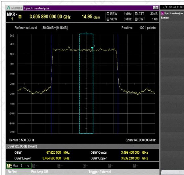
NTNV_N78-3450-3550_PC2_30_70_M_TID1_Ant1#1
