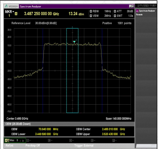
NTNV_N78-3450-3550_PC2_30_70_L_TID7_Ant1#1
