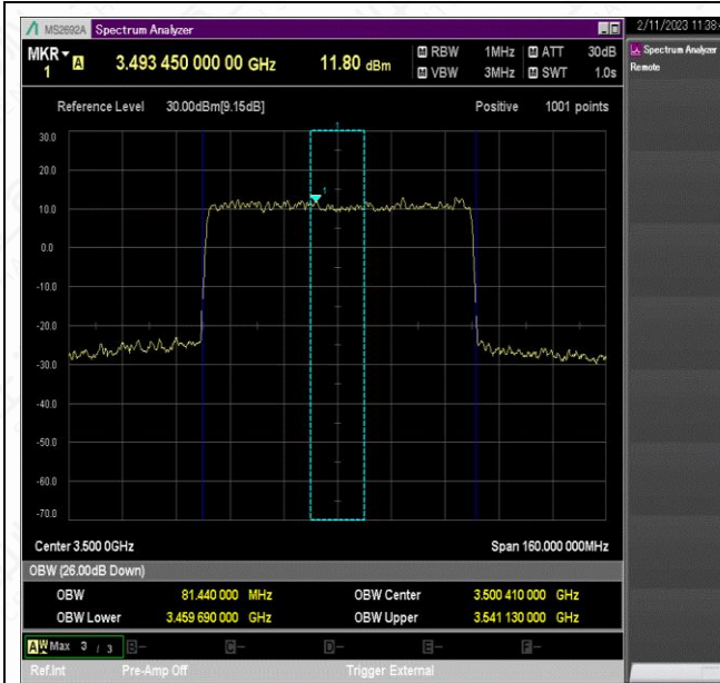
NTV_N78-3450-3550_PC2_30_80_M_TID6_Ant1#1
