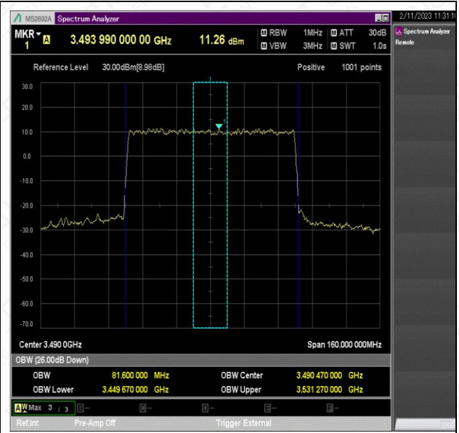
NTVN_N78-3450-3550_PC2_30_80_L_TID8_Ant1#1
