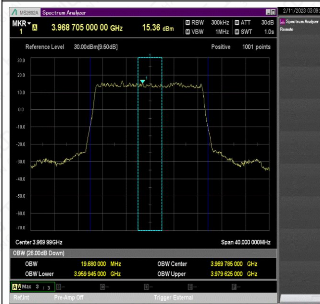
NTNV_N77-3700-3980_PC2_30_20_H_TID1_Ant1#1
