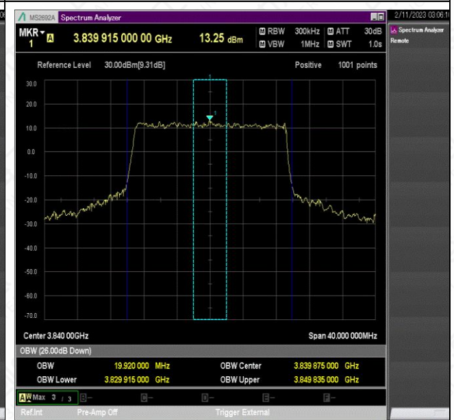
NTNV_N77-3700-3980_PC2_30_20_M_TID7_Ant1#1
