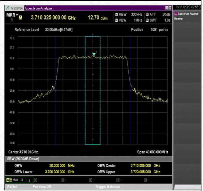
NTNV_N77-3700-3980_PC2_30_20_L_TID6_Ant1#1
