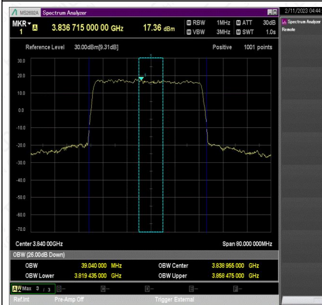
NTVN_N77-3700-3980_PC2_30_40_M_TID2_Ant1#1
