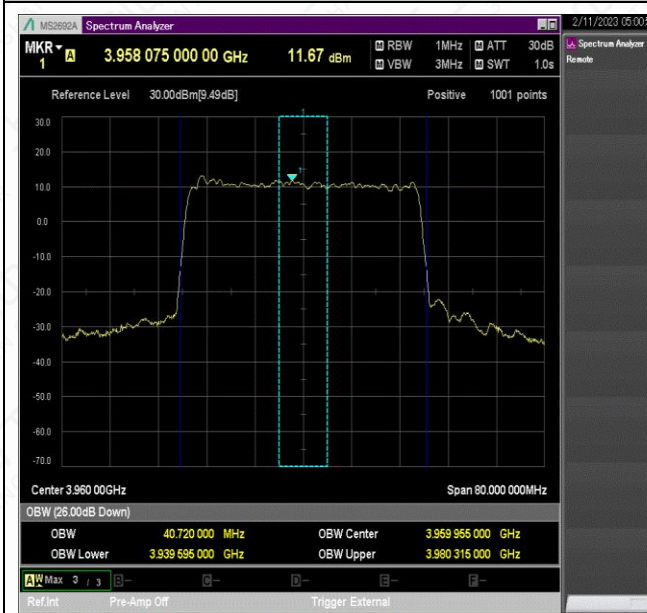
NTNV_N77-3700-3980_PC2_30_40_H_TID9_Ant1#1
