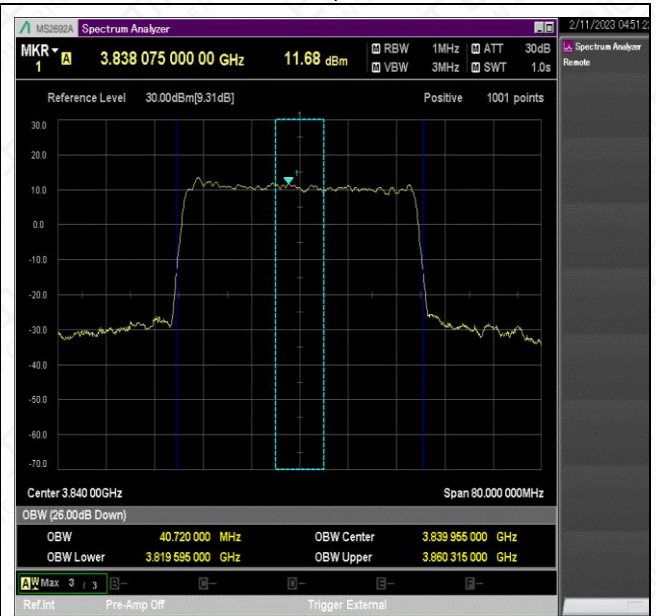
NTNV_N77-3700-3980_PC2_30_40_M_TID9_Ant1#1
