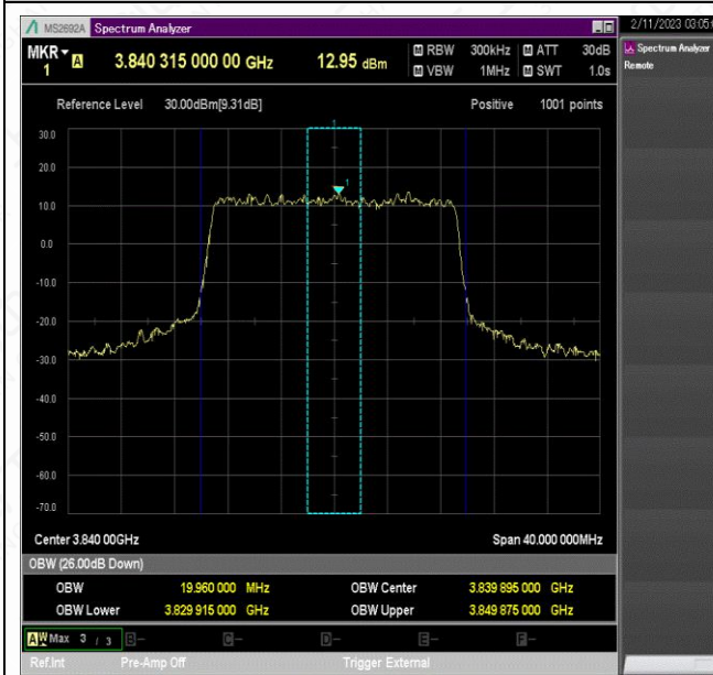
NTNV_N77-3700-3980_PC2_30_20_M_TID6_Ant1#1
