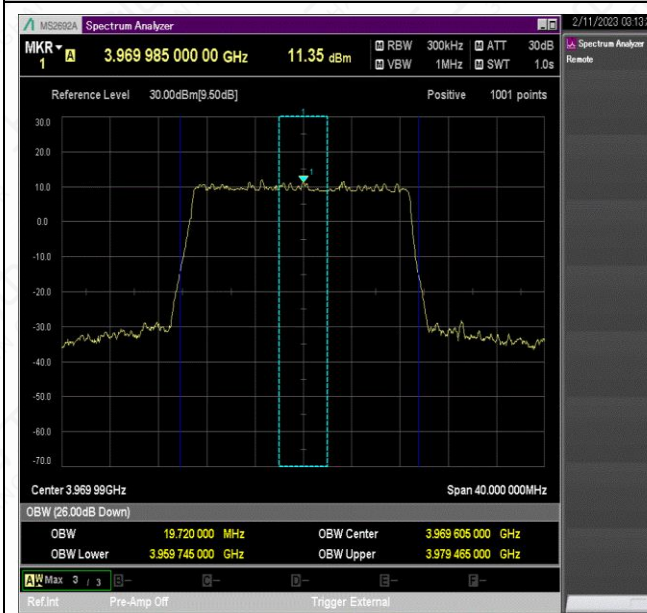
NTNV_N77-3700-3980_PC2_30_20_H_TID5_Ant1#1
