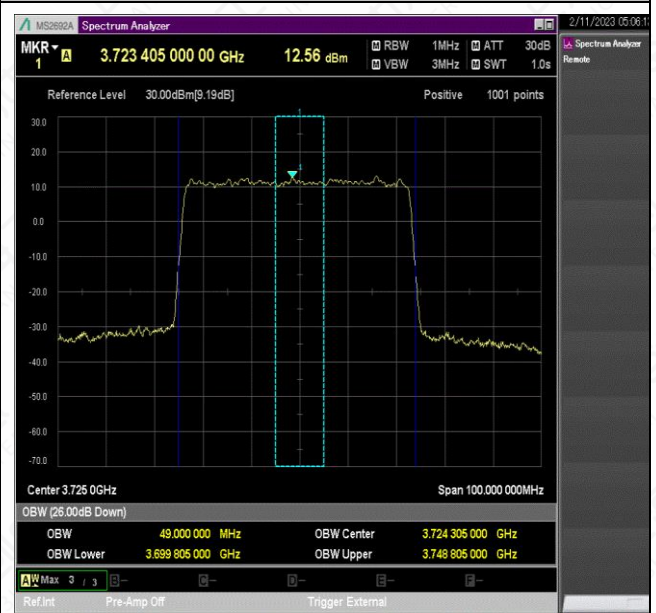
NTNV_N77-3700-3980_PC2_30_50_L_TID5_Ant1#1
