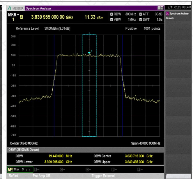
NTNV_N77-3700-3980_PC2_30_20_M_TID5_Ant1#1
