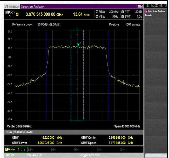
NTNV_N77-3700-3980_PC2_30_20_H_TID6_Ant1#1
