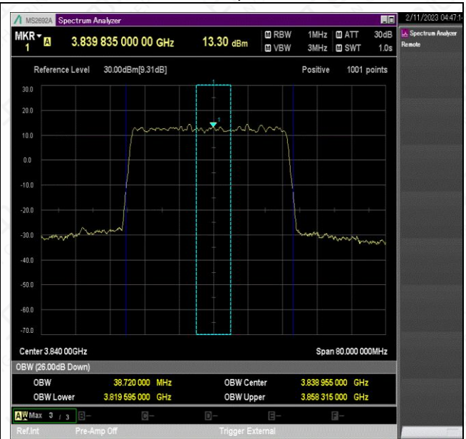
NTNV_N77-3700-3980_PC2_30_40_M_TID5_Ant1#1
