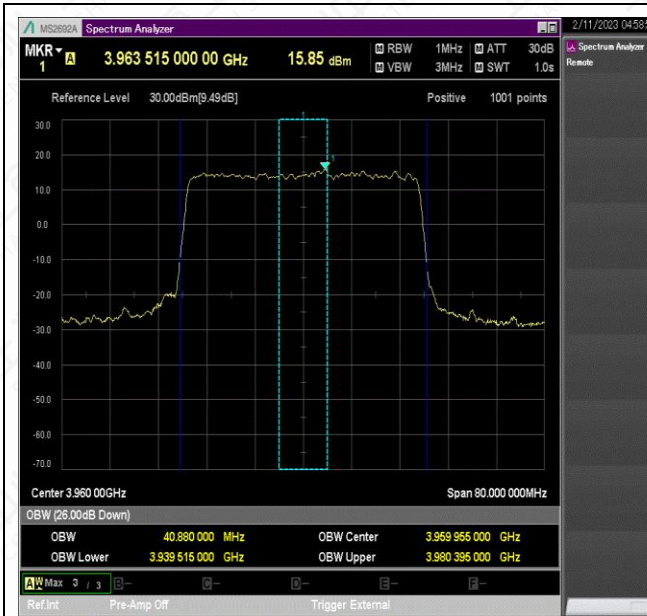
NTNV_N77-3700-3980_PC2_30_40_H_TID7_Ant1#1
