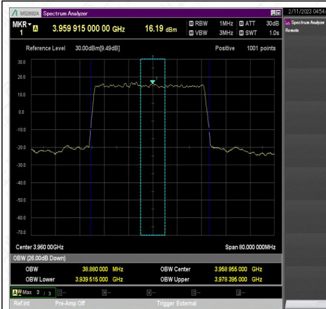
NTNV_N77-3700-3980_PC2_30_40_H_TID3_Ant1#1
