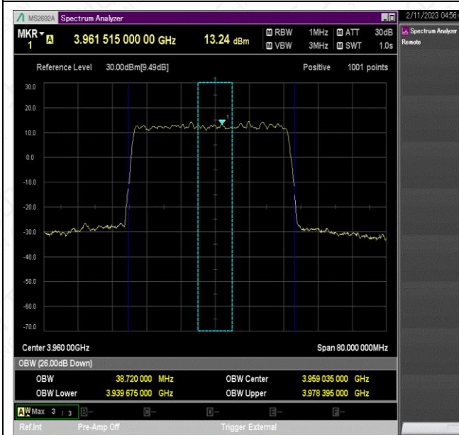
NTNV_N77-3700-3980_PC2_30_40_H_TID5_Ant1#1
