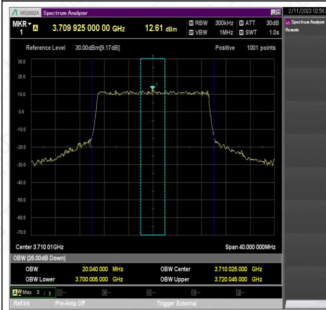
NTNV_N77-3700-3980_PC2_30_20_L_TID7_Ant1#1
