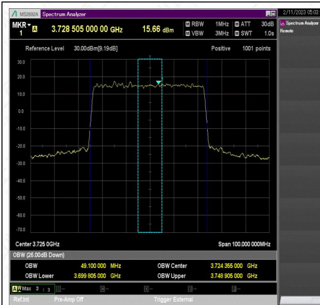
NTNV_N77-3700-3980_PC2_30_50_L_TID2_Ant1#1
