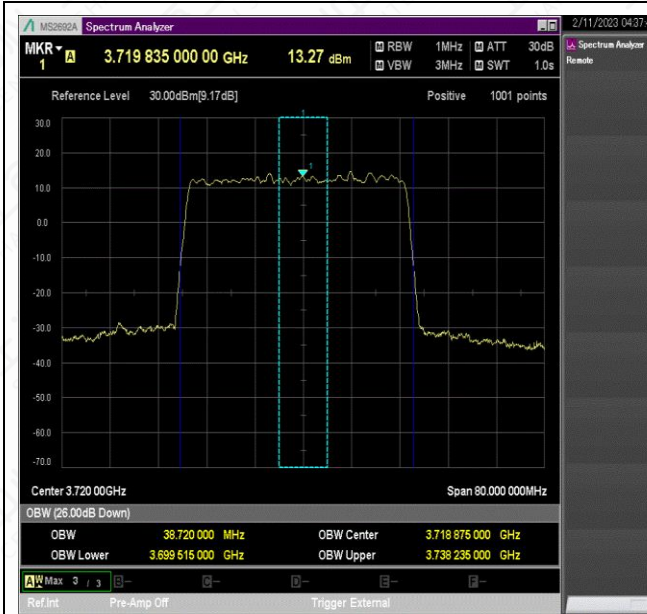
NTNV_N77-3700-3980_PC2_30_40_L_TID5_Ant1#1
