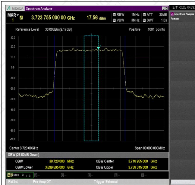
NTNV_N77-3700-3980_PC2_30_40_L_TID1_Ant1#1
