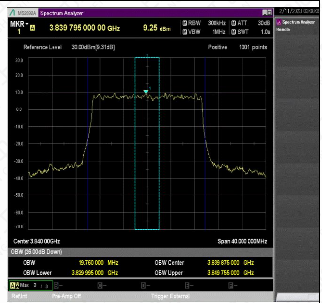
NTNV_N77-3700-3980_PC2_30_20_M_TID9_Ant1#1
