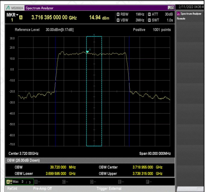
NTNV_N77-3700-3980_PC2_30_40_L_TID4_Ant1#1
