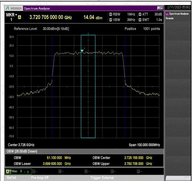
NTNV_N77-3700-3980_PC2_30_50_L_TID7_Ant1#1
