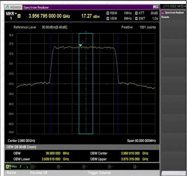
NTNV_N77-3700-3980_PC2_30_40_H_TID2_Ant1#1
