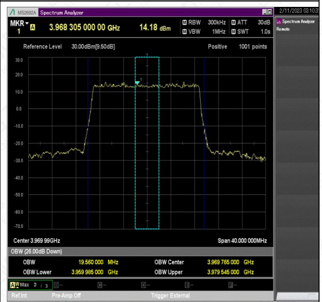
NTNV_N77-3700-3980_PC2_30_20_H_TID2_Ant1#1
