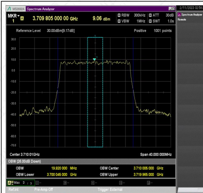
NTVN_N77-3700-3980_PC2_30_20_L_TID9_Ant1#1
