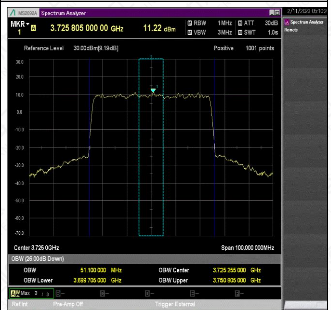
NTNV_N77-3700-3980_PC2_30_50_L_TID9_Ant1#1
