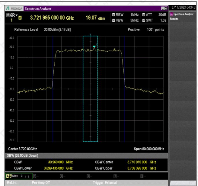
NTNV_N77-3700-3980_PC2_30_40_L_TID2_Ant1#1
