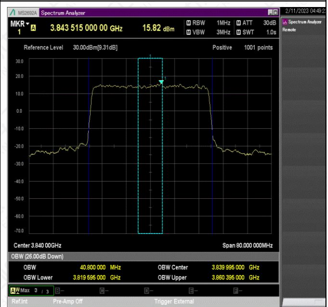
NTNV_N77-3700-3980_PC2_30_40_M_TID7_Ant1#1
