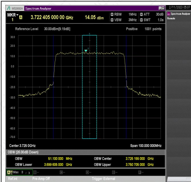
NTNV_N77-3700-3980_PC2_30_50_L_TID6_Ant1#1
