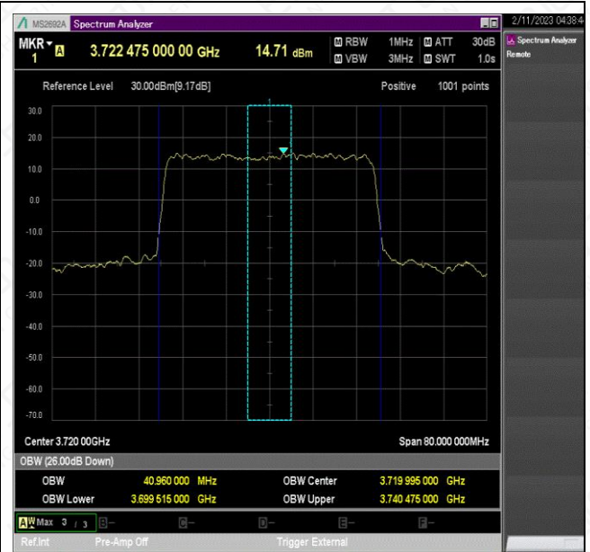
NTNV_N77-3700-3980_PC2_30_40_L_TID6_Ant1#1
