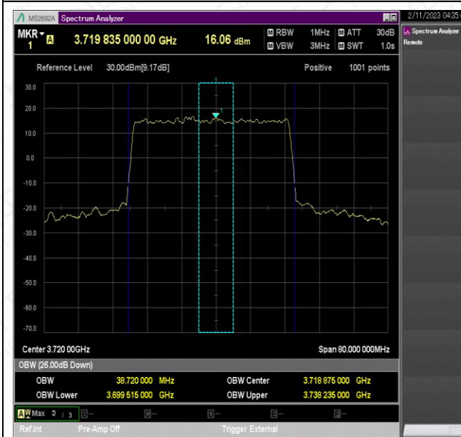
NTNV_N77-3700-3980_PC2_30_40_L_TID3_Ant1#1
