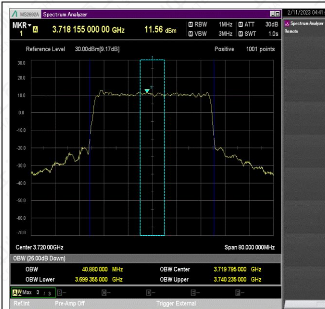
NTVN_N77-3700-3980_PC2_30_40_L_TID9_Ant1#1
