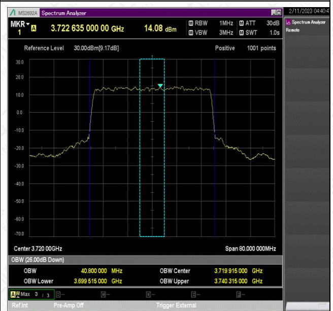
NTNV_N77-3700-3980_PC2_30_40_L_TID8_Ant1#1
