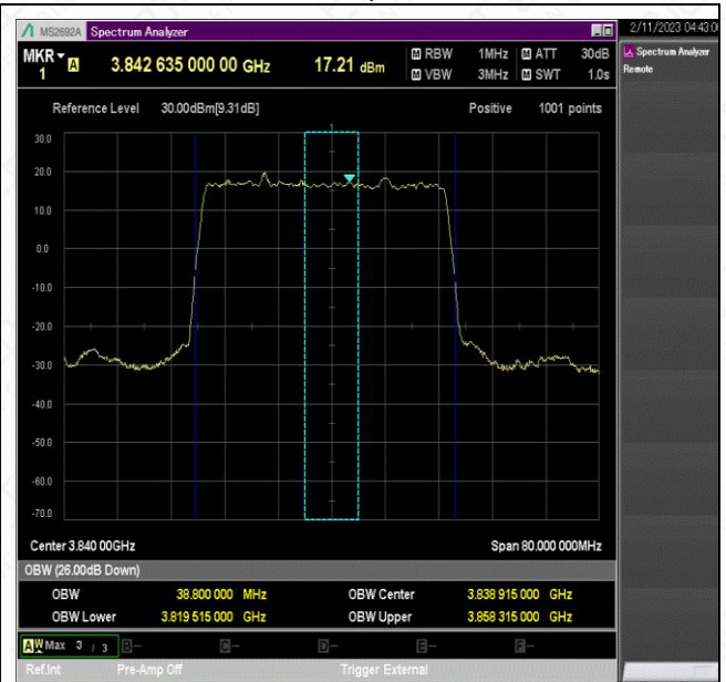
NTVN_N77-3700-3980_PC2_30_40_M_TID1_Ant1#1
