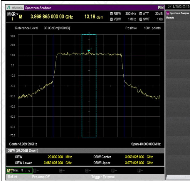
NTNV_N77-3700-3980_PC2_30_20_H_TID7_Ant1#1
