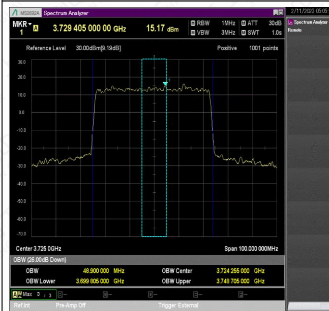
NTNV_N77-3700-3980_PC2_30_50_L_TID4_Ant1#1
