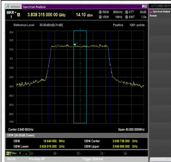
NTVN_N77-3700-3980_PC2_30_20_M_TID2_Ant1#1
