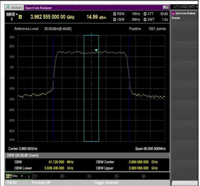
NTNV_N77-3700-3980_PC2_30_40_H_TID6_Ant1#1
