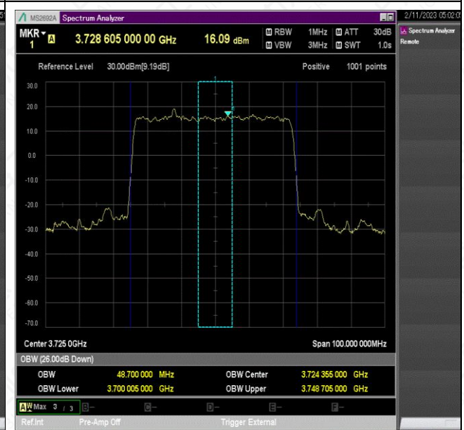
NTNV_N77-3700-3980_PC2_30_50_L_TID1_Ant1#1
