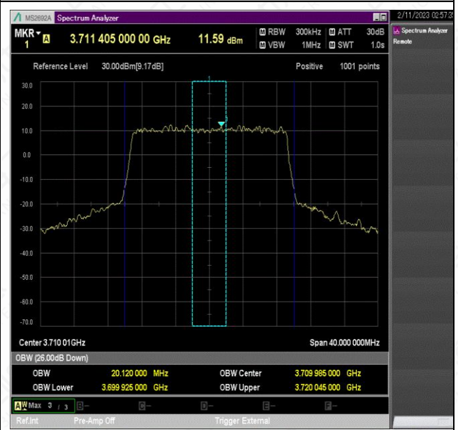
NTNV_N77-3700-3980_PC2_30_20_L_TID8_Ant1#1
