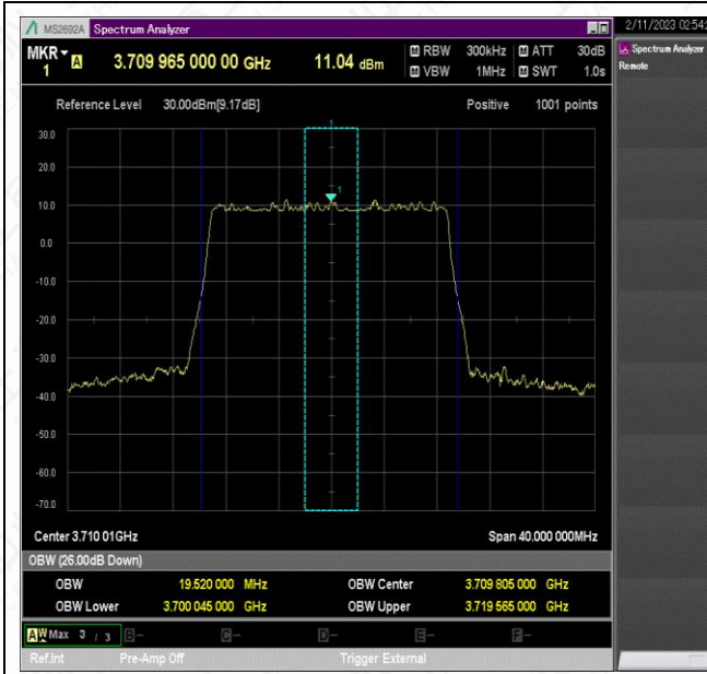
NTNV_N77-3700-3980_PC2_30_20_L_TID5_Ant1#1
