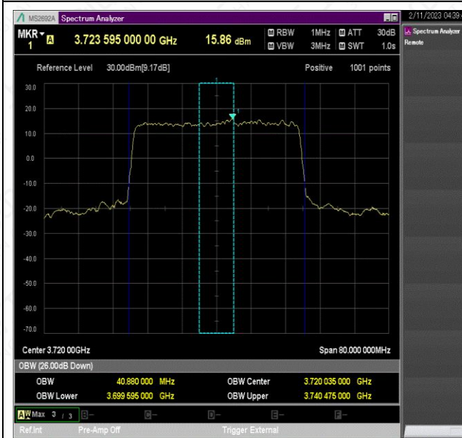
NTNV_N77-3700-3980_PC2_30_40_L_TID7_Ant1#1
