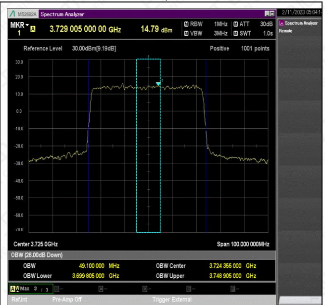
NTNV_N77-3700-3980_PC2_30_50_L_TID3_Ant1#1
