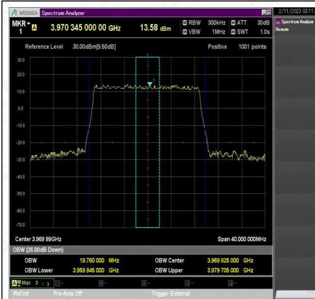
NTNV_N77-3700-3980_PC2_30_20_H_TID3_Ant1#1
