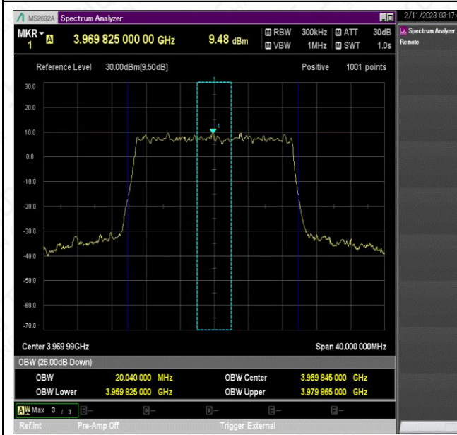
NTNV_N77-3700-3980_PC2_30_20_H_TID9_Ant1#1
