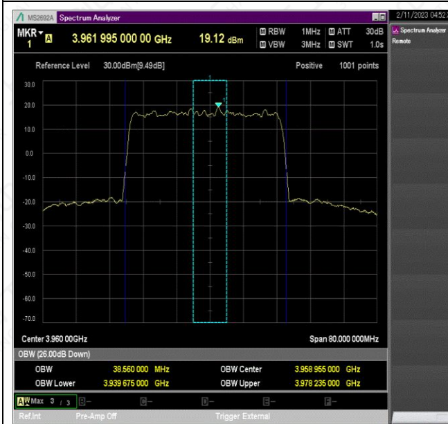
NTNV_N77-3700-3980_PC2_30_40_H_TID1_Ant1#1
