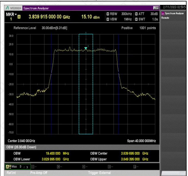
NTVN_N77-3700-3980_PC2_30_20_M_TID1_Ant1#1
