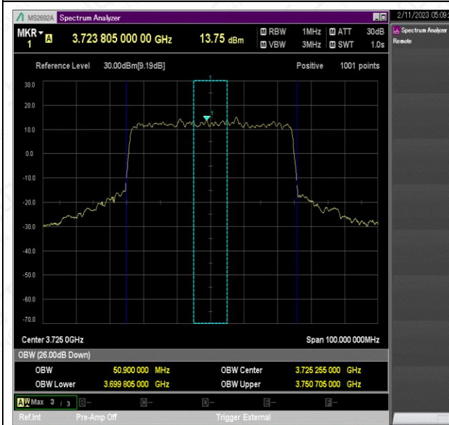
NTNV_N77-3700-3980_PC2_30_50_L_TID8_Ant1#1
