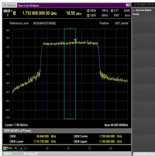
NTNV_N66_PC3_15_40_L_TID8_Ant1#1
