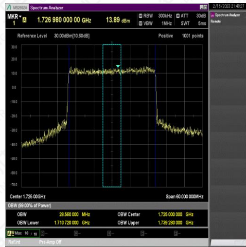
NTNV_N66_PC3_15_30_L_TID2_Ant1#1
