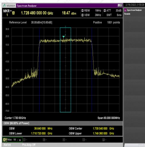
NTNV_N66_PC3_15_40_L_TID4_Ant1#1
