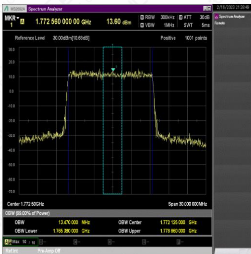
NTNV_N66_PC3_15_15_H_TID3_Ant1#1
