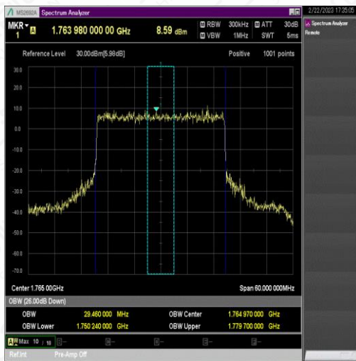
NTNV_N66_PC3_15_30_H_TID7_Ant1#1
