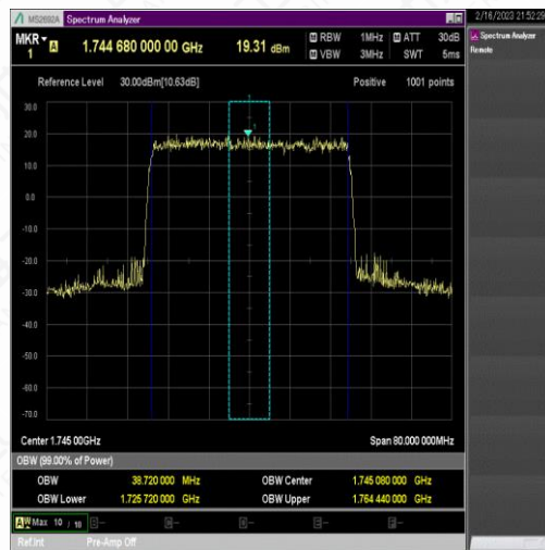
NTNV_N66_PC3_15_40_M_TID2_Ant1#1
