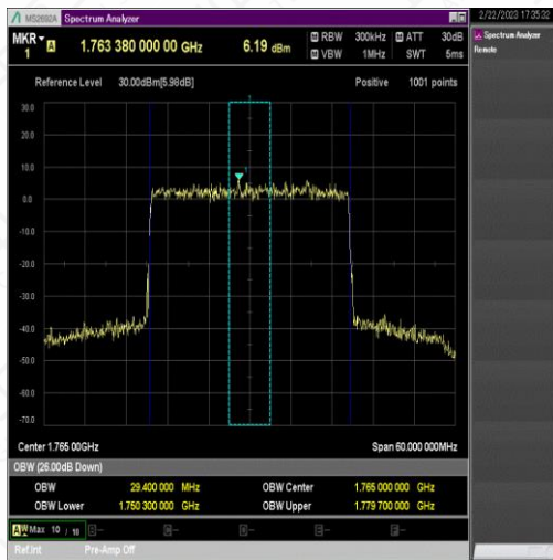
NTNV_N66_PC3_15_30_H_TID9_Ant1#1
