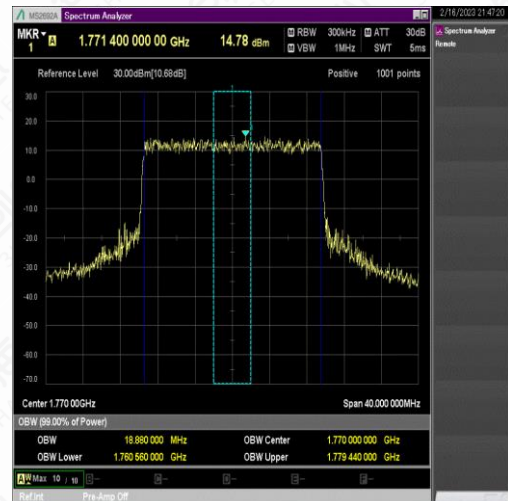
NTNV_N66_PC3_15_20_H_TID7_Ant1#1
