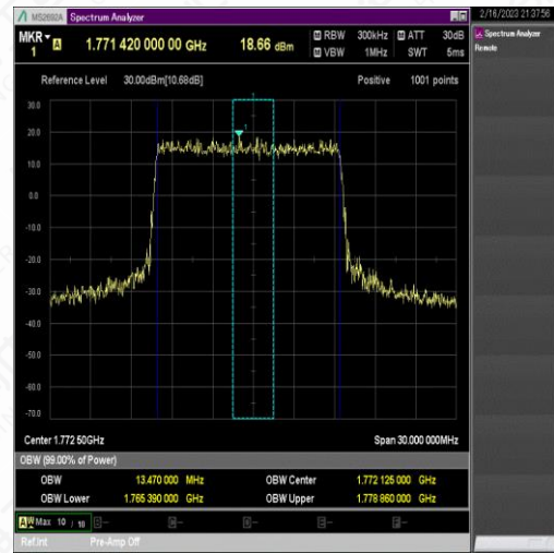
NTNV_N66_PC3_15_15_H_TID2_Ant1#1
