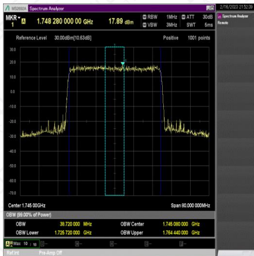
NTNV_N66_PC3_15_40_M_TID3_Ant1#1
