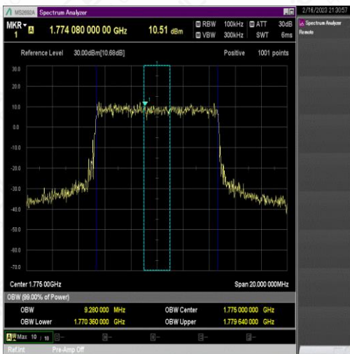
NTNV_N66_PC3_15_10_H_TID6_Ant1#1
