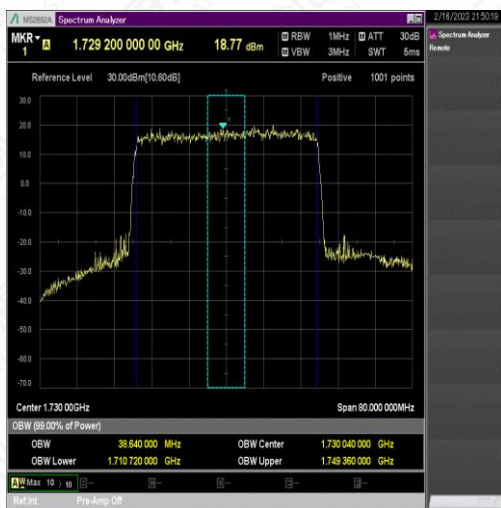
NTNV_N66_PC3_15_40_L_TID2_Ant1#1
