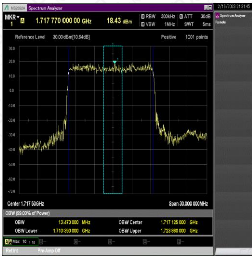
NTNV_N66_PC3_15_15_L_TID1_Ant1#1
