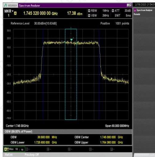
NTNV_N66_PC3_15_40_M_TID6_Ant1#1
