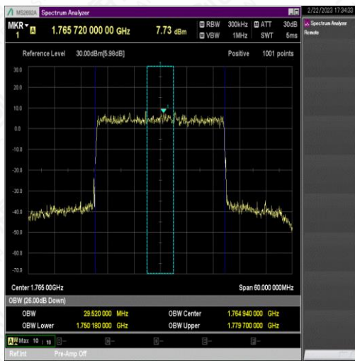
NTNV_N66_PC3_15_30_H_TID5_Ant1#1
