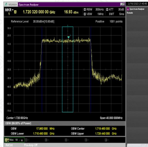
NTNV_N66_PC3_15_20_L_TID1_Ant1#1
