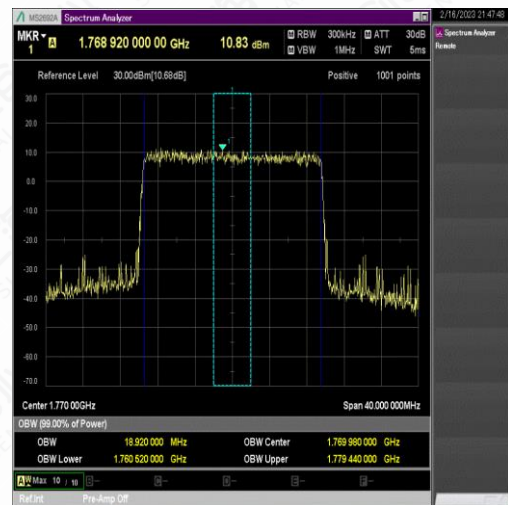
NTNV_N66_PC3_15_20_H_TID7_Ant1#1
