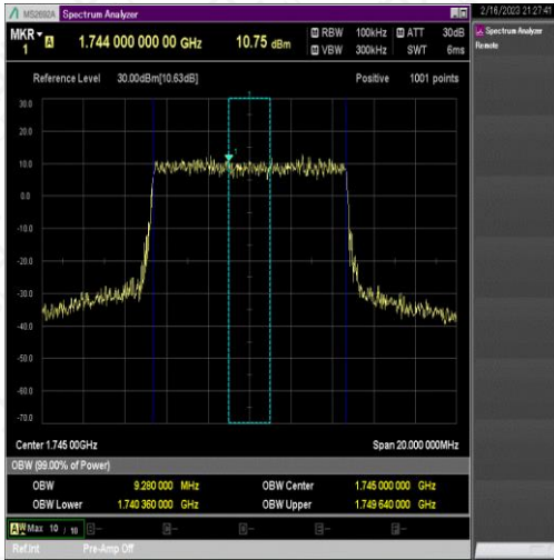
NTNV_N66_PC3_15_10_M_TID7_Ant1#1
