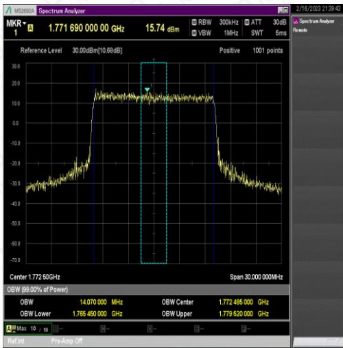
NTNV_N66_PC3_15_15_H_TID7_Ant1#1
