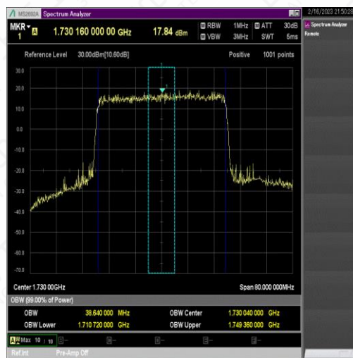
NTNV_N66_PC3_15_40_L_TID3_Ant1#1
