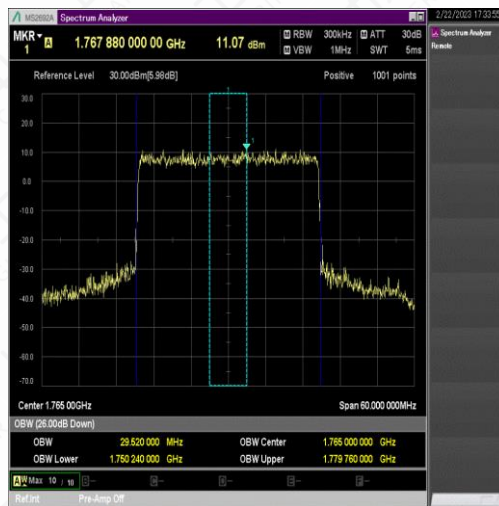
NTNV_N66_PC3_15_30_H_TID2_Ant1#1
