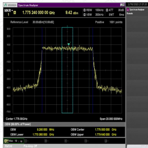
NTNV_N66_PC3_15_10_H_TID7_Ant1#1
