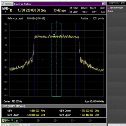
NTNV_N66_PC3_15_20_H_TID6_Ant1#1
