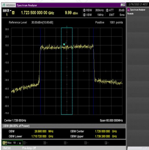
NTNV_N66_PC3_15_30_L_TID3_Ant1#1
