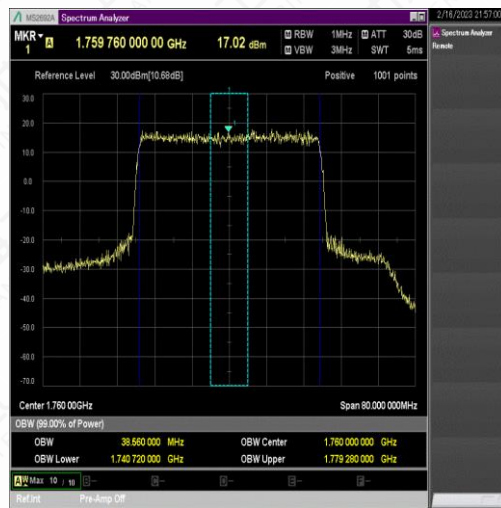
NTNV_N66_PC3_15_40_H_TID6_Ant#1
