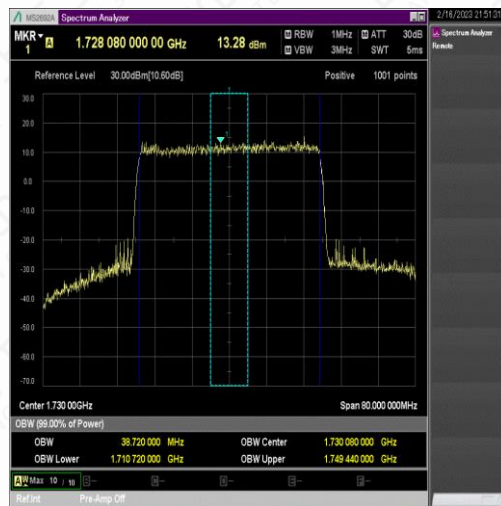
NTNV_N66_PC3_15_40_L_TID9_Ant1#1
