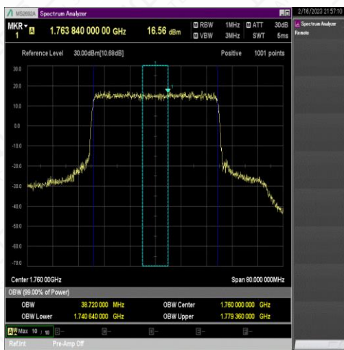
NTNV_N66_PC3_15_40_H_TID7_Ant#1
