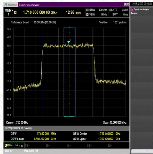
NTNV_N66_PC3_15_20_L_TID5_Ant1#1
