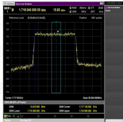
NTNV_N66_PC3_15_15_L_TID4_Ant1#1
