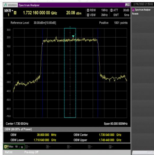
NTNV_N66_PC3_15_40_L_TID1_Ant1#1
