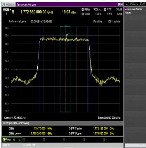
NTNV_N66_PC3_15_15_H_TID1_Ant1#1
