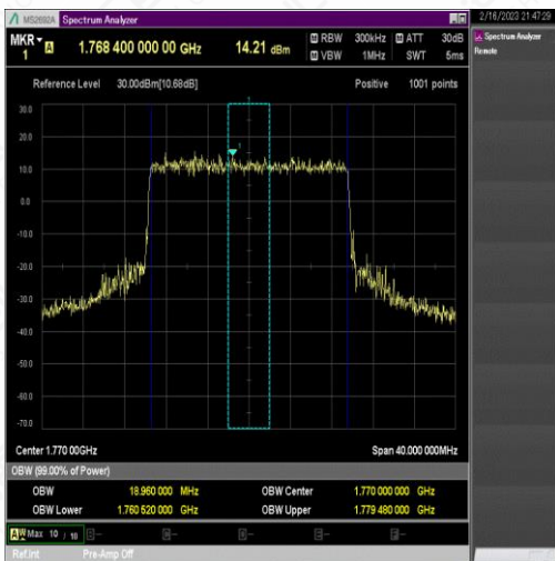
NTNV_N66_PC3_15_20_H_TID6_Ant1#1
