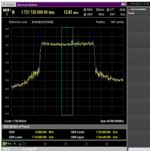
NTNV_N66_PC3_15_20_L_TID6_Ant1#1
