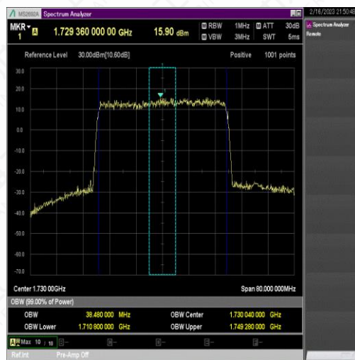
NTNV_N66_PC3_15_40_L_TID5_Ant1#1
