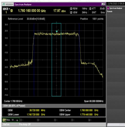
NTNV_N66_PC3_15_40_H_TID3_Ant#1
