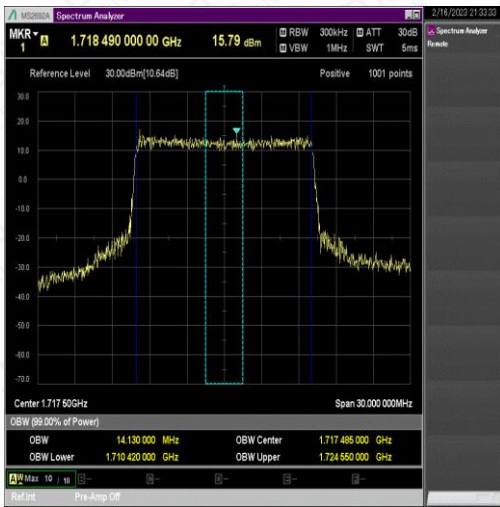
NTNV_N66_PC3_15_15_L_TID7_Ant1#1
