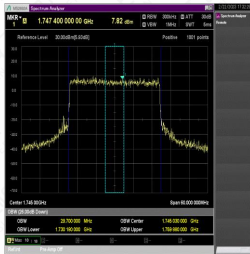
NTNV_N66_PC3_15_30_M_TID7_Ant1#1
