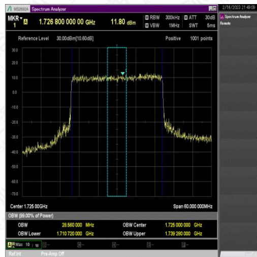
NTNV_N66_PC3_15_30_L_TID4_Ant1#1
