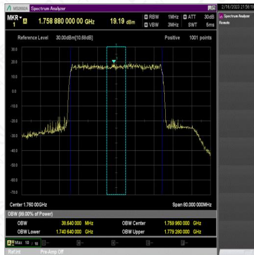
NTNV_N66_PC3_15_40_H_TID2_Ant1#1
