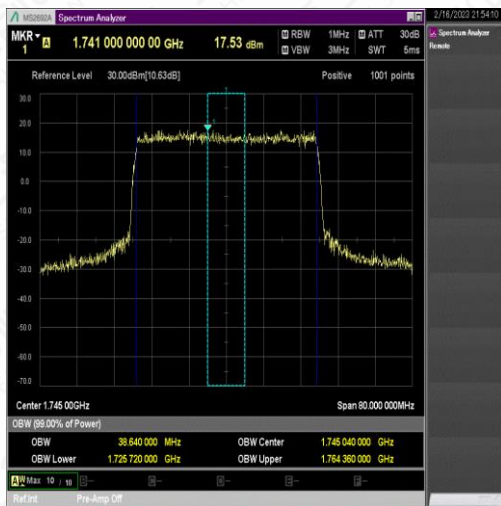
NTNV_N66_PC3_15_40_M_TID7_Ant1#1
