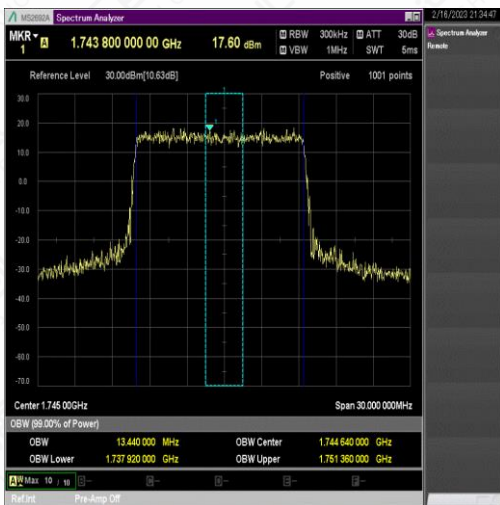
NTNV_N66_PC3_15_15_L_TID9_Ant1#1
