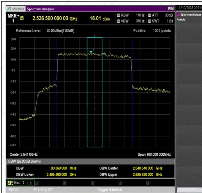
NTNV_N41_PC2_30_90_L_TID5_Ant1#1
