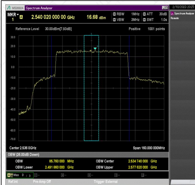
NTNV_N41_PC2_30_80_L_TID8_Ant1#1
