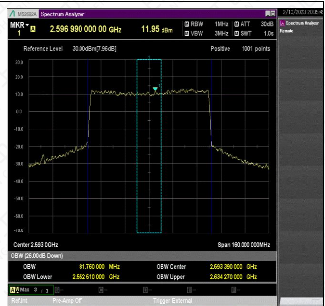
NTNV_N41_PC2_30_80_M_TID8_Ant1#1
