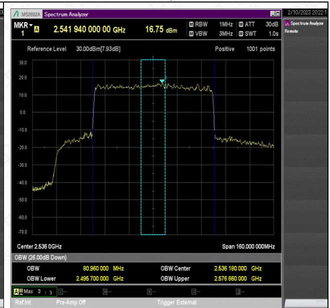
NTNV_N41_PC2_30_80_L_TID5_Ant1#1
