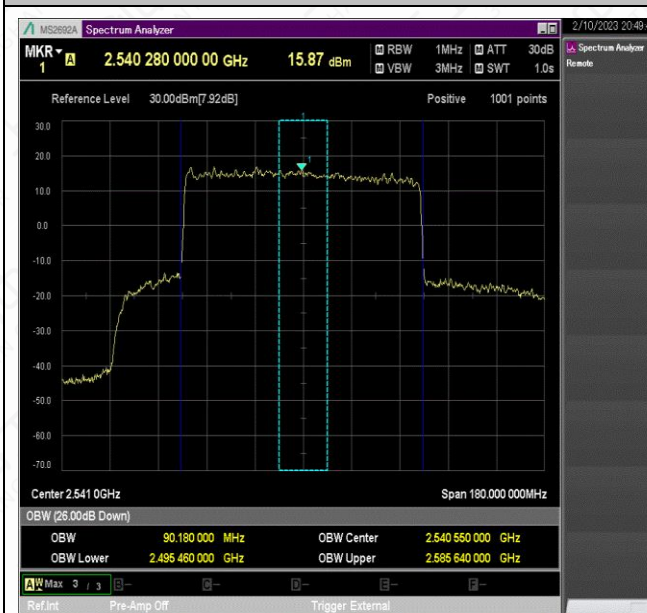
NTNV_N41_PC2_30_90_L_TID3_Ant1#1
