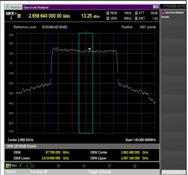
NTNV_N41_PC2_30_70_H_TID4_Ant1#1
