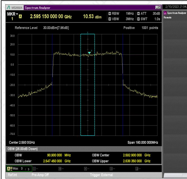
NTNV_N41_PC2_30_90_M_TID8_Ant1#1
