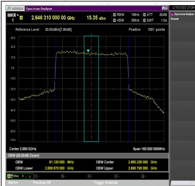
NTNV_N41_PC2_30_80_H_TID2_Ant1#1
