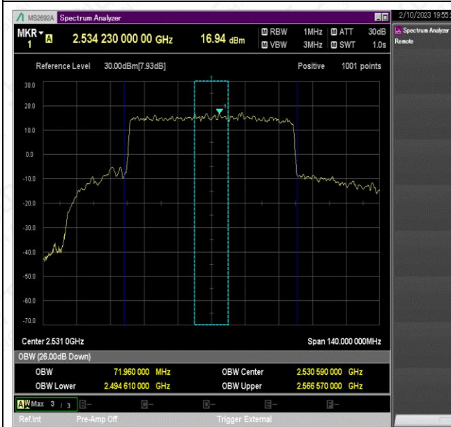
NTNV_N41_PC2_30_70_L_TID9_Ant1#1
