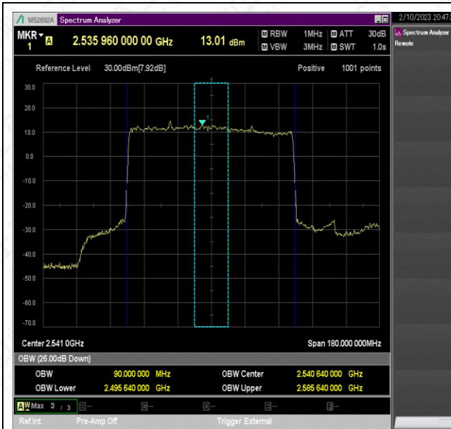
NTNV_N41_PC2_30_90_L_TID1_Ant1#1
