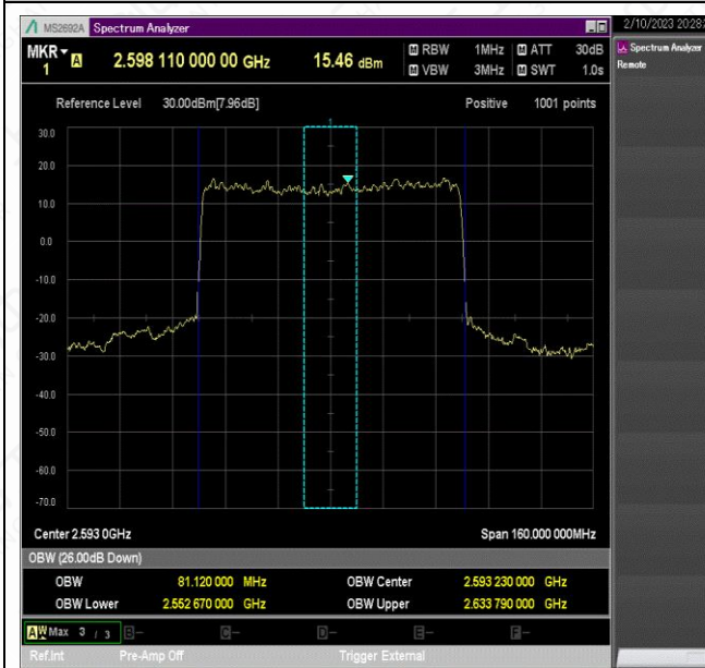
NTNV_N41_PC2_30_80_M_TID1_Ant1#1
