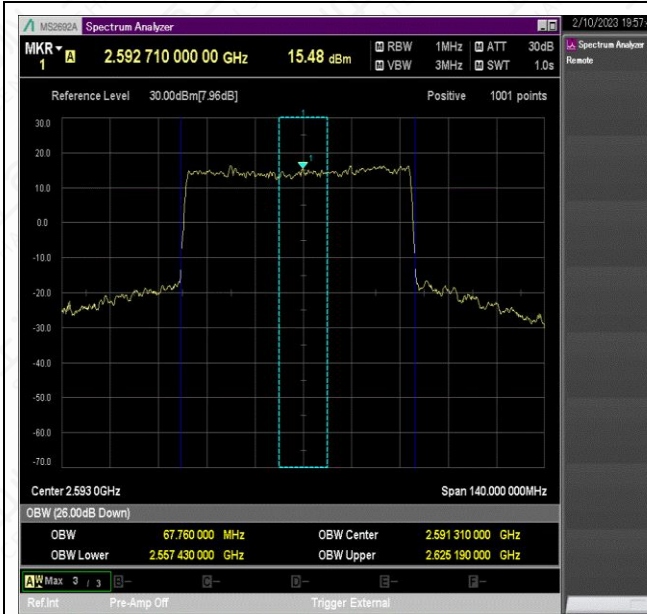
NTNV_N41_PC2_30_70_M_TID2_Ant1#1
