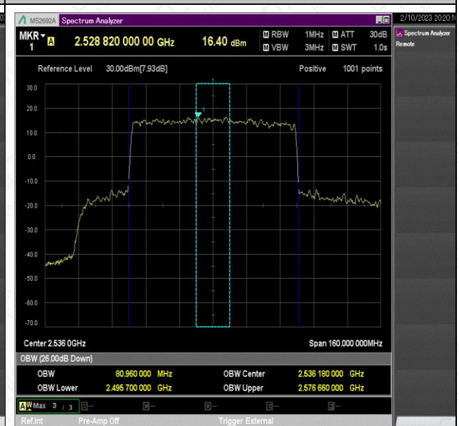
NTNV_N41_PC2_30_80_L_TID3_Ant1#1
