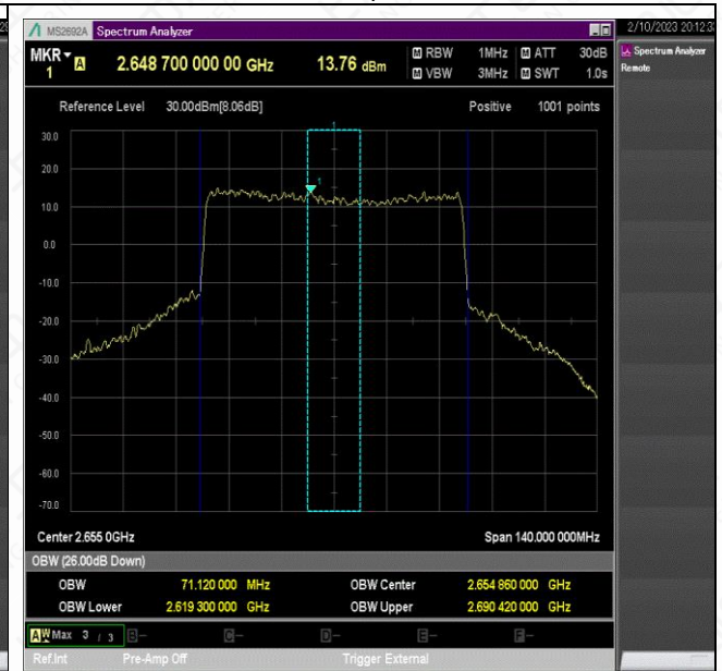
NTNV_N41_PC2_30_70_H_TID6_Ant1#1
