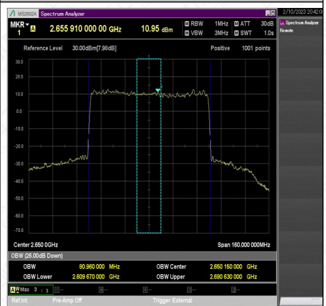
NTNV_N41_PC2_30_80_H_TID5_Ant1#1
