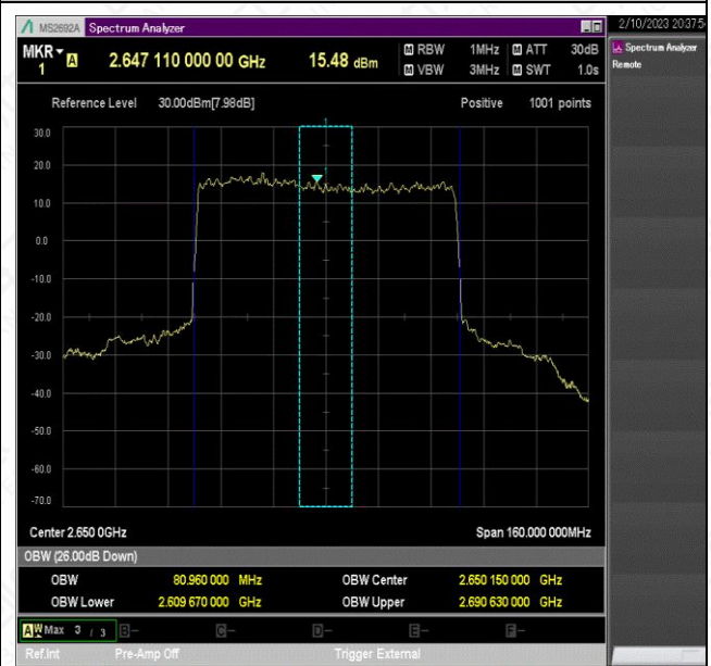
NTNV_N41_PC2_30_80_H_TID1_Ant1#1
