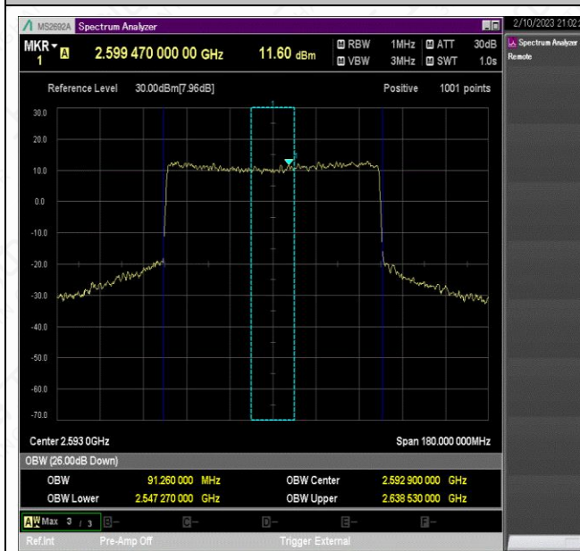
NTNV_N41_PC2_30_90_M_TID6_Ant1#1
