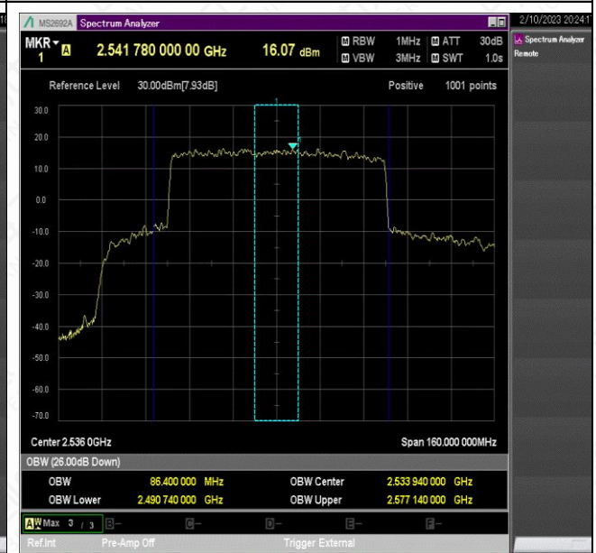
NTNV_N41_PC2_30_80_L_TID7_Ant1#1
