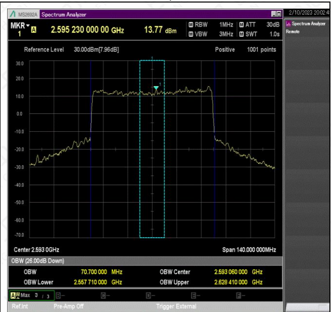
NTNV_N41_PC2_30_70_M_TID7_Ant1#1
