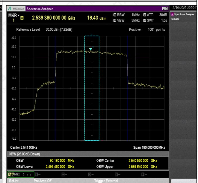
NTNV_N41_PC2_30_90_L_TID4_Ant1#1
