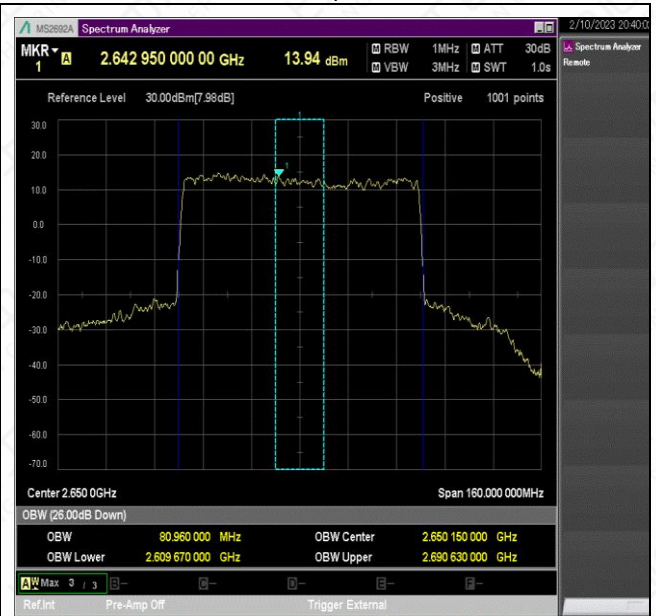
NTNV_N41_PC2_30_80_H_TID3_Ant1#1
