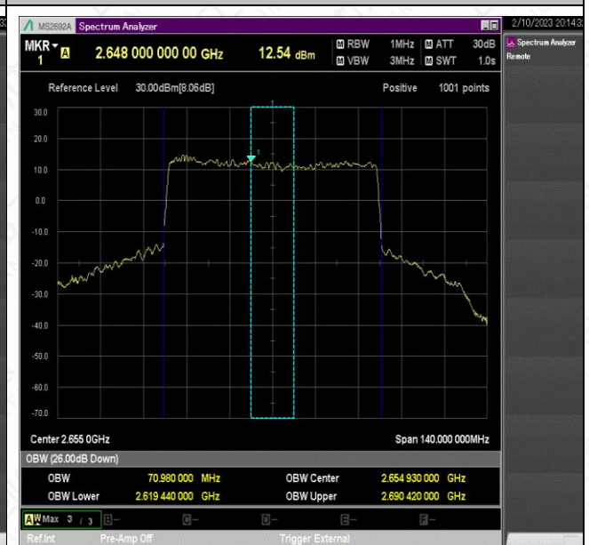
NTNV_N41_PC2_30_70_H_TID8_Ant1#1
