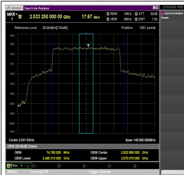
NTNV_N41_PC2_30_70_L_TID7_Ant1#1
