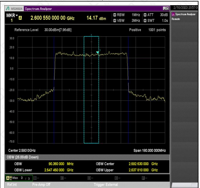
NTNV_N41_PC2_30_90_M_TID1_Ant1#1
