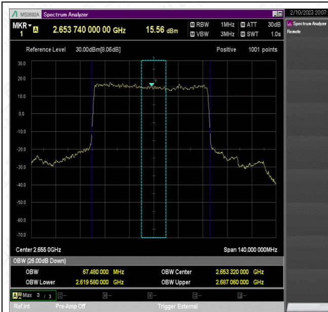
NTNV_N41_PC2_30_70_H_TID1_Ant1#1
