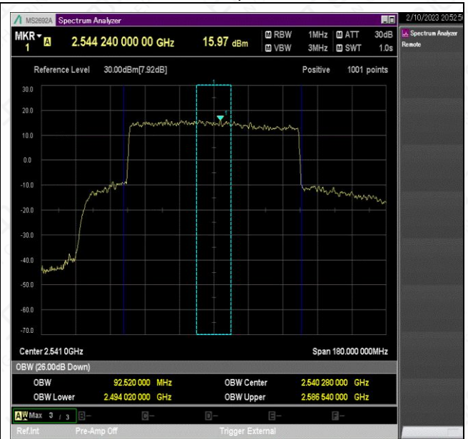
NTNV_N41_PC2_30_90_L_TID6_Ant1#1
