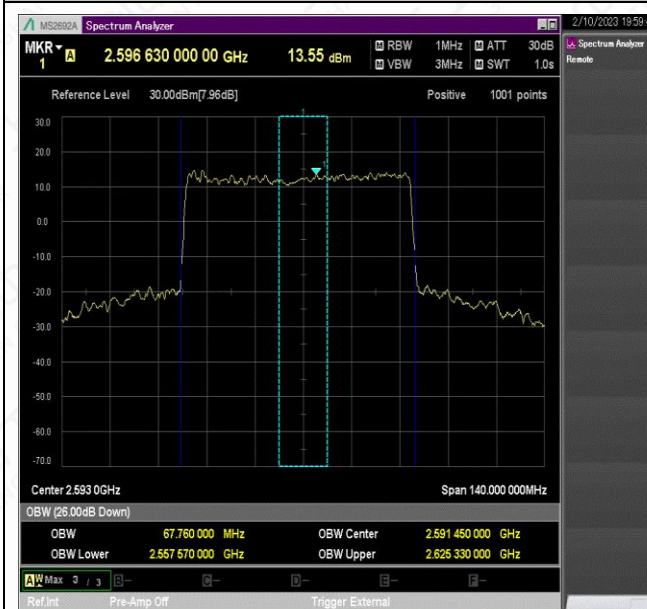
NTNV_N41_PC2_30_70_M_TID4_Ant1#1
