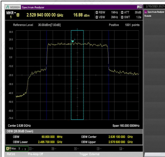
NTNV_N41_PC2_30_80_L_TID4_Ant1#1
