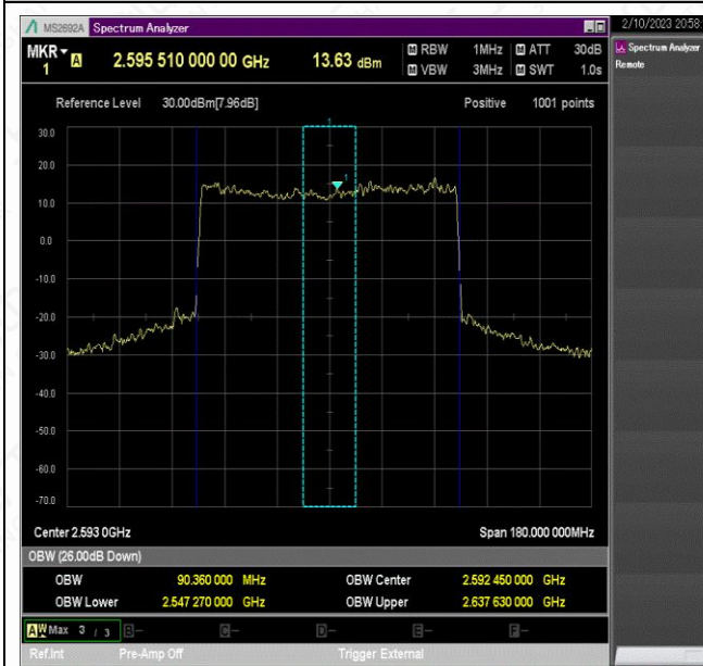
NTNV_N41_PC2_30_90_M_TID2_Ant1#1
