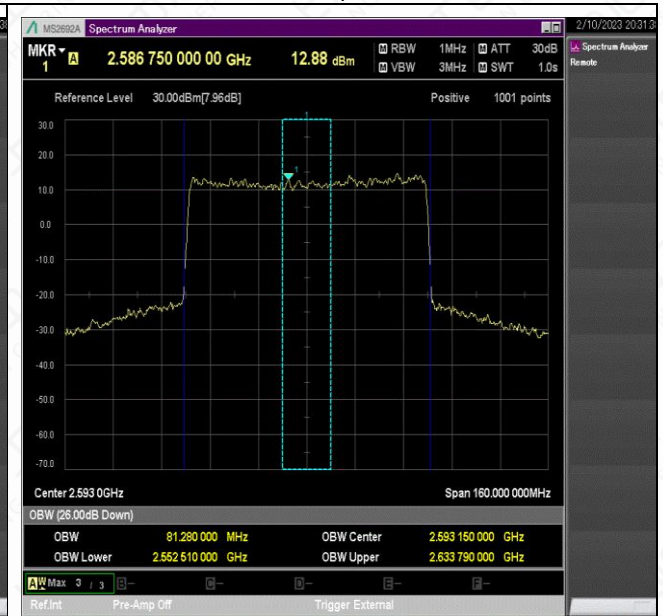
NTNV_N41_PC2_30_80_M_TID4_Ant1#1
