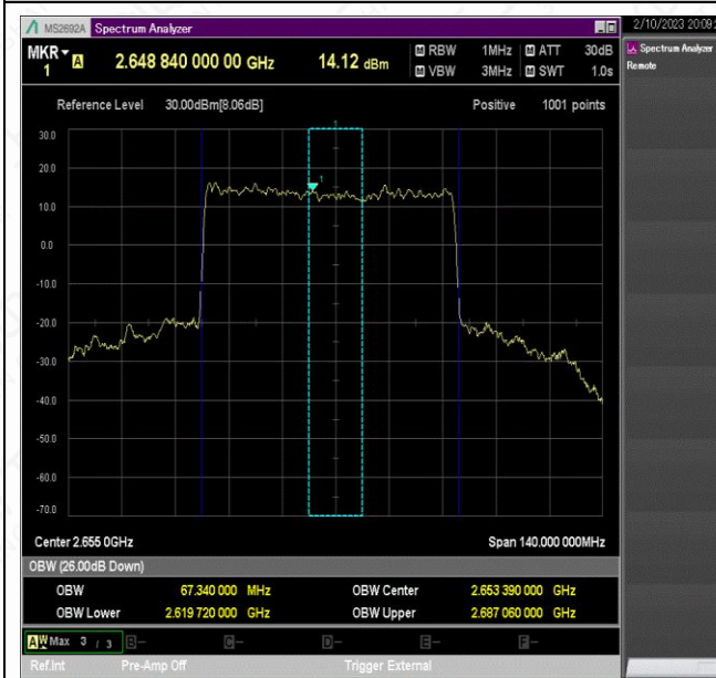
NTNV_N41_PC2_30_70_H_TID3_Ant1#1
