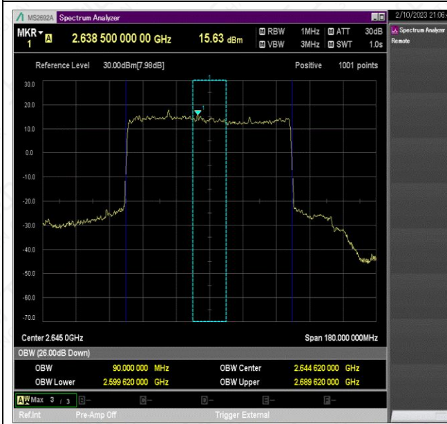
NTNV_N41_PC2_30_90_H_TID1_Ant1#1
