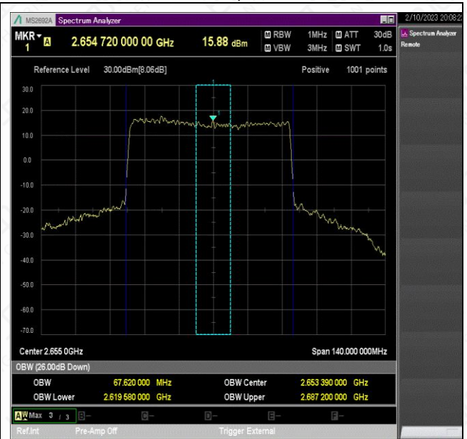
NTNV_N41_PC2_30_70_H_TID2_Ant1#1
