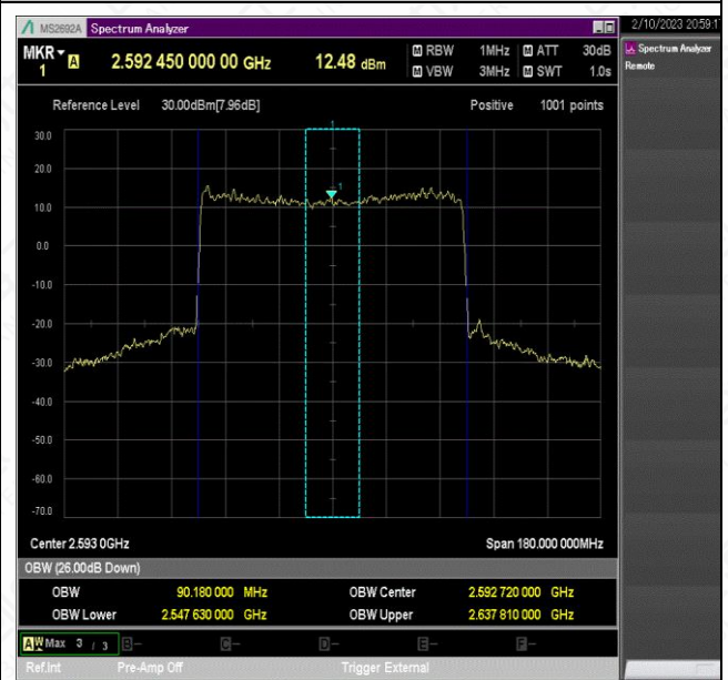
NTNV_N41_PC2_30_90_M_TID3_Ant1#1
