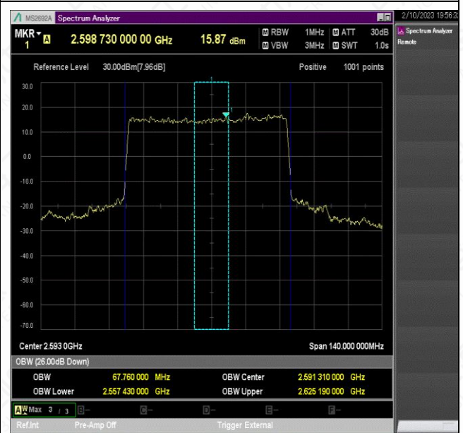
NTNV_N41_PC2_30_70_M_TID1_Ant1#1
