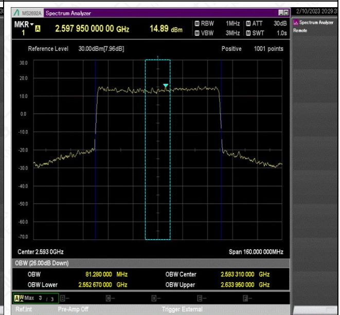
NTNV_N41_PC2_30_80_M_TID2_Ant1#1
