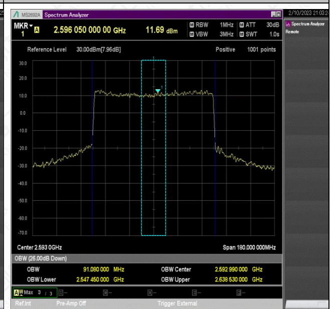
NTNV_N41_PC2_30_90_M_TID7_Ant1#1
