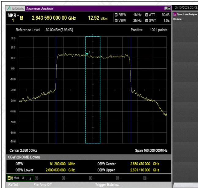
NTNV_N41_PC2_30_80_H_TID6_Ant1#1
