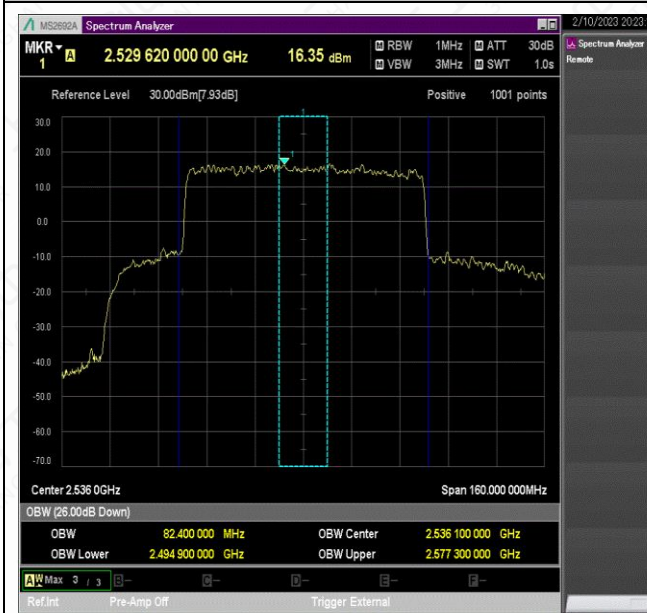
NTNV_N41_PC2_30_80_L_TID6_Ant1#1
