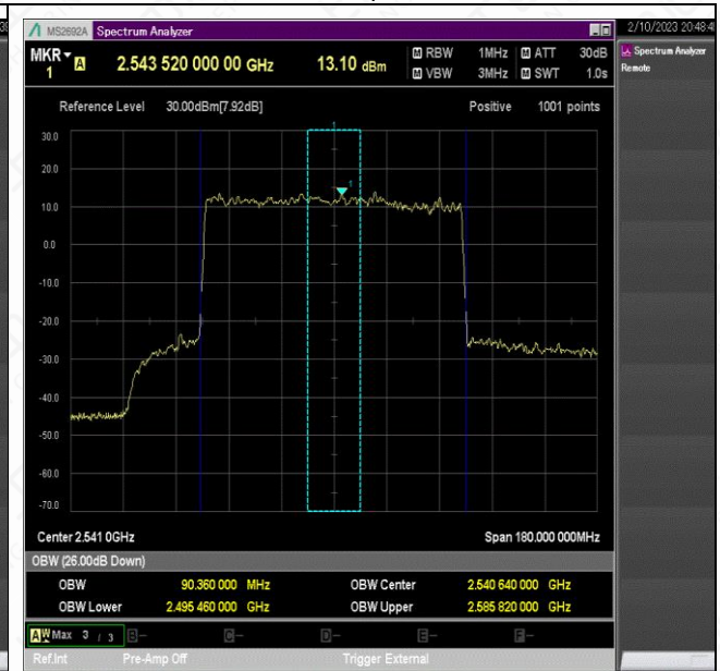
NTNV_N41_PC2_30_90_L_TID2_Ant1#1
