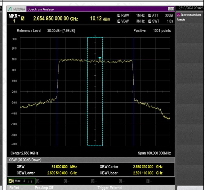
NTNV_N41_PC2_30_80_H_TID9_Ant1#1
