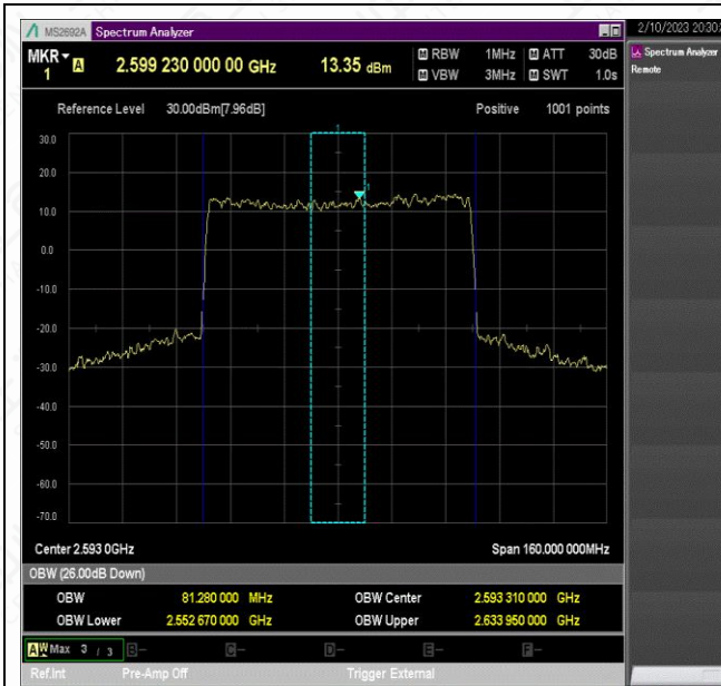
NTNV_N41_PC2_30_80_M_TID3_Ant1#1
