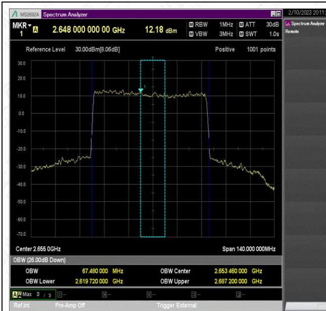
NTNV_N41_PC2_30_70_H_TID5_Ant1#1
