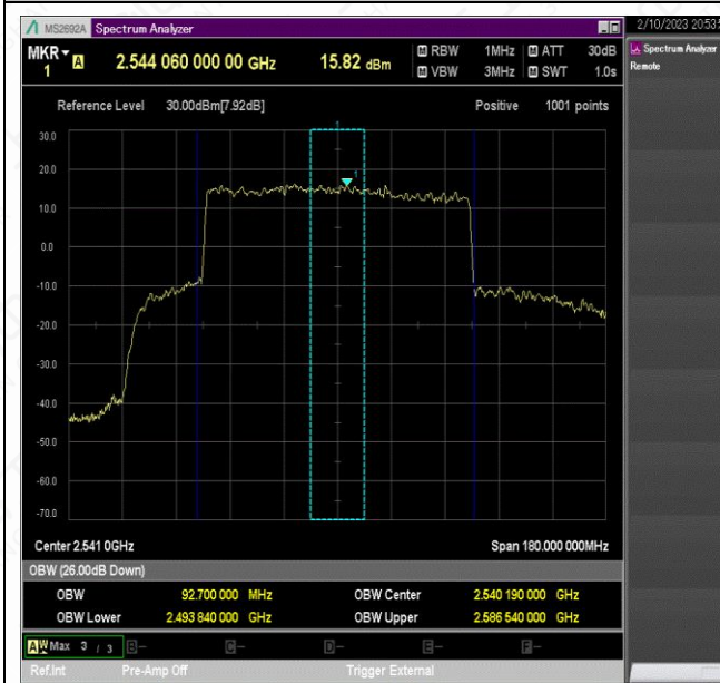
NTNV_N41_PC2_30_90_L_TID7_Ant1#1
