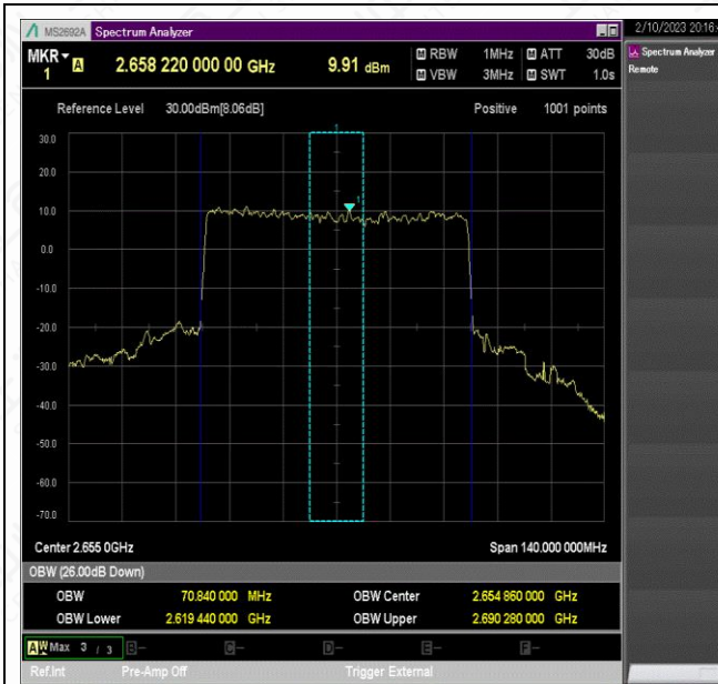
NTNV_N41_PC2_30_70_H_TID9_Ant1#1
