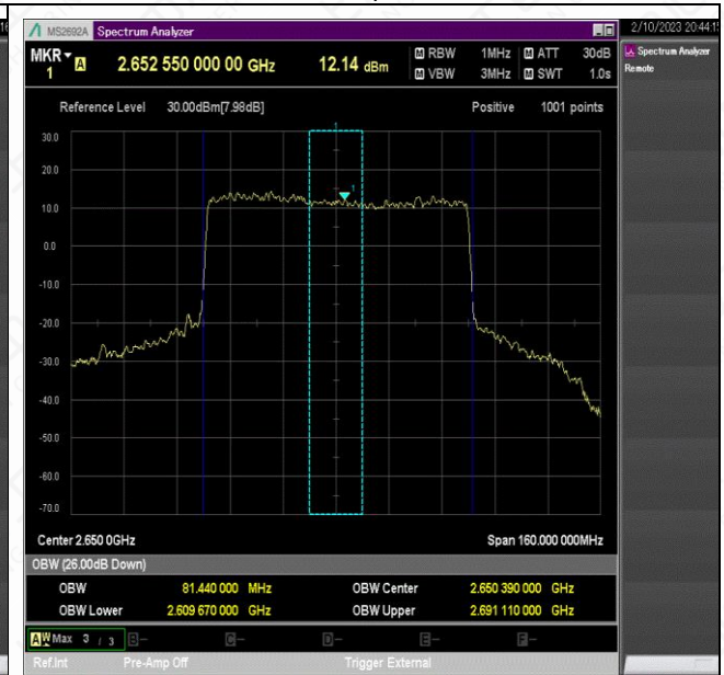
NTNV_N41_PC2_30_80_H_TID7_Ant1#1
