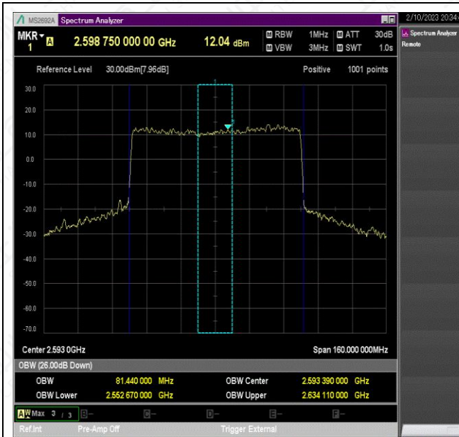
NTNV_N41_PC2_30_80_M_TID7_Ant1#1
