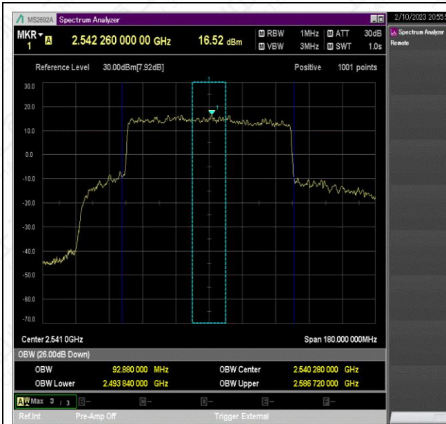
NTNV_N41_PC2_30_90_L_TID9_Ant1#1
