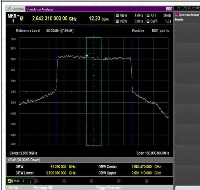
NTNV_N41_PC2_30_80_H_TID8_Ant1#1
