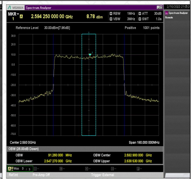
NTNV_N41_PC2_30_90_M_TID9_Ant1#1
