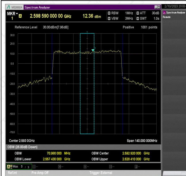
NTNV_N41_PC2_30_70_M_TID8_Ant1#1
