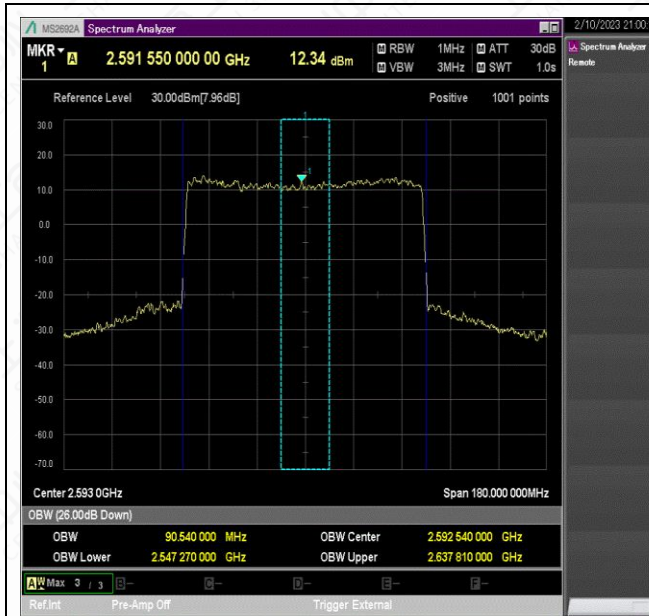
NTNV_N41_PC2_30_90_M_TID4_Ant1#1
