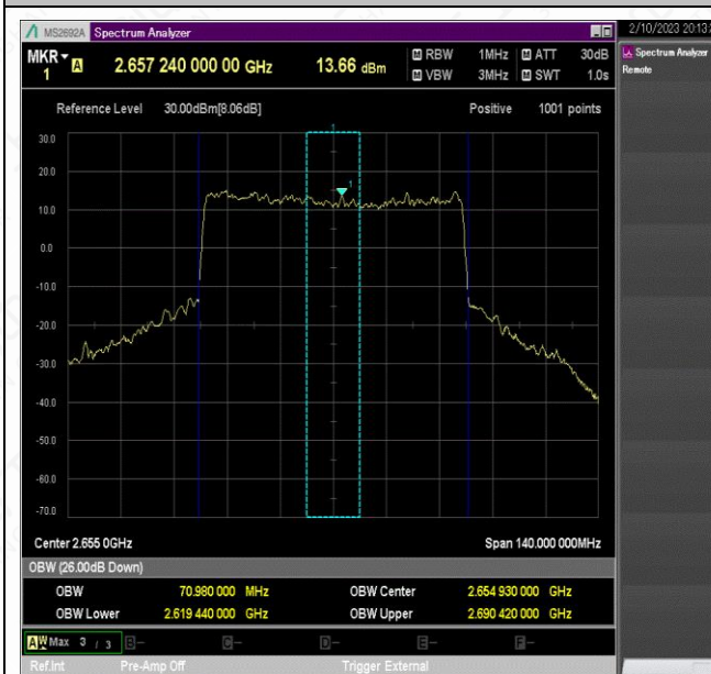
NTNV_N41_PC2_30_70_H_TID7_Ant1#1
