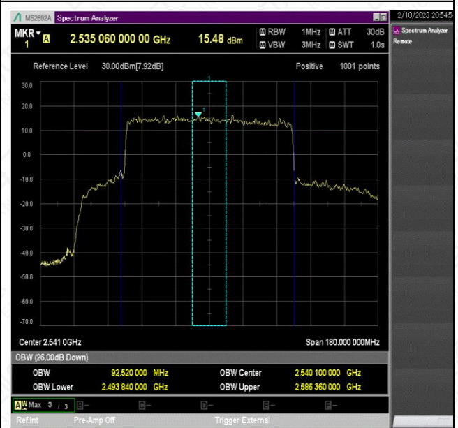
NTNV_N41_PC2_30_90_L_TID8_Ant1#1
