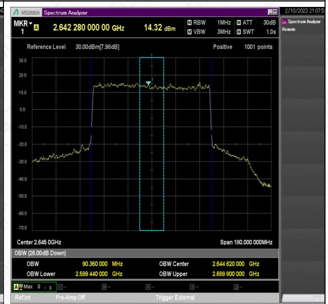
NTNV_N41_PC2_30_90_H_TID2_Ant1#1
