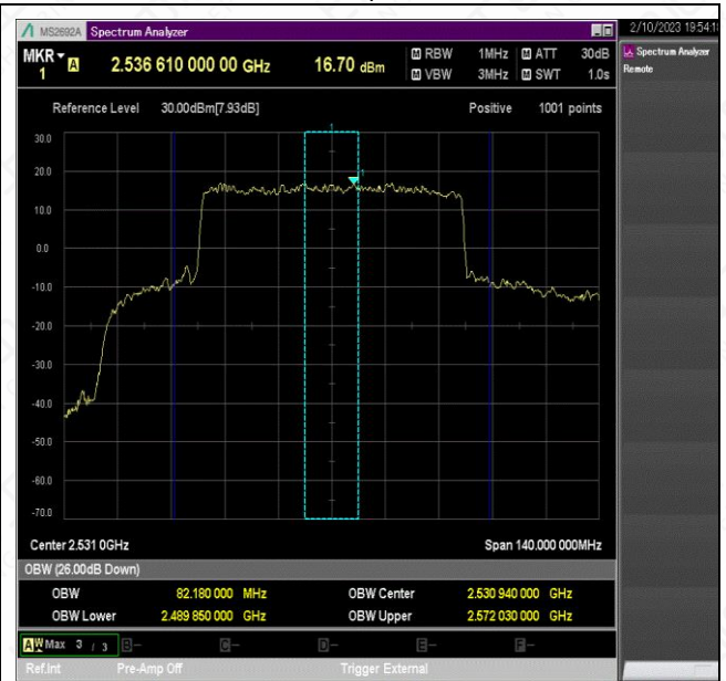
NTNV_N41_PC2_30_70_L_TID8_Ant1#1
