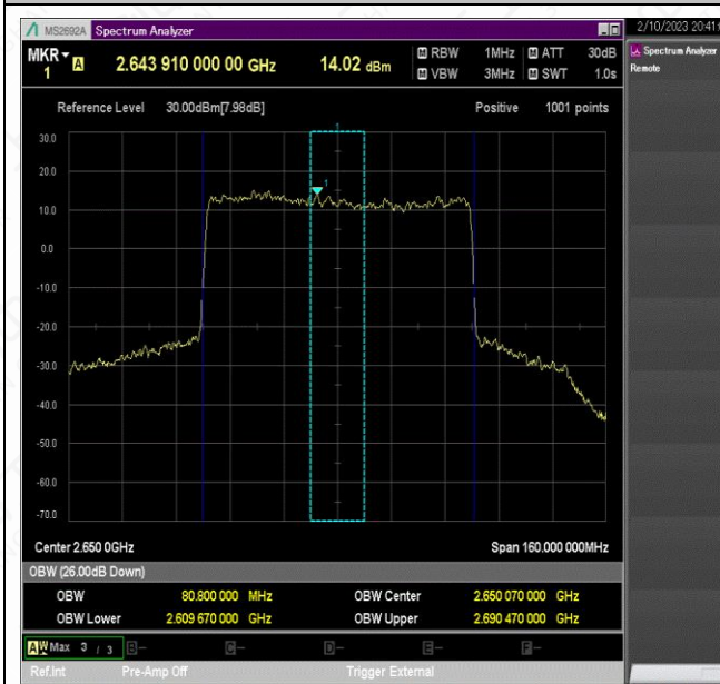
NTNV_N41_PC2_30_80_H_TID4_Ant1#1
