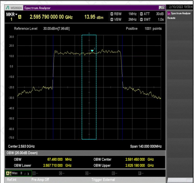
NTNV_N41_PC2_30_70_M_TID3_Ant1#1
