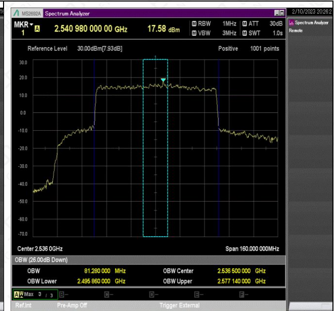
NTNV_N41_PC2_30_80_L_TID9_Ant1#1
