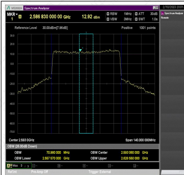
NTNV_N41_PC2_30_70_M_TID6_Ant1#1
