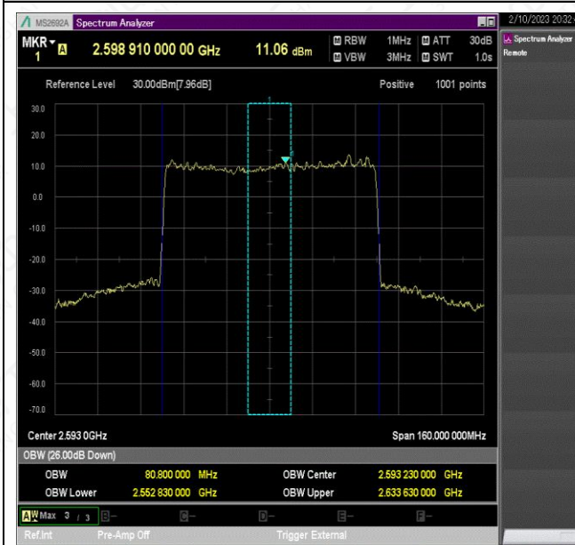
NTNV_N41_PC2_30_80_M_TID5_Ant1#1
