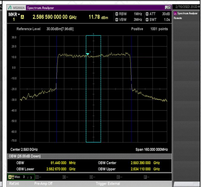
NTNV_N41_PC2_30_80_M_TID6_Ant1#1
