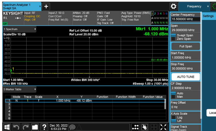
20M_5M_Q16_FULLRB_CSE1
