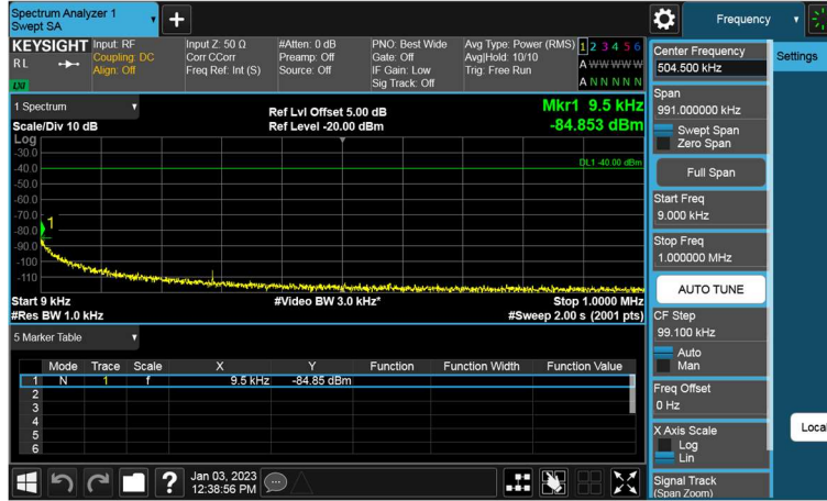
20M_5M_Q16_FULLRB_CSE0b
