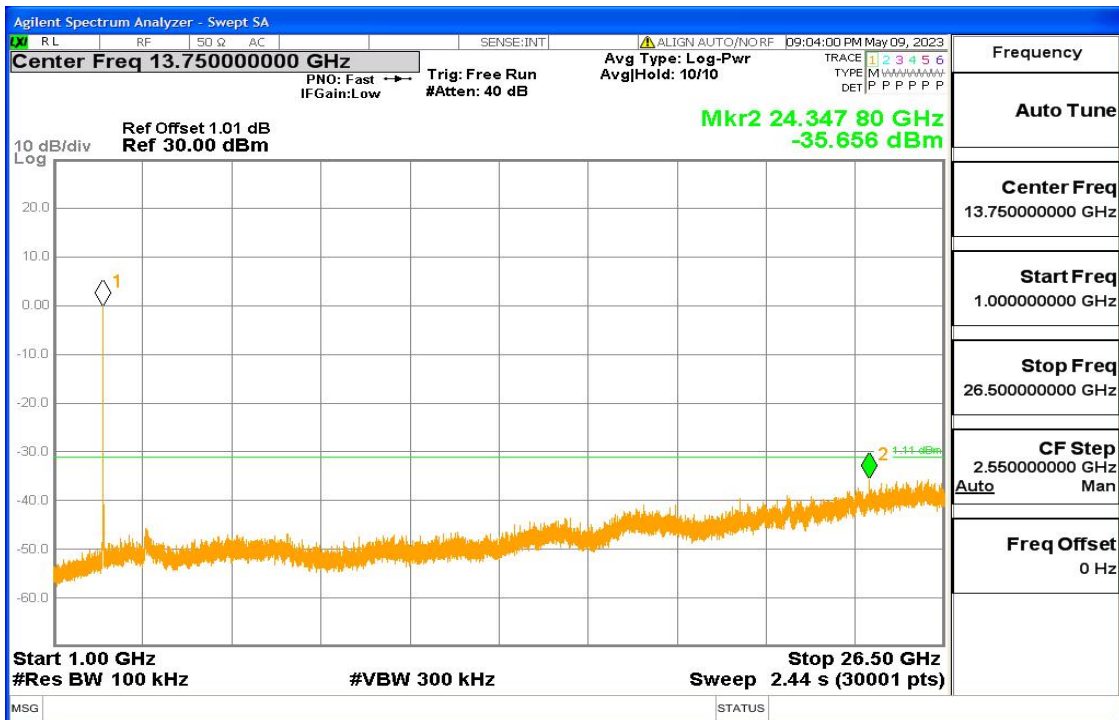
11g Fig3
