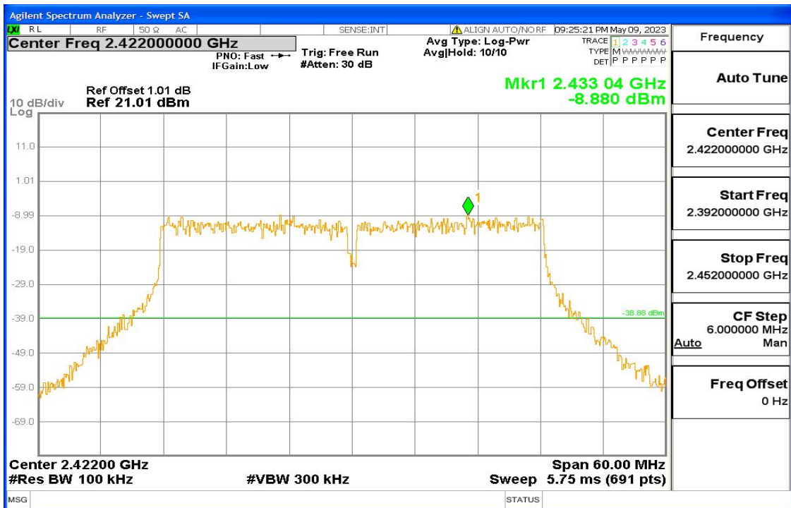
11n-HT40 Fig1
