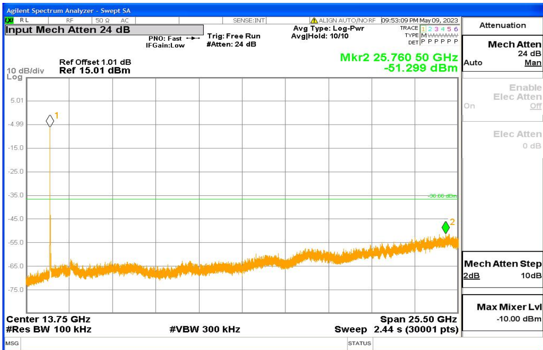
11n-HT20 Fig3
