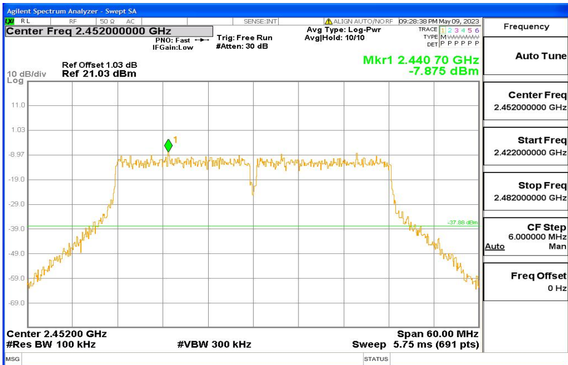
11n-HT40 Fig7
