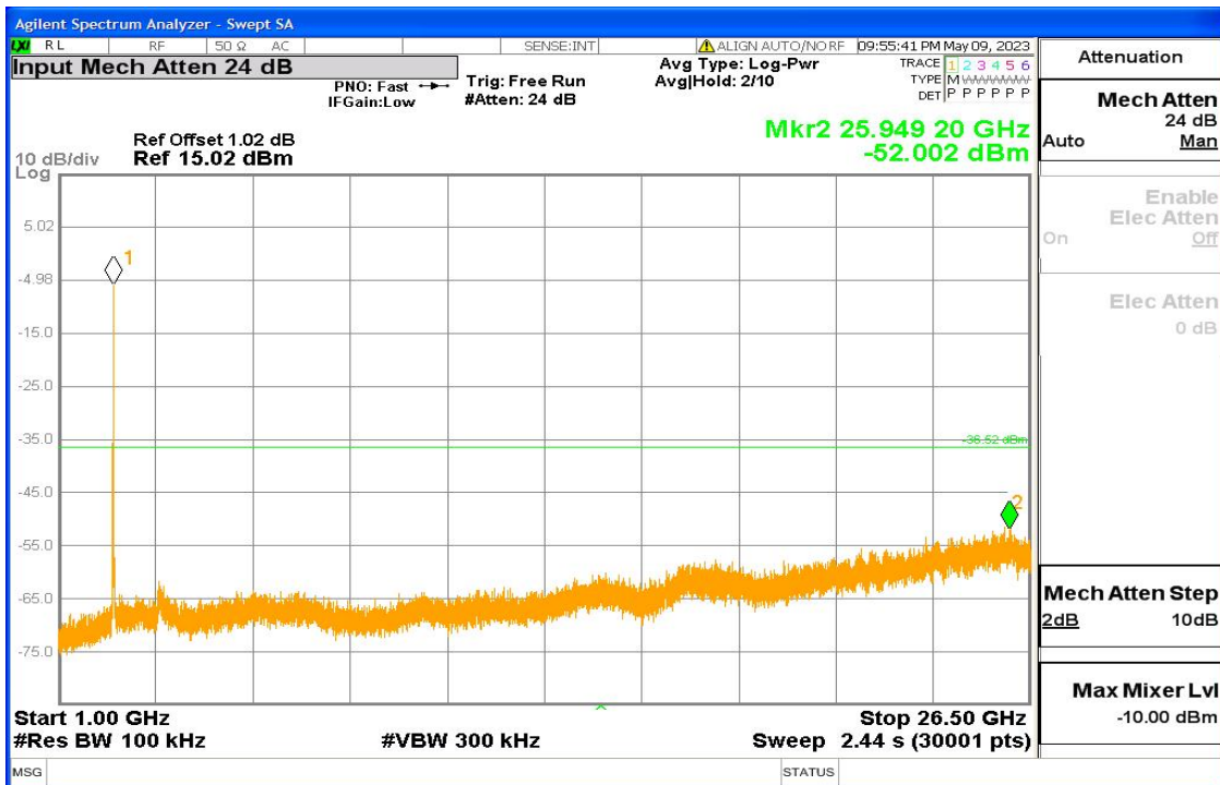
11n-HT20 Fig6
