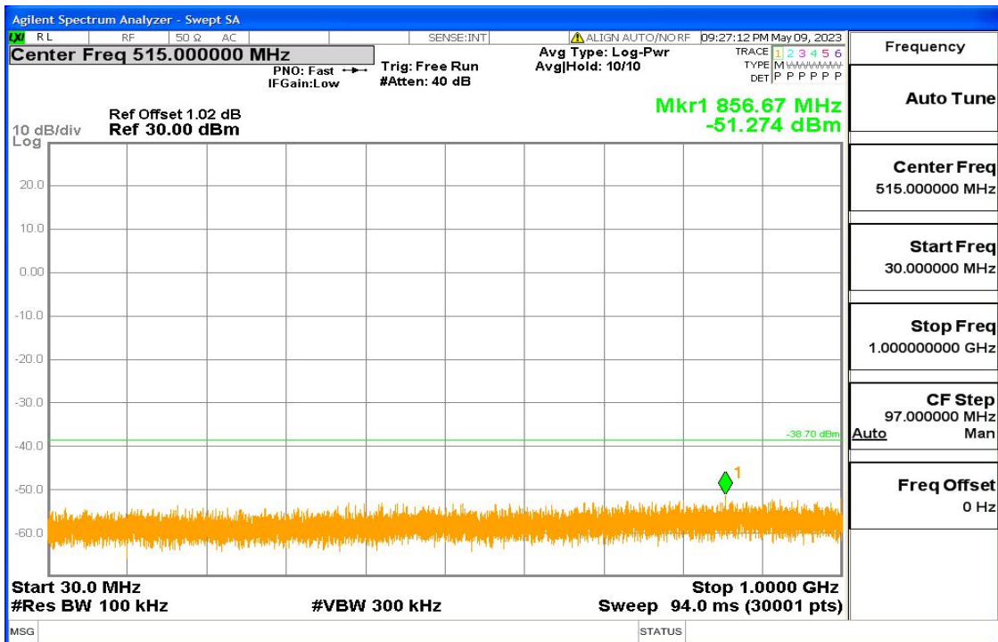
11n-HT40 Fig5
