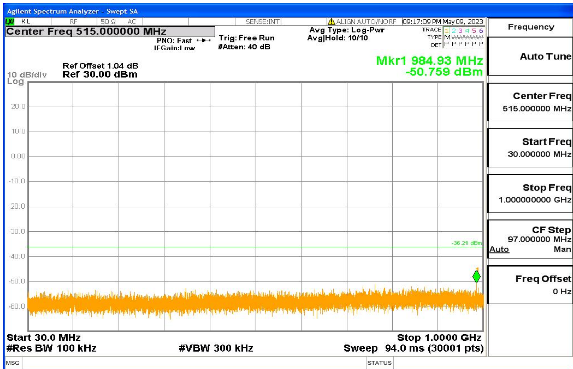
11n-HT20 Fig8
