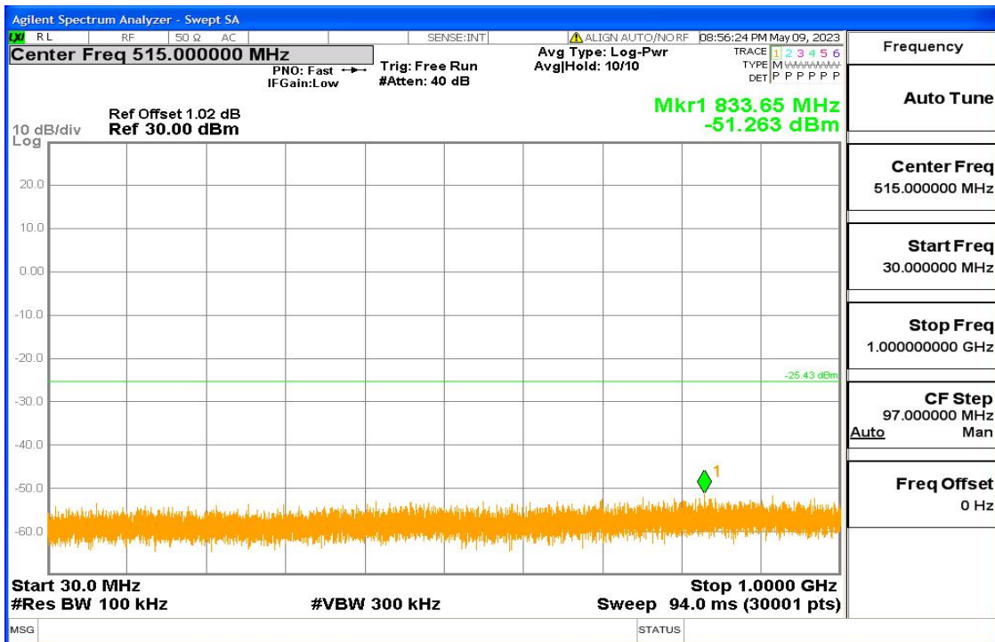
11b Fig5
