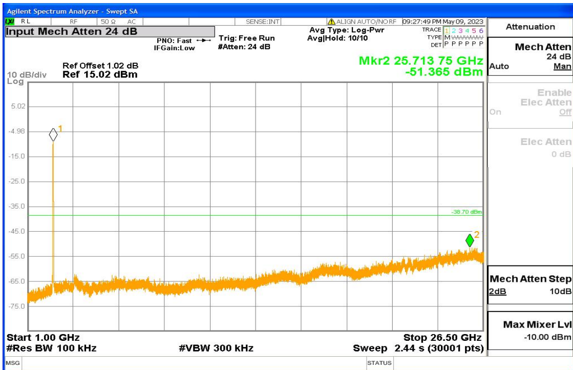
11n-HT40 Fig6
