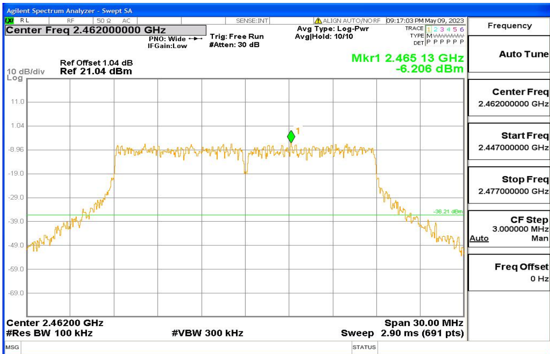
11n-HT20 Fig7
