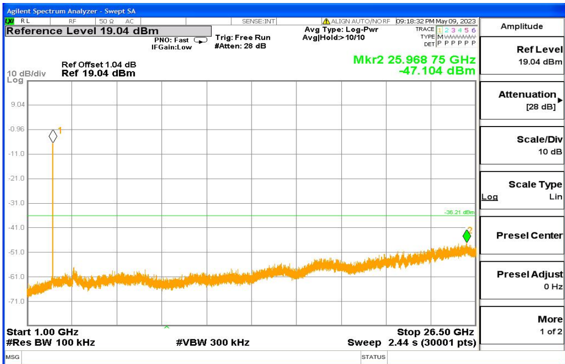
11n-HT20 Fig9
