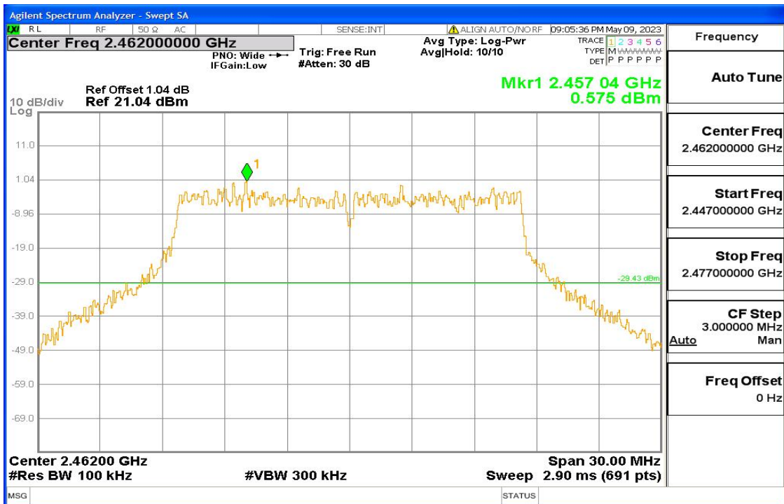
11g Fig7
