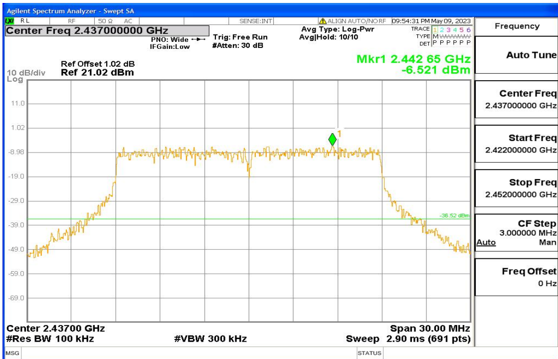
11n-HT20 Fig4
