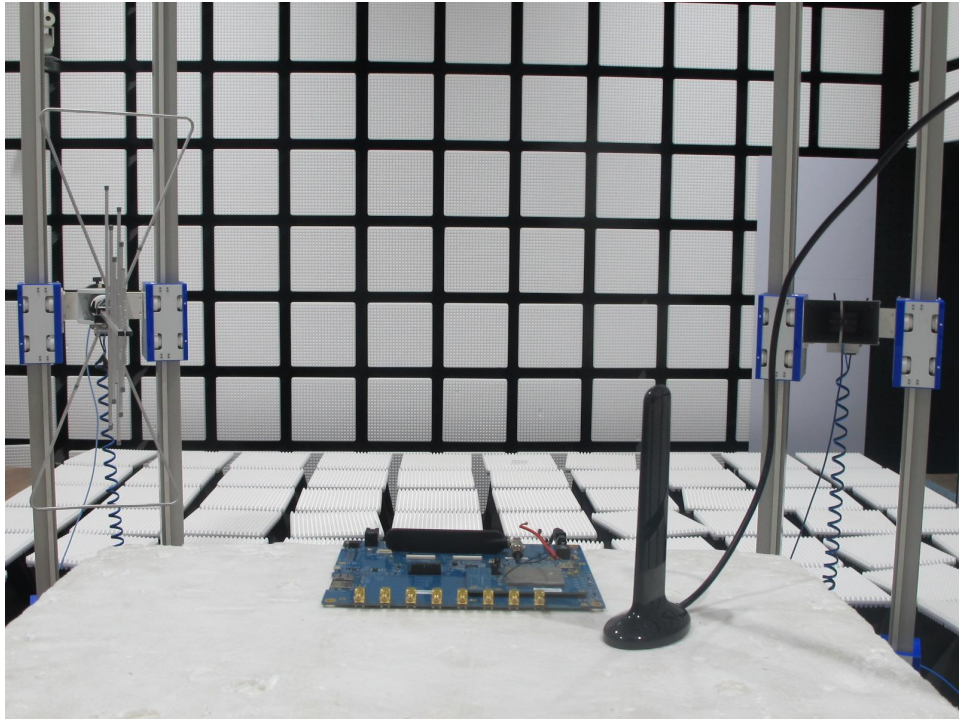
RSE_30MHz-18GHz
