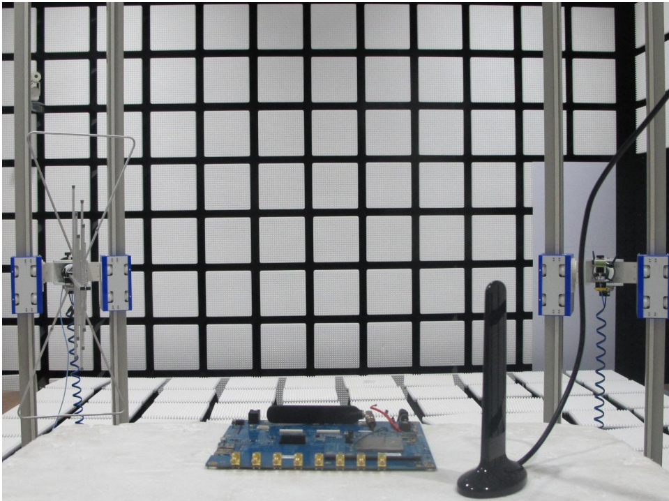
RSE_18GHz-20GHz
