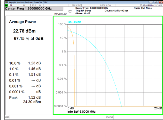
Band25-20M-QPSK-1 RB-M
