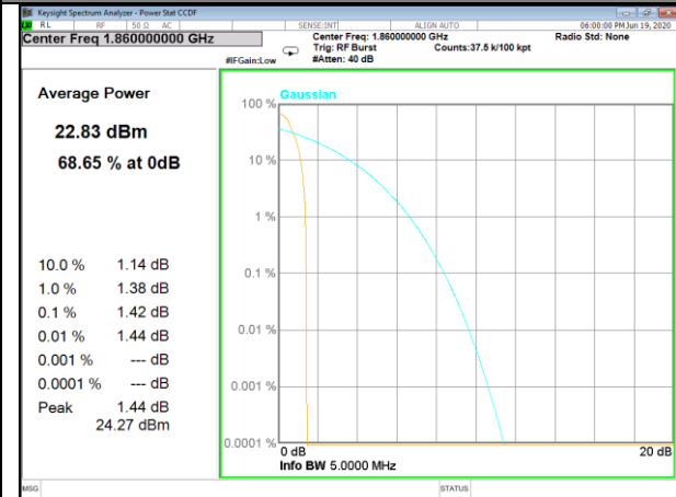
Band2-20M-QPSK-1 RB-M
