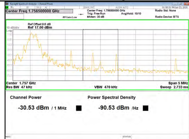
Band4 16QAM_3M_Higher_1-RB
