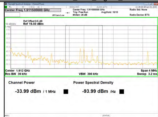
Band2 16QAM_15M_Higher_1-RB
