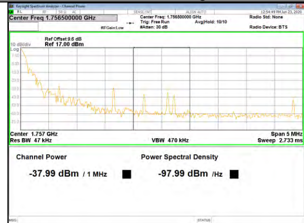
Band4 16QAM_15M_Higher_1-RB
