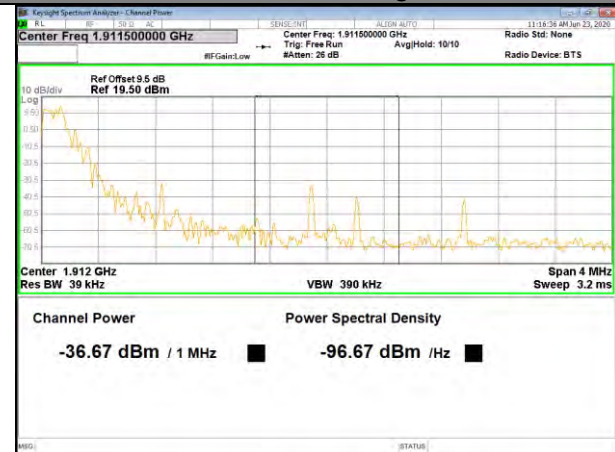
Band2 16QAM_3M_Higher_1-RB
