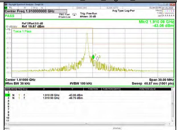
Band2 16QAM_15M_Higher_1-RB
