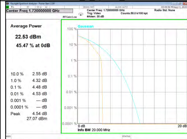
Band4_1_Q16_Low
