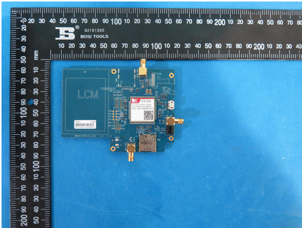
A7672SA
