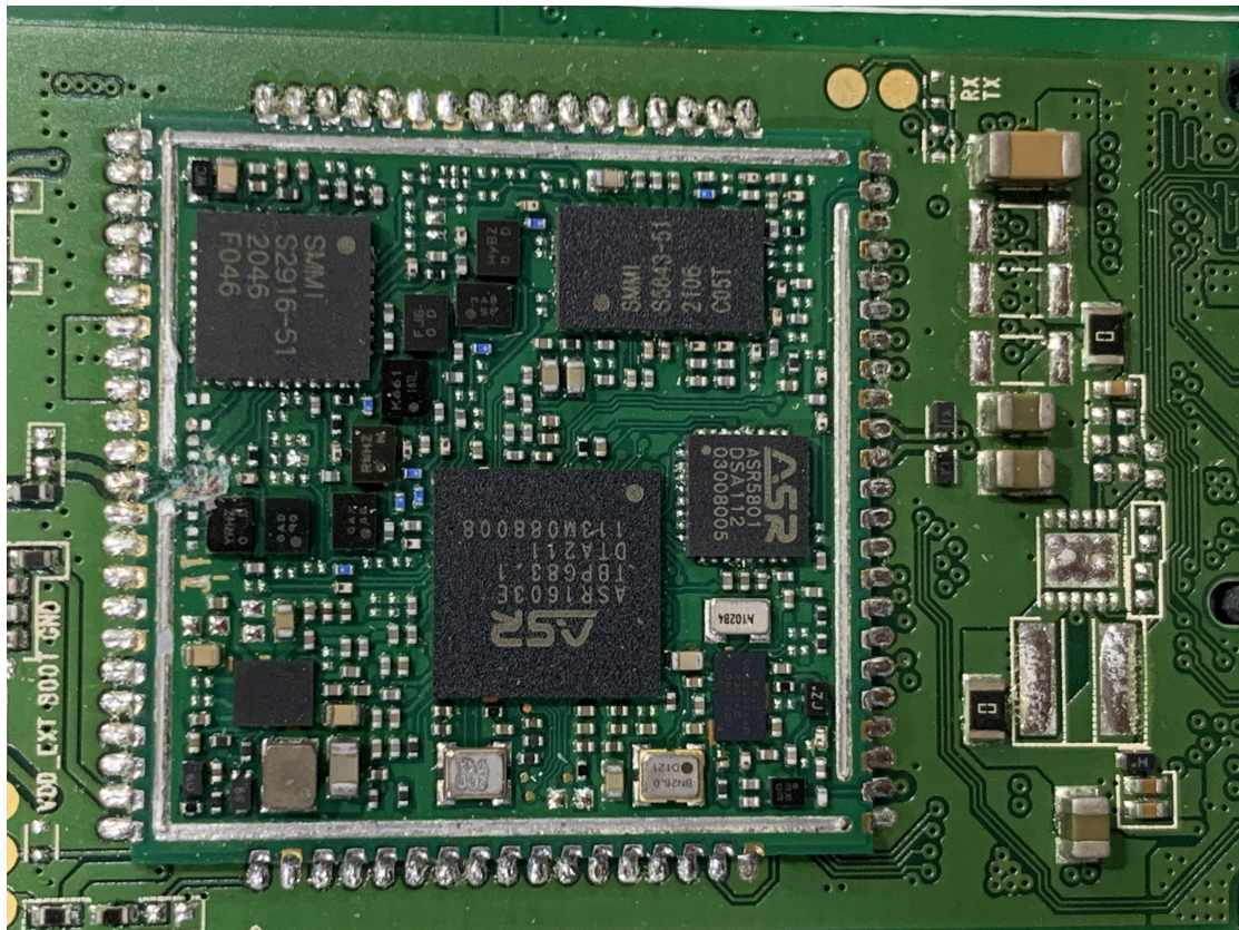
A7672SAminiPCIE
