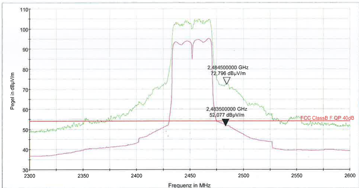
S770_2_4_40_CH11_Bandedge PK+ CLRWR [S770_2_4_40_CH11_Bandedge.Result:1] S770_2_4_40_CH11_Bandedge AVG CLRWR [S770_2_4_40_CH11_Bandedge.Result:2] FCC ClassB F QP 40dB [..EMI radiated!] PK+ CLRWR [Ergebnistabelle.Result:1] AVG CLRWR [Ergebnistabelle.Result:2]
