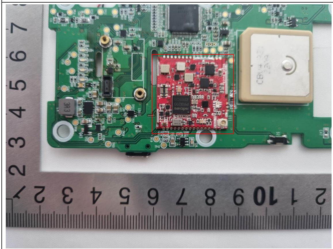
RFID Module
