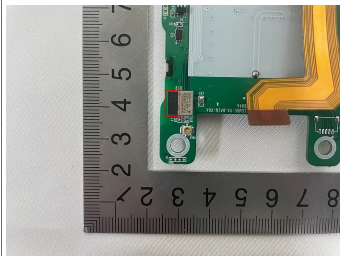
BLE Antenna
