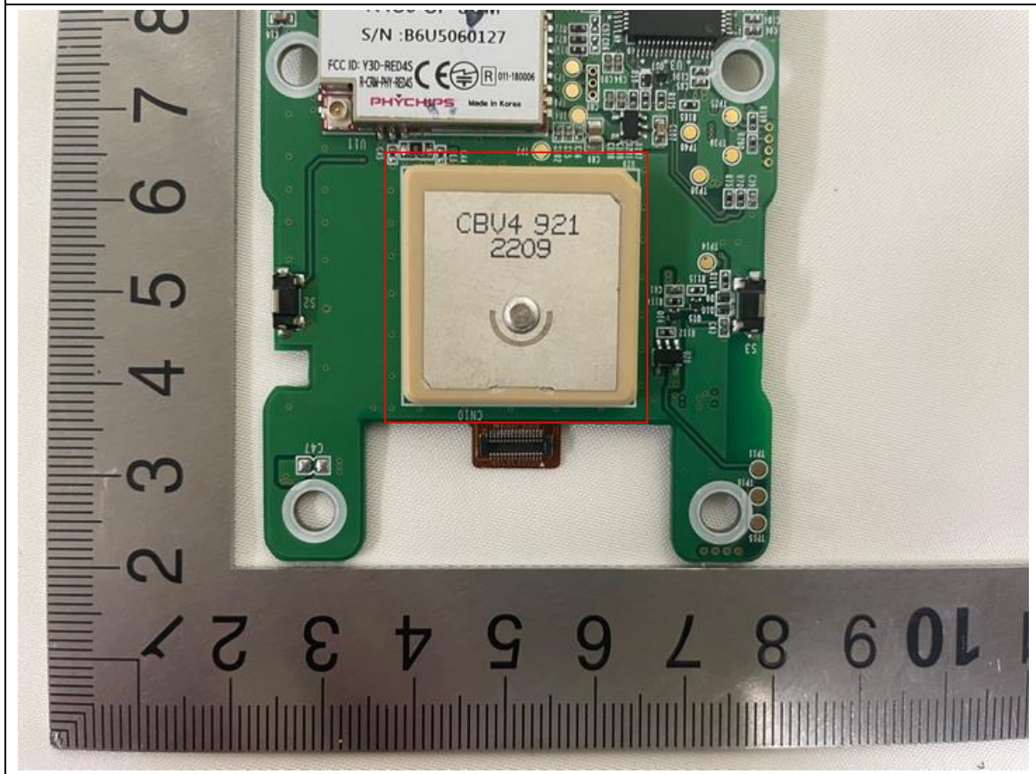
RFID Antenna
