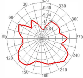
2500.000MHz E1
