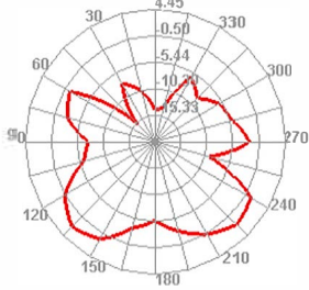
2450.000MHz E1
