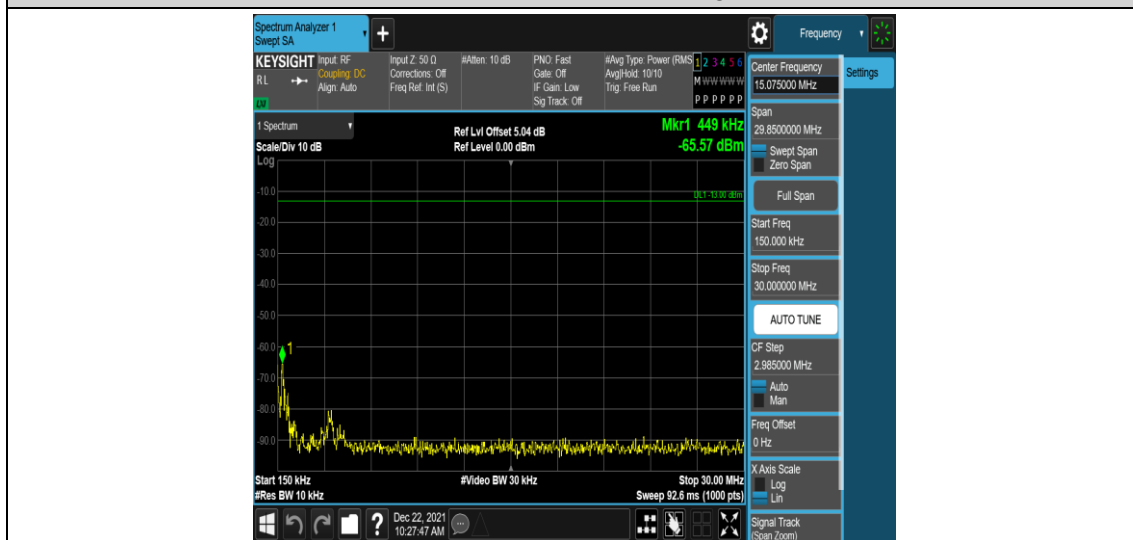
Band71-5MHz-16QAM-133447-1RB#0-Range2:0.15~30MHz
