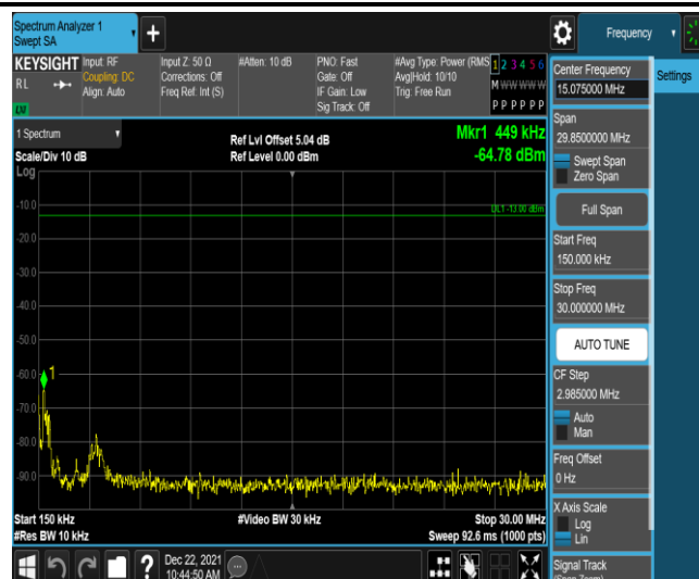
Band71-10MHz-QPSK-133172-1RB#0-Range2:0.15~30MHz
