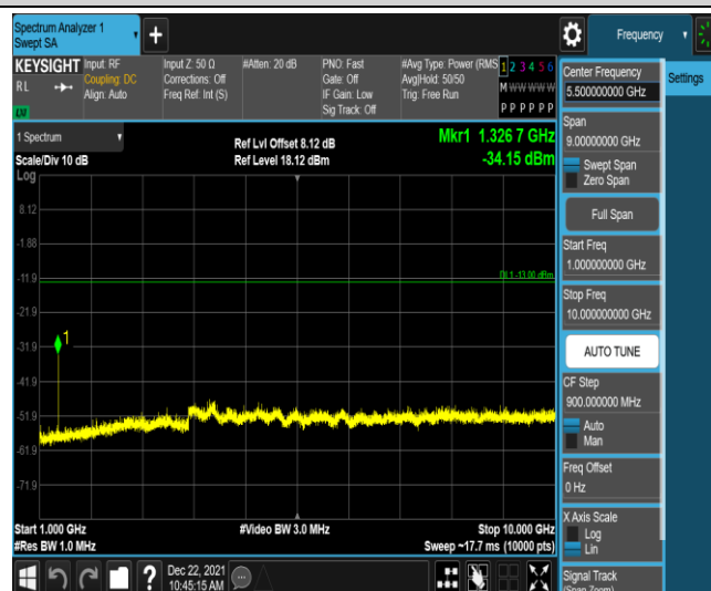
Band71-10MHz-QPSK-133172-1RB#0-Range4:1000~10000MHz
