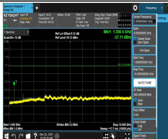
Band71-5MHz-QPSK-133297-1RB#0-Range4:1000~10000MHz
