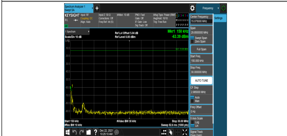
Band71-5MHz-QPSK-133297-1RB#0-Range2:0.15~30MHz
