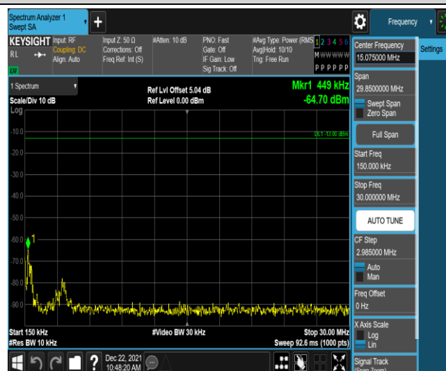
Band71-10MHz-QPSK-133422-1RB#0-Range2:0.15~30MHz
