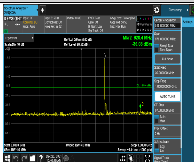
Band71-10MHz-QPSK-133297-1RB#0-Range3:30~1000MHz
