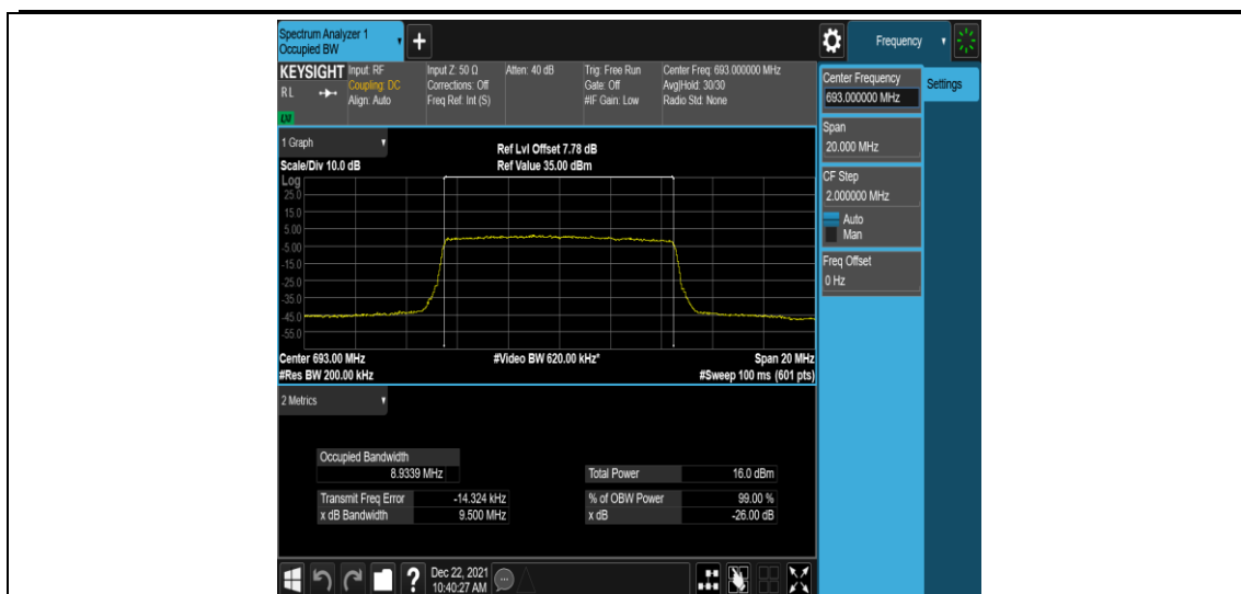
Band71-10MHz-QPSK-133422-50RB#0
