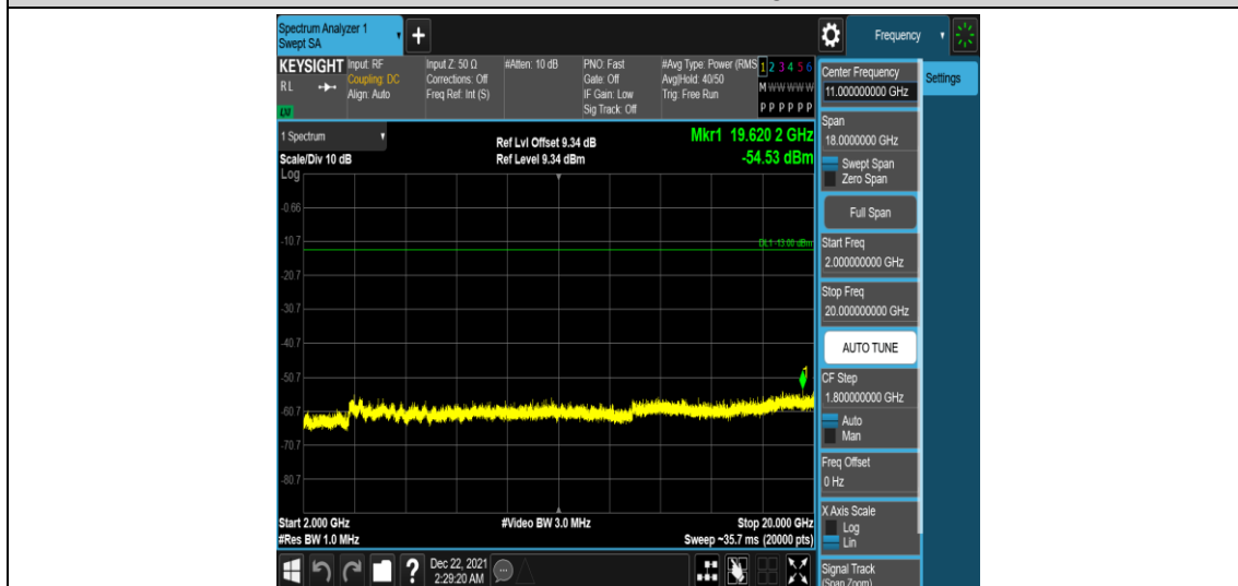
Band25-20MHz-QPSK-26590-1RB#0-Range5:2000~20000MHz
