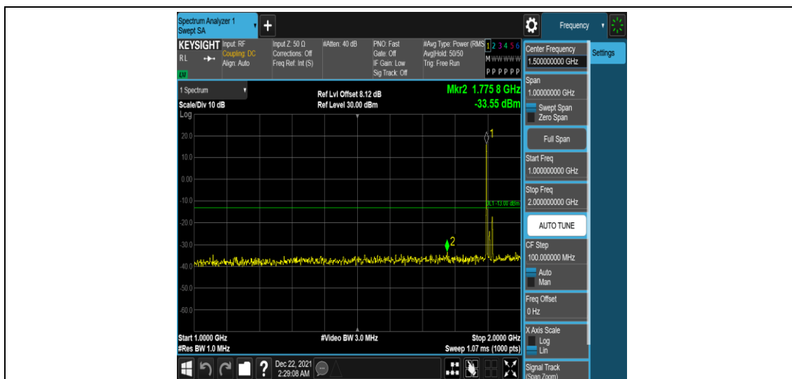
Band25-20MHz-QPSK-26590-1RB#0-Range4:1000~2000MHz
