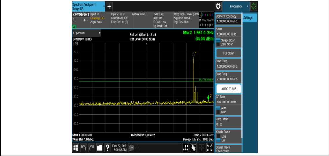
Band25-15MHz-QPSK-26115-1RB#0-Range4:1000~2000MHz
