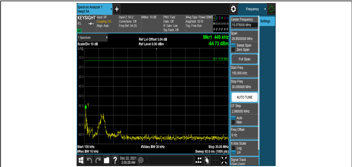
Band25-15MHz-QPSK-26115-1RB#0-Range2:0.15~30MHz
