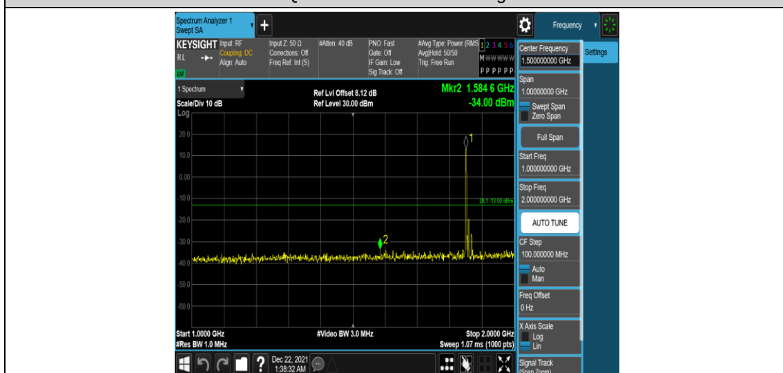
Band25-10MHz-QPSK-26090-1RB#0-Range4:1000~2000MHz
