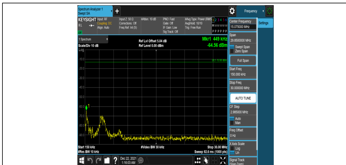
Band25-5MHz-QPSK-26065-1RB#0-Range2:0.15~30MHz
