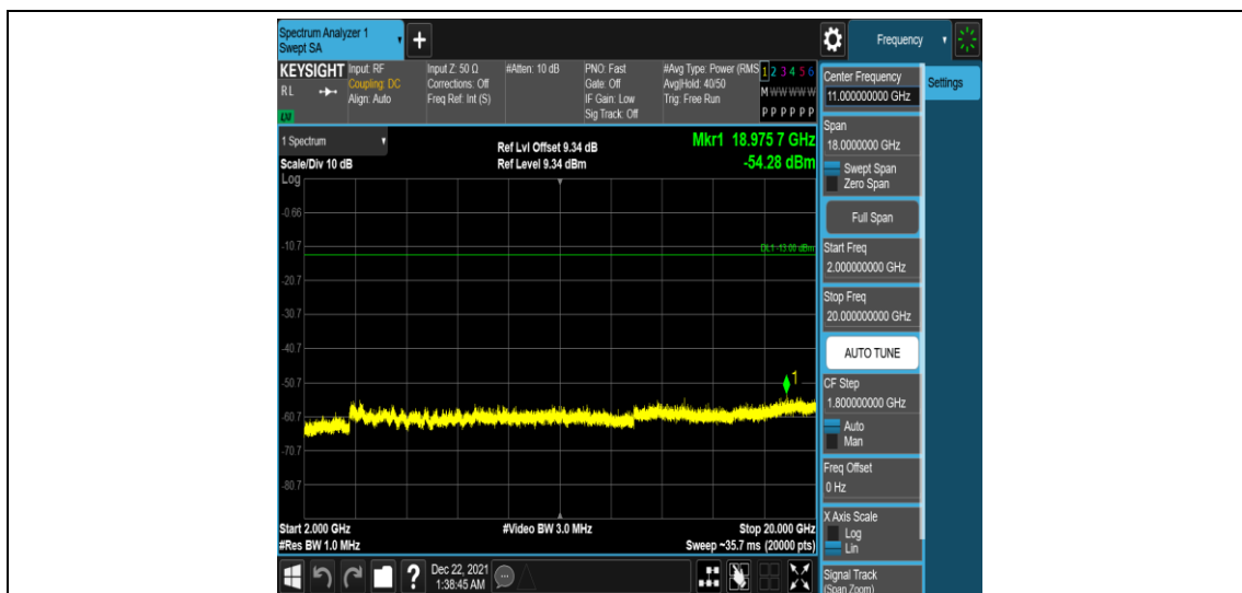
Band25-10MHz-QPSK-26090-1RB#0-Range5:2000~20000MHz
