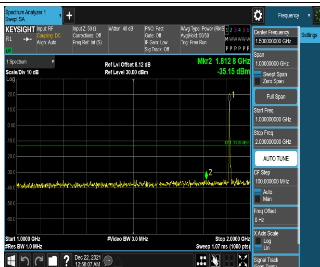
Band25-3MHz-QPSK-26675-1RB#0-Range4:1000~2000MHz
