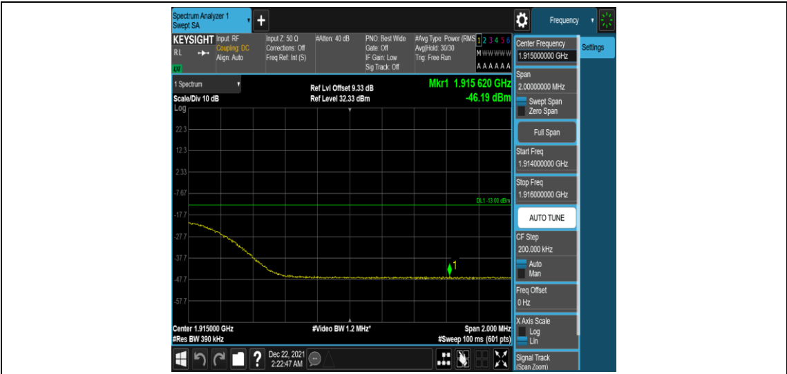
Band25-20MHz-16QAM-26590-1RB#0
