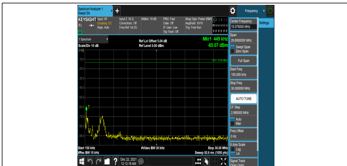
Band13-10MHz-QPSK-23230-1RB#0-Range2:0.15~30MHz
