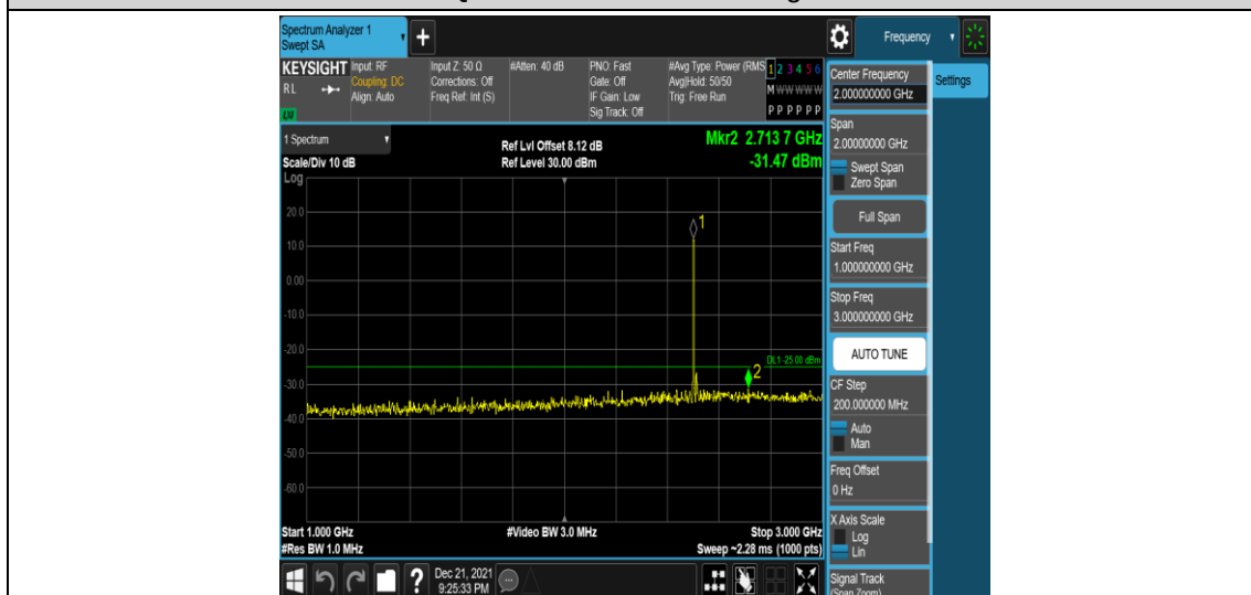
Band7-15MHz-QPSK-20825-1RB#0-Range4:1000~3000MHz
