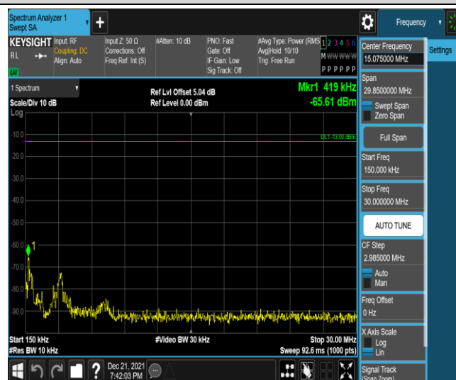
Band5-3MHz-QPSK-20635-1RB#0-Range2:0.15~30MHz
