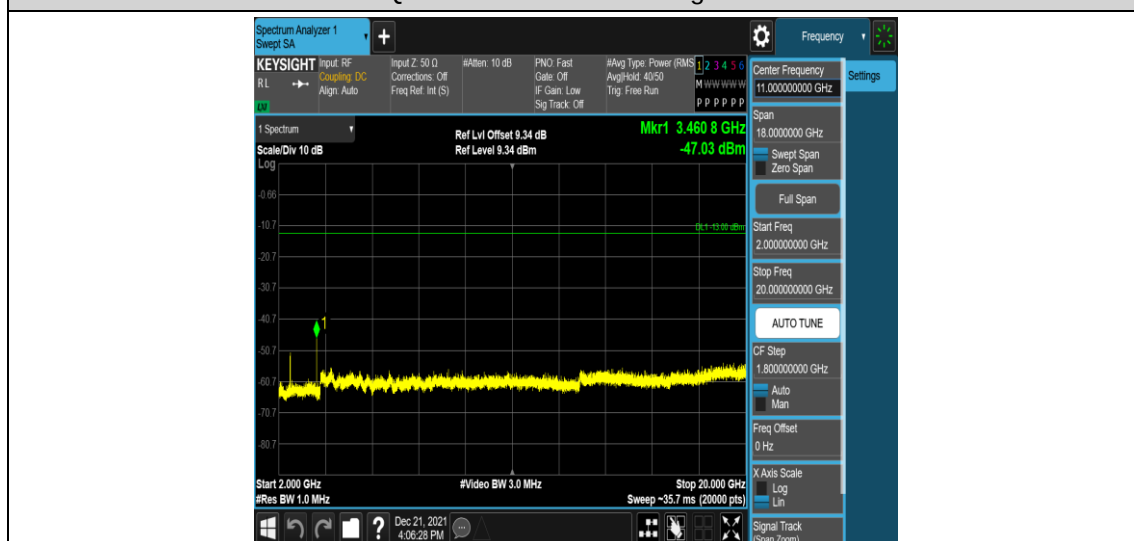
Band4-5MHz-QPSK-20175-1RB#0-Range5:2000~20000MHz
