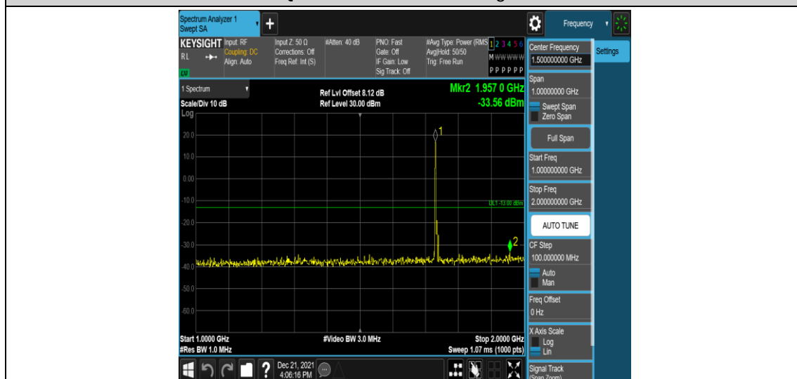
Band4-5MHz-QPSK-20175-1RB#0-Range4:1000~2000MHz
