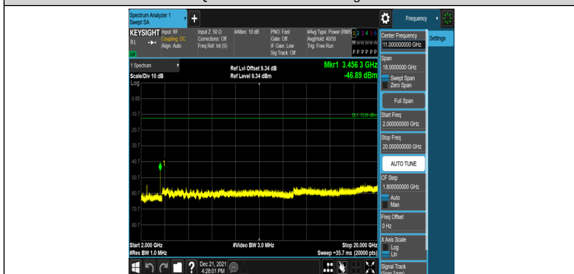
Band4-10MHz-QPSK-20175-1RB#0-Range5:2000~20000MHz
