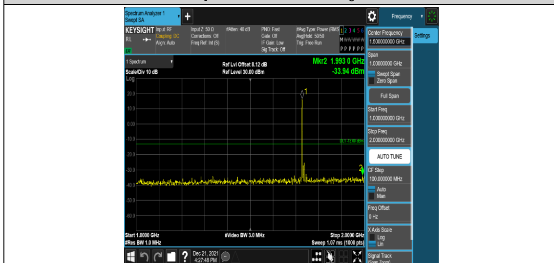
Band4-10MHz-QPSK-20175-1RB#0-Range4:1000~2000MHz
