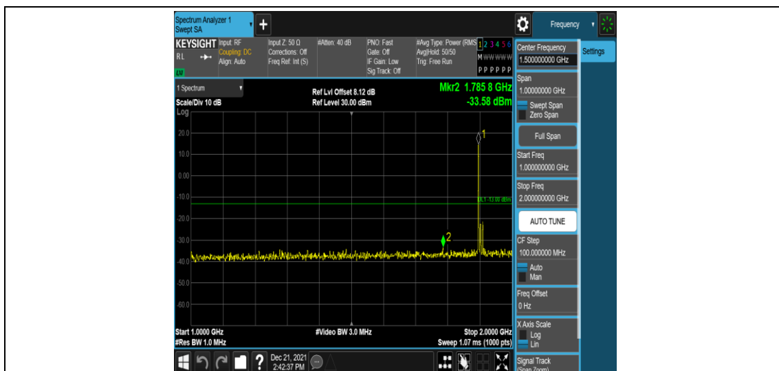
Band2-15MHz-QPSK-19125-1RB#0-Range4:1000~2000MHz
