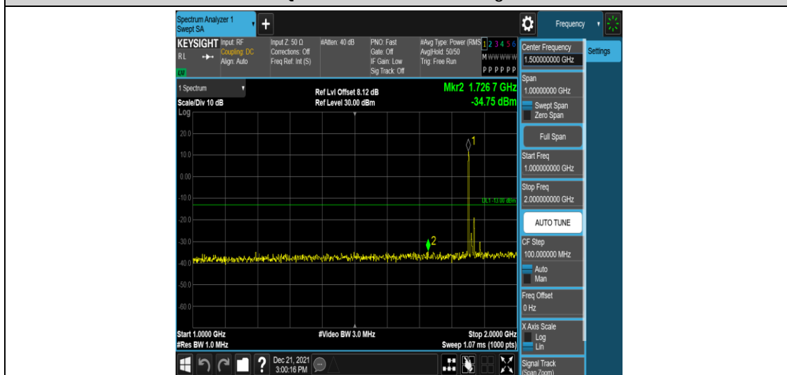
Band2-20MHz-QPSK-18700-1RB#0-Range4:1000~2000MHz
