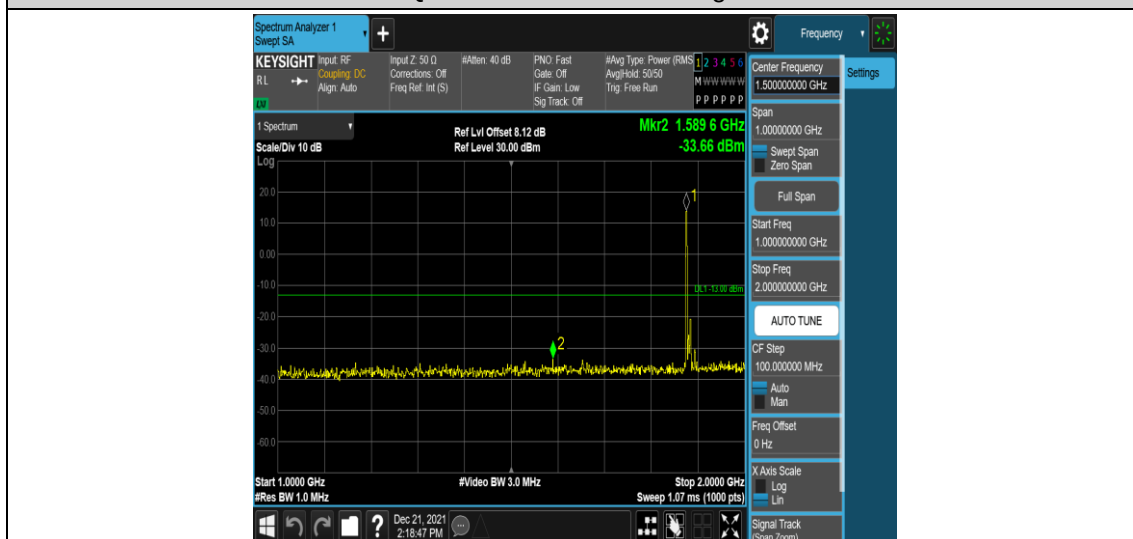
Band2-10MHz-QPSK-18900-1RB#0-Range4:1000~2000MHz
