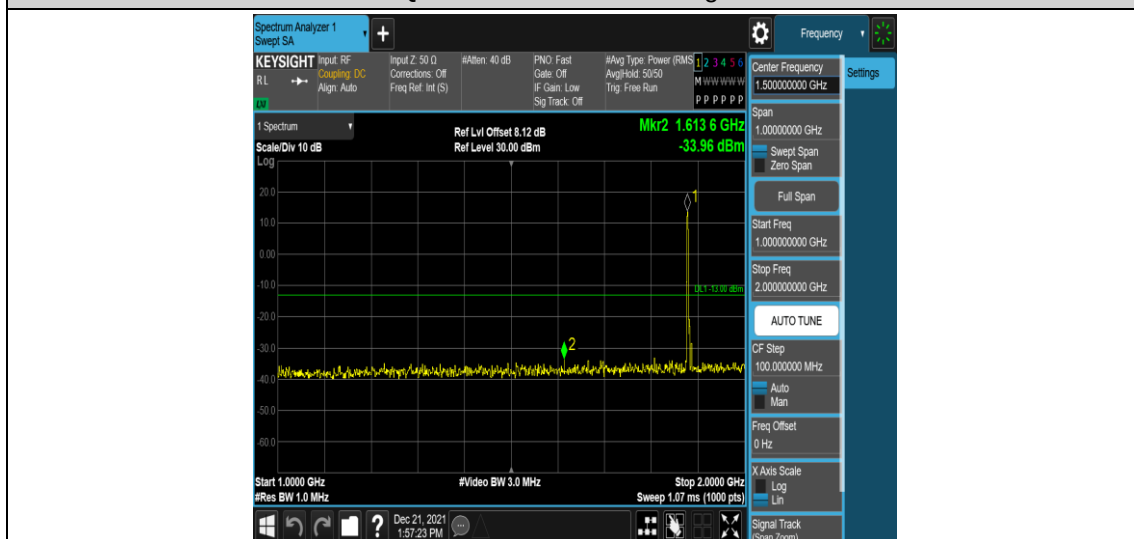
Band2-5MHz-QPSK-18900-1RB#0-Range4:1000~2000MHz
