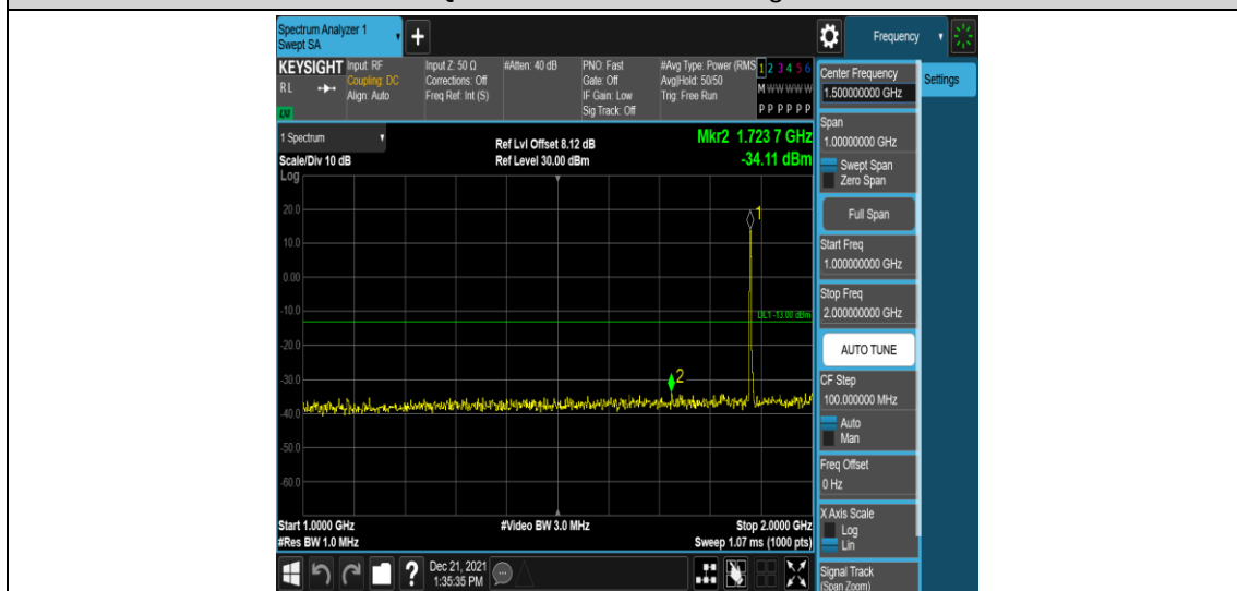
Band2-3MHz-QPSK-18900-1RB#0-Range4:1000~2000MHz
