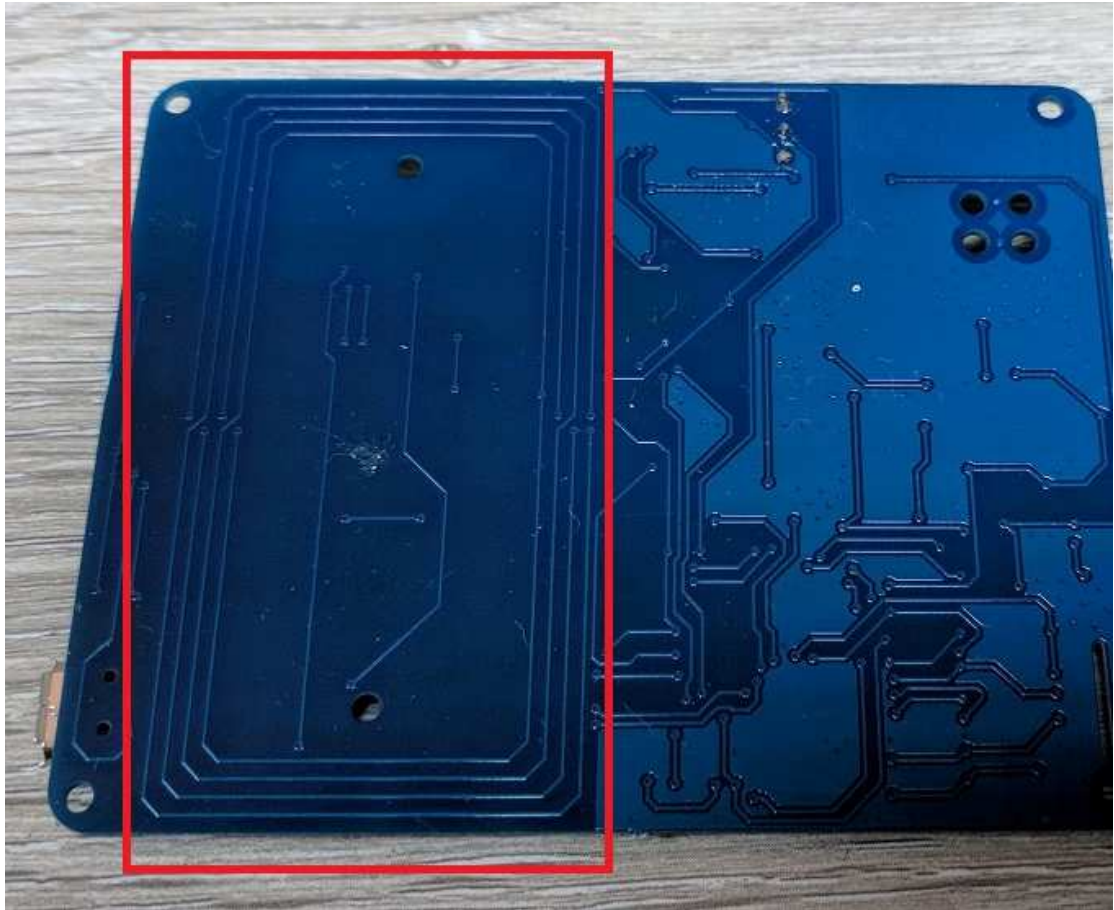
Antenna
