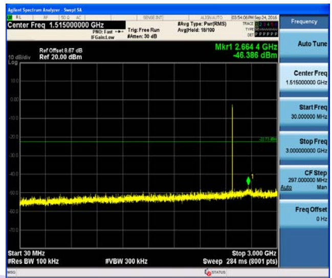
30MHz-3GHz
