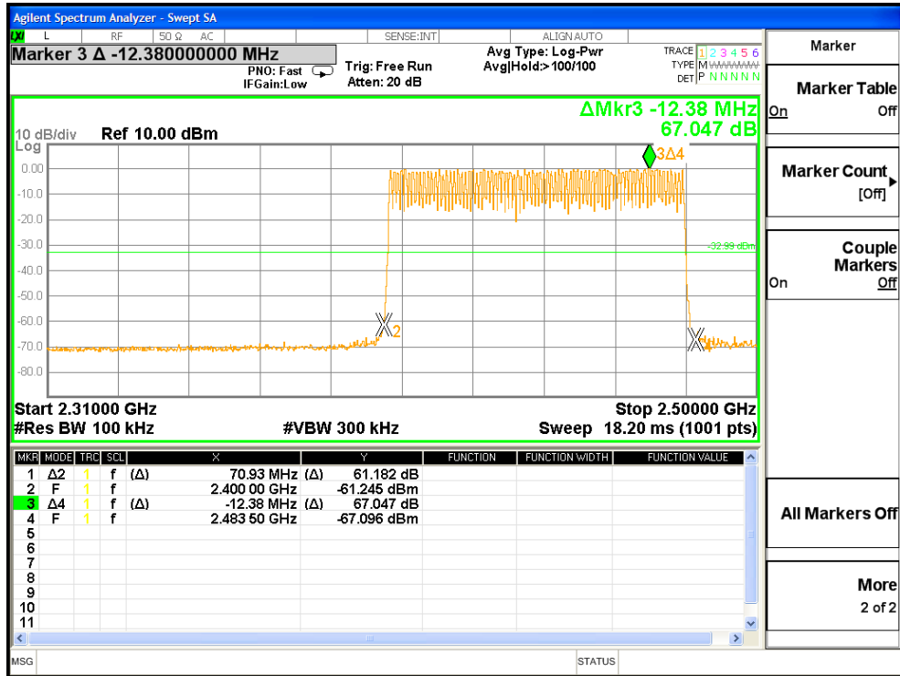
8DPSK mode
