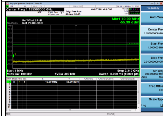
Case 31MHz~2310MHz: 802.11g,2437MHz,
