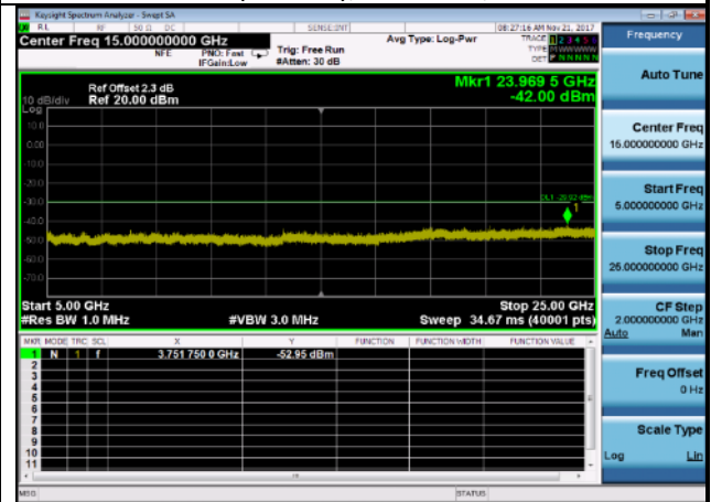
Case 55000MHz~25000MHz: 802.11n(40MHz),2437MHz, ANT 0
