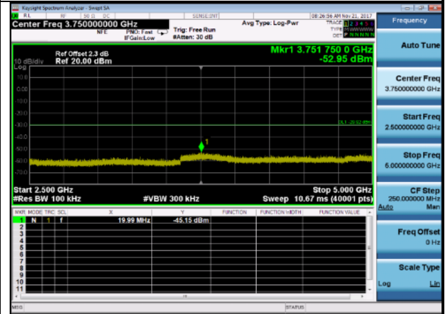
Case 4 2500MHz~5000MHz: 802.11n(40MHz),2437MHz, ANT 0
