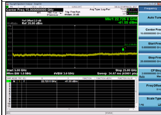
Case 55000MHz~25000MHz: 802.11n,2437MHz, ANT 1
