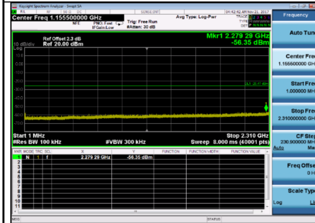
Case 31MHz~2310MHz: 802.11b,2462MHz,
