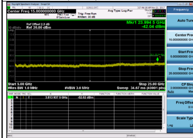
Case 55000MHz~25000MHz: 802.11n(40MHz),2437MHz, ANT 1
