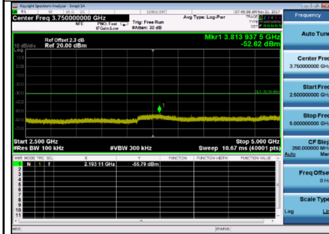
Case 42500MHz~5000MHz: 802.11n(40MHz),2437MHz,
