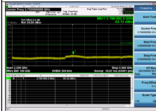
Case 42500MHz~5000MHz: 802.11n,2462MHz,
