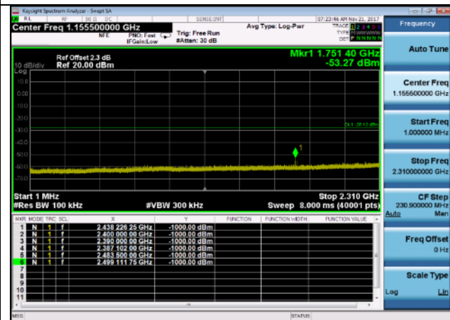
Case 31MHz~2310MHz: 802.11n,2462MHz, ANT 0
