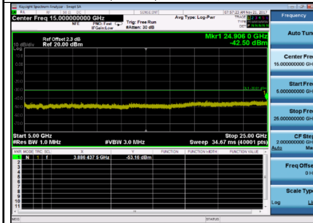
Case 55000MHz~25000MHz: 802.11n(40MHz),2452MHz, ANT 1
