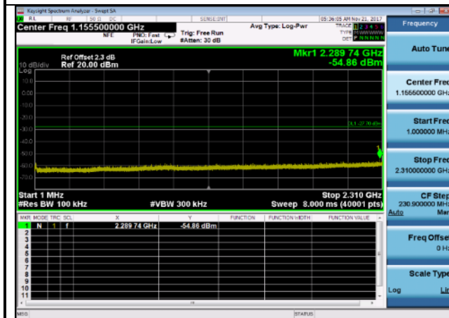
Case 31MHz~2310MHz: 802.11n,2462MHz,
