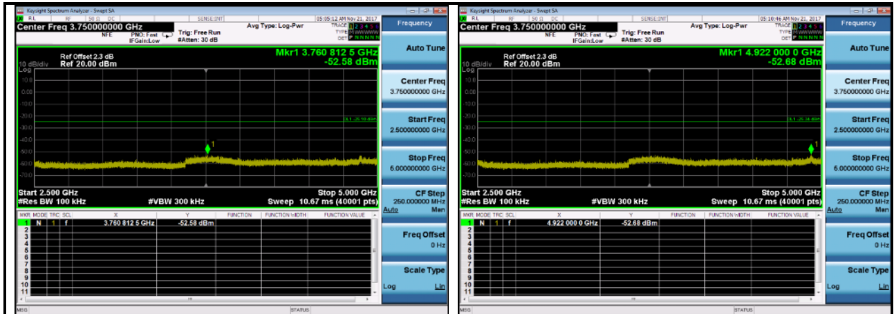
Case 4 2500MHz~5000MHz: 802.11n(40MHz),2422MHz,
