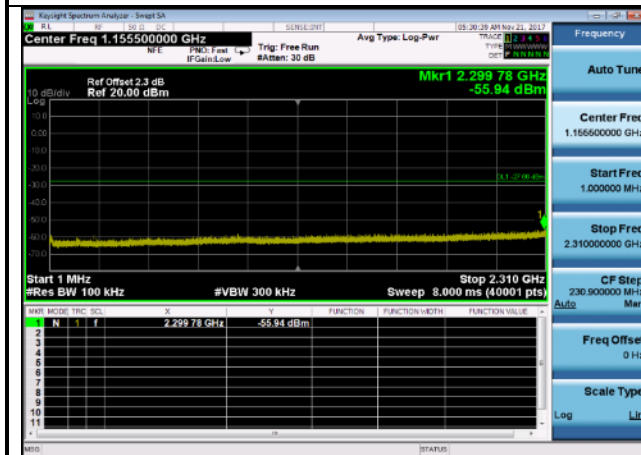
Case 31MHz~2310MHz: 802.11n,2437MHz,
