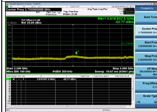
Case 42500MHz~5000MHz: 802.11n,2437MHz,
