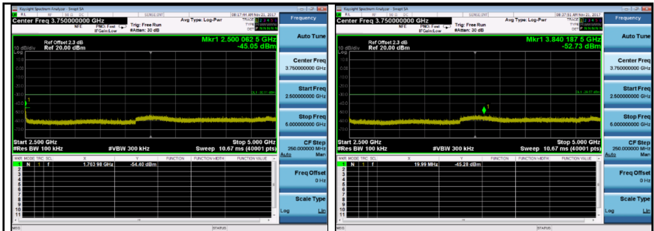
Case 42500MHz~5000MHz: 802.11n,2412MHz, ANT 0
