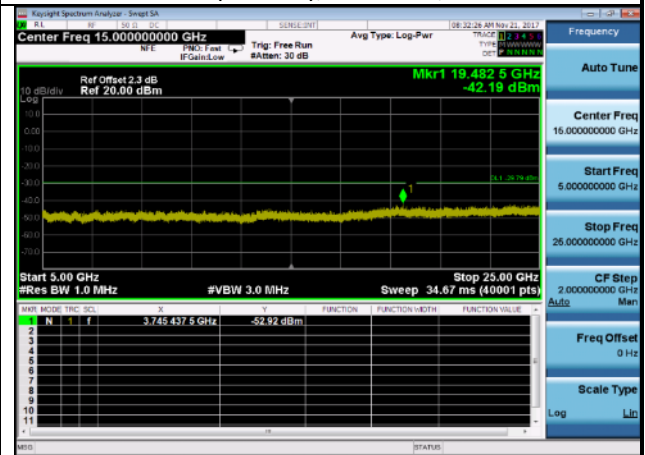
Case 55000MHz~25000MHz: 802.11n(40MHz),2452MHz, ANT 0
