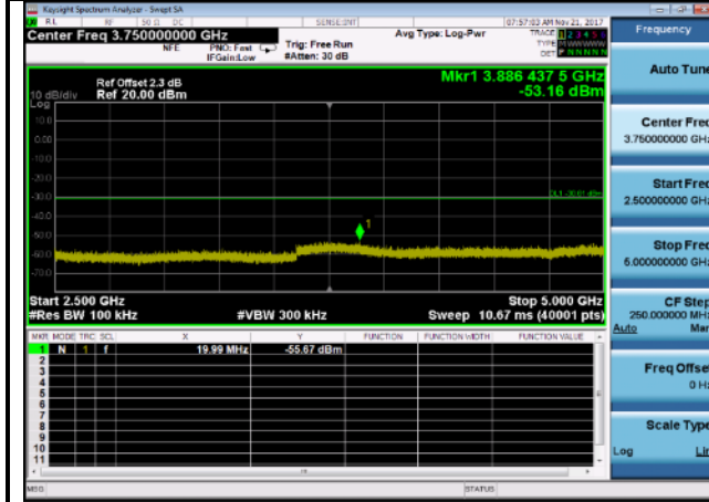
Case 42500MHz~5000MHz: 802.11n(40MHz),2452MHz,
