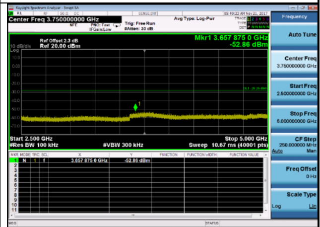
Case 42500MHz~5000MHz: 802.11n,2437MHz, ANT 0
