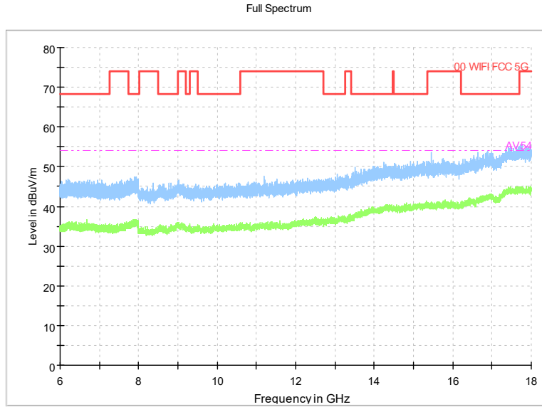
Frequency Range: 6GHz -18GHz Detector: Av mode and PK mode Modulation type: 802.11n(HT40)
