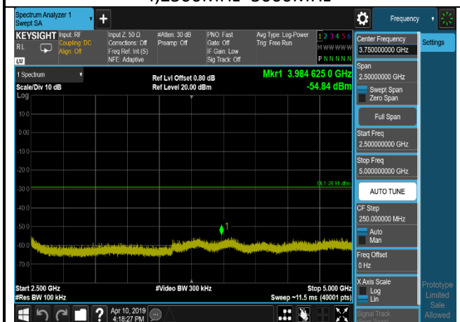
802.11n(HT40),2452MHz,Ant1,Plot 4,2500MHz~5000MHz
