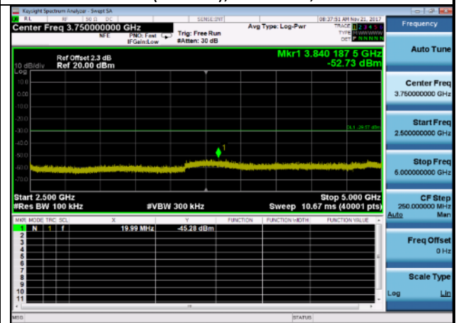
Case 42500MHz~5000MHz: 802.11n,2412MHz, ANT 0
