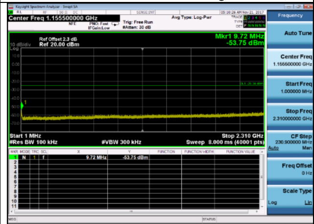
Case 31MHz~2310MHz: 802.11n(40MHz),2422MHz, ANT 0
