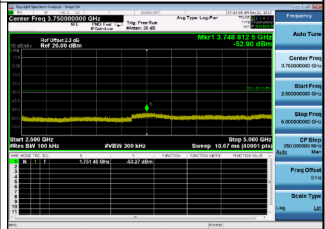
Case 42500MHz~5000MHz: 802.11n,2462MHz, ANT 0
