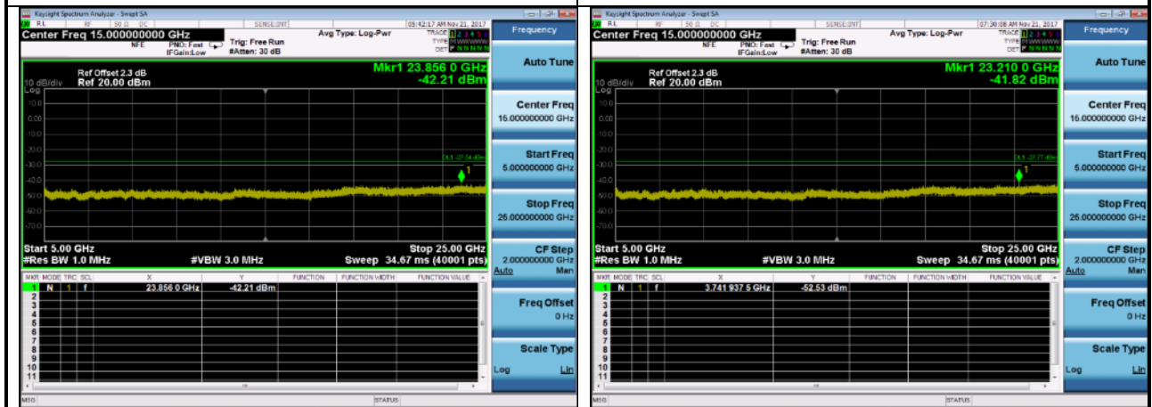
Case 55000MHz~25000MHz: 802.11n,2462MHz, ANT 1
