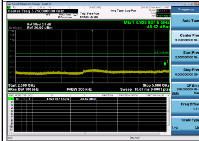
Case 42500MHz~5000MHz: 802.11g,2437MHz,
