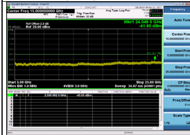
Case 55000MHz~25000MHz: 802.11n,2412MHz, ANT 1
