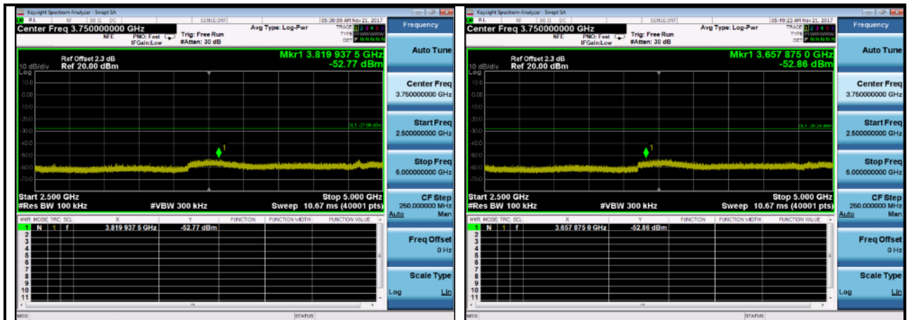
Case 42500MHz~5000MHz: 802.11n,2437MHz, ANT 0
