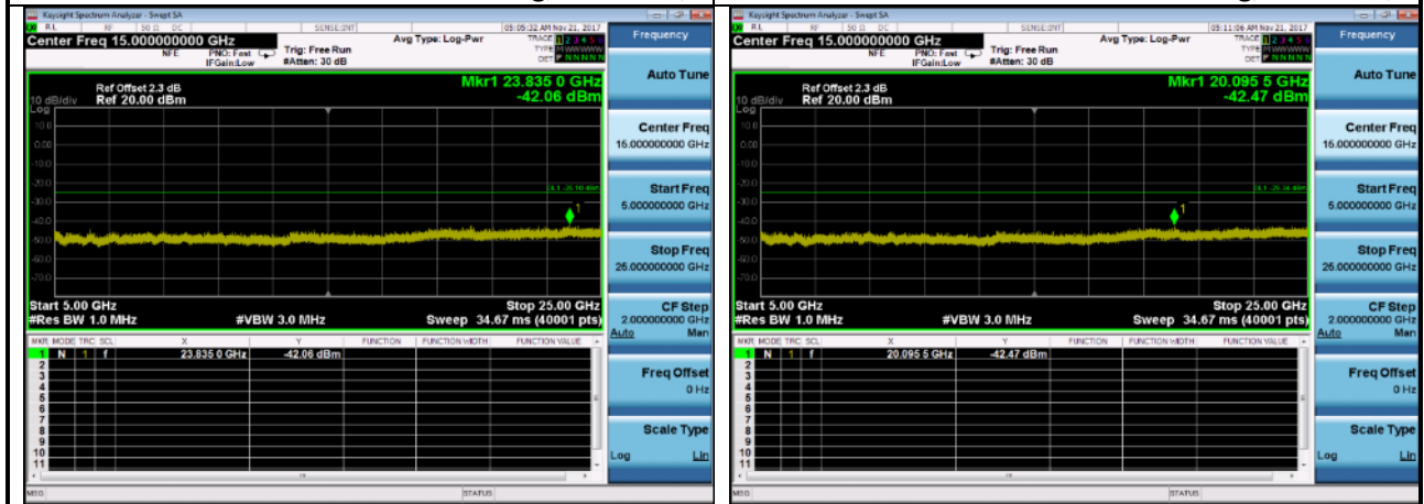
Case 55000MHz~25000MHz: 802.11n(40MHz),2422MHz, ANT 1
