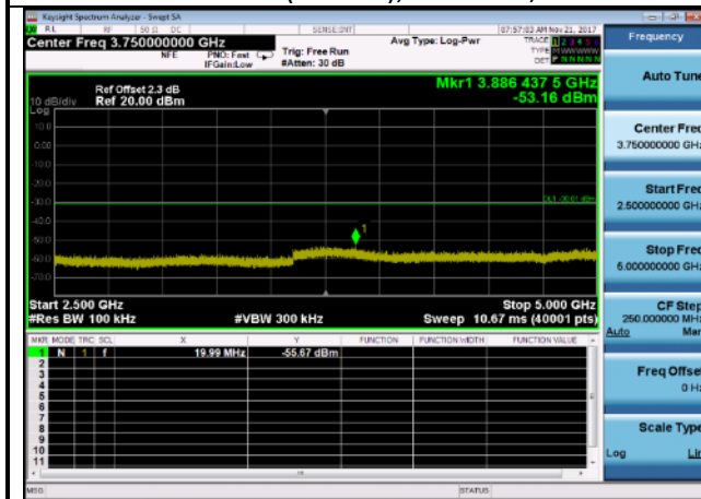
Case 42500MHz~5000MHz: 802.11n(40MHz),2452MHz,
