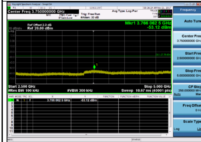
Case 42500MHz~5000MHz: 802.11n,2462MHz,
