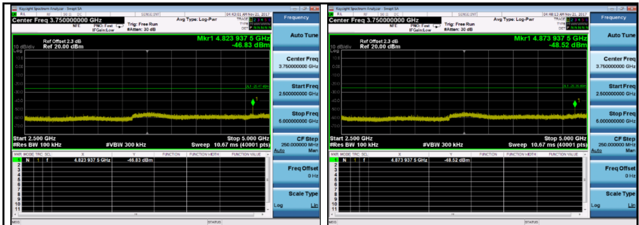
Case 42500MHz~5000MHz: 802.11b,2462MHz,
