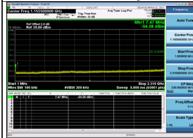
Case 31MHz~2310MHz: 802.11n(40MHz),2422MHz,
