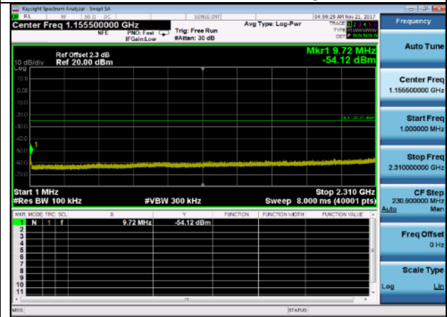
Case 31MHz~2310MHz: 802.11g,2462MHz,
