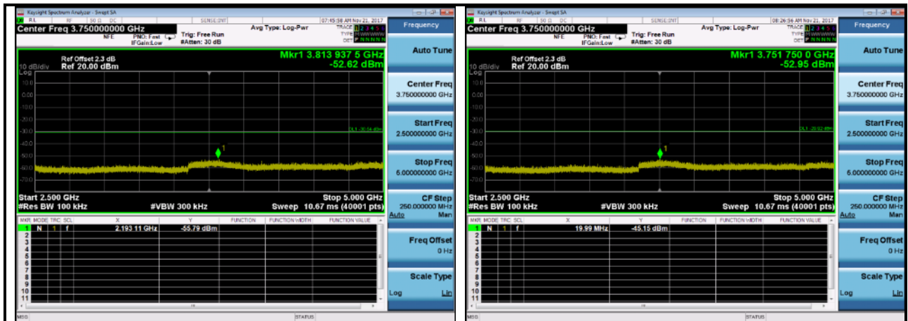
Case 42500MHz~5000MHz: 802.11n(40MHz),2437MHz,
