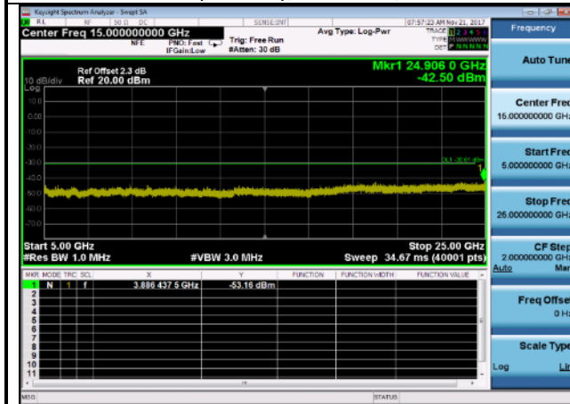
Case 55000MHz~25000MHz: 802.11n(40MHz),2452MHz, ANT 1
