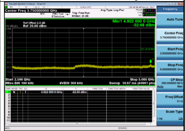
Case 4 2500MHz~5000MHz: 802.11n(40MHz),2422MHz, ANT 0
