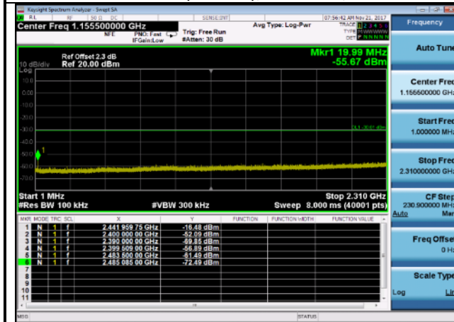
Case 31MHz~2310MHz: 802.11n(40MHz),2452MHz,
