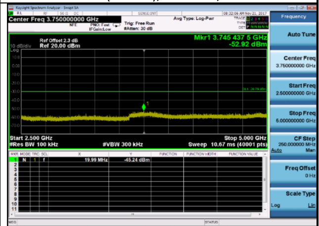
Case 42500MHz~5000MHz: 802.11n(40MHz),2452MHz, ANT 0
