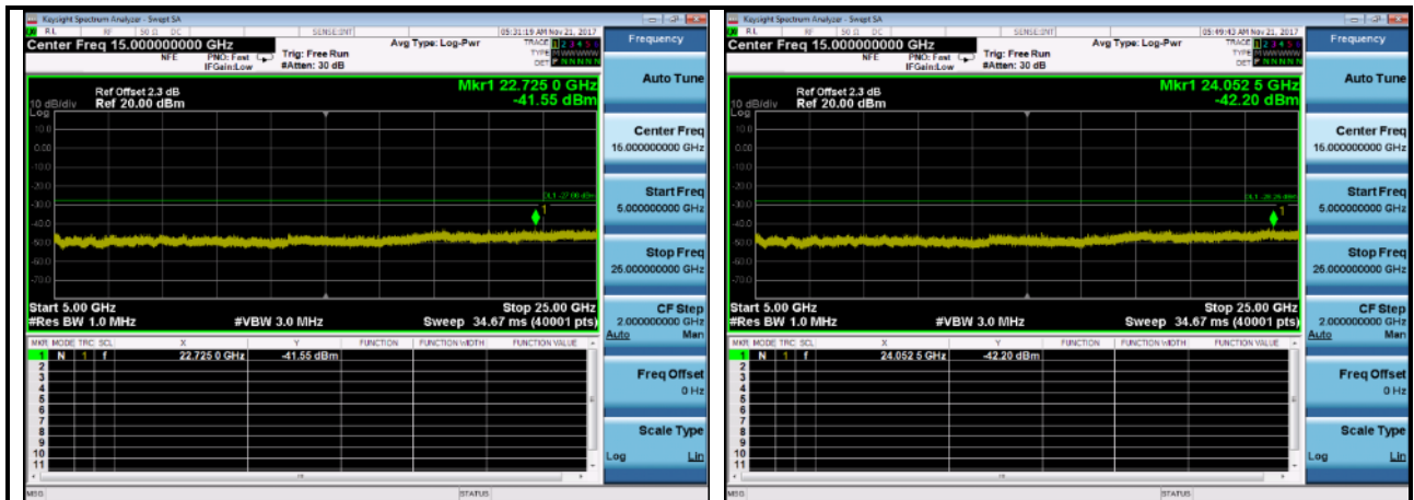
Case 55000MHz~25000MHz: 802.11n,2437MHz, ANT 1
