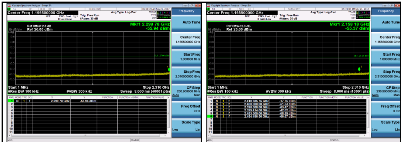
Case 31MHz~2310MHz: 802.11n,2437MHz, ANT 0
