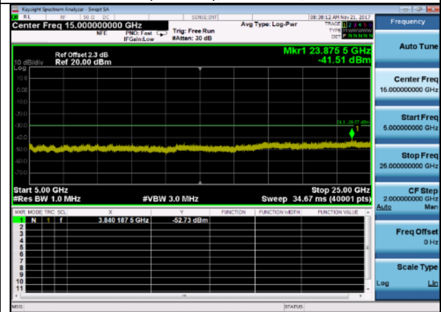
Case 55000MHz~25000MHz: 802.11n,2412MHz, ANT 0
