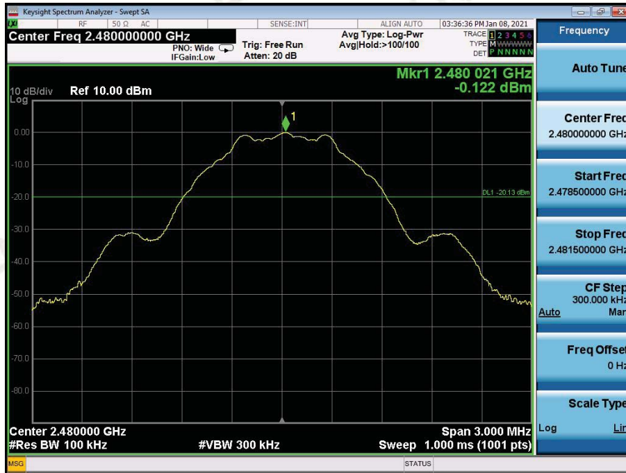
CH: 2480MHz
