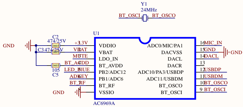
MCU : AC6969A
