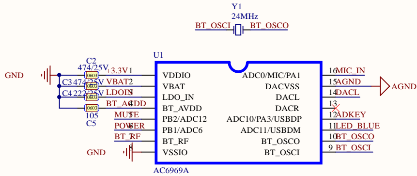
MCU : AC6969A
