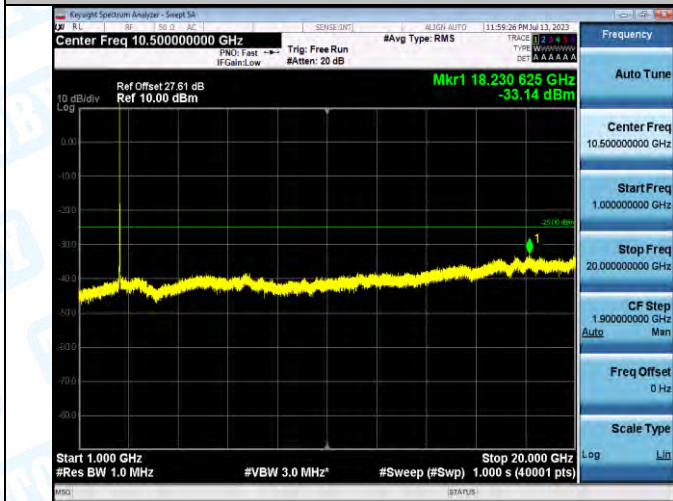
Band7_Band7_20MHz_16QAM_21350_1RB#0_1000-20000_1000-20000
