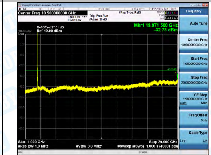
Band7_Band7_20MHz_16QAM_20850_1RB#0_1000-20000_1000-20000
