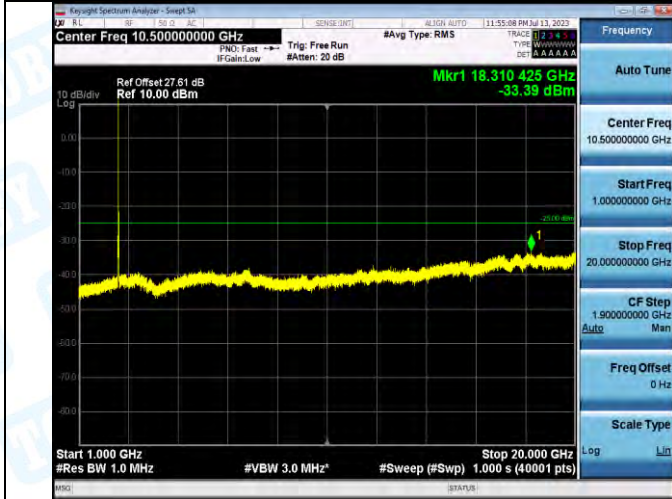
Band7_Band7_20MHz_QPSK_20850_1RB#0_1000-20000_1000-20000
