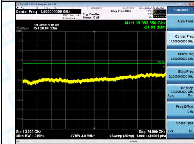
Band2_Band2_3MHz_QPSK_18615_1RB#0_3000-20000_3000-20000
