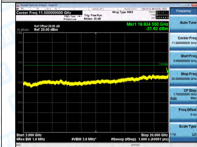
Band2_Band2_10MHz_QPSK_18650_1RB#0_3000-20000_3000-20000
