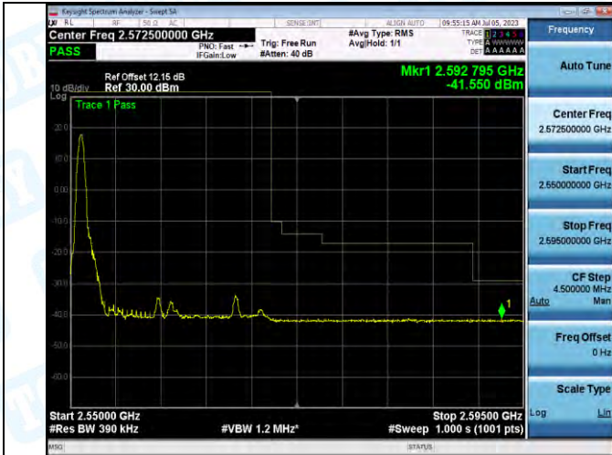
Band7_Band7_20MHz_QPSK_21350_1RB#0
