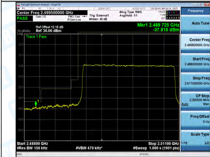
Band41_Band41_15MHz_QPSK_39725_75RB#0
