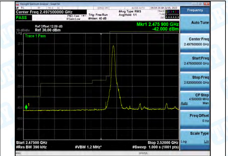
Band7_Band7_20MHz_16QAM_20850_1RB#0
