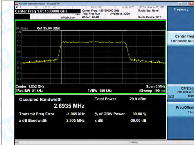
Band2-3MHz-QPSK-18615-15RB#0-PASS
