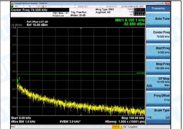
GPRS1900-810-0-0.009~0.15MHz-PASS
