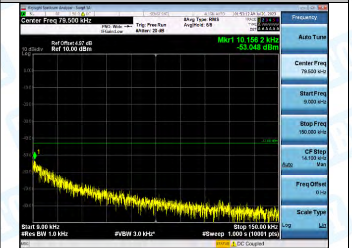
EGPRS1900-661-2-0.009~0.15MHz-PASS
