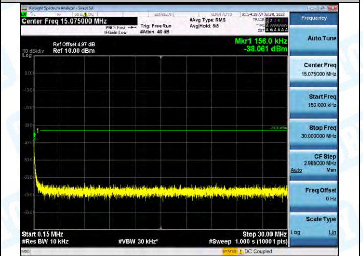
EGPRS1900-810-2-0.15~30MHz-PASS
