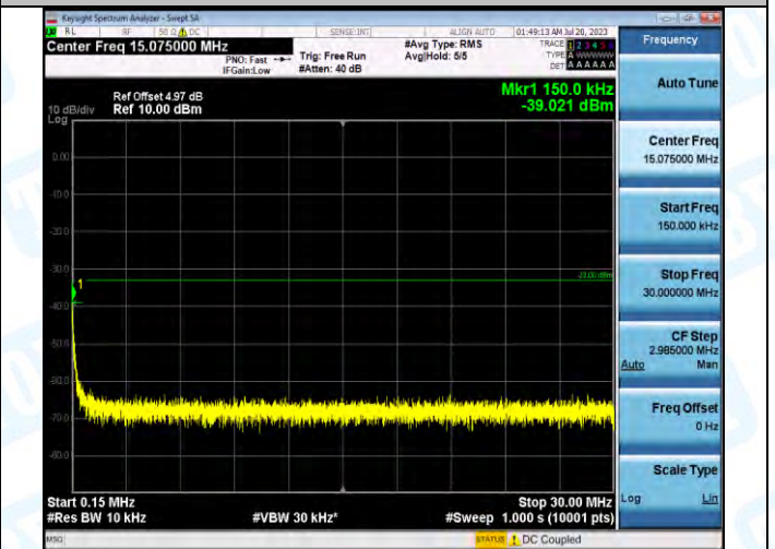
GPRS1900-661-0-0.15~30MHz-PASS
