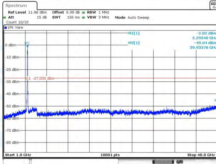
11AC80SISO_Ant1_5290_1000~40000
