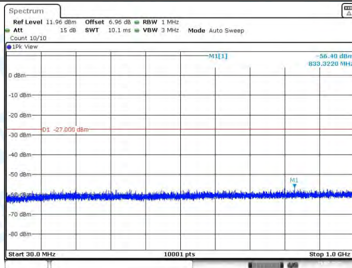
11AC80SISO_Ant1_5530_30~1000
