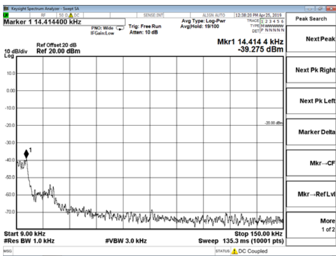
9 KHz – 150 KHz
