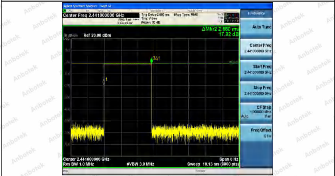
DH5_Ant1_Hop
