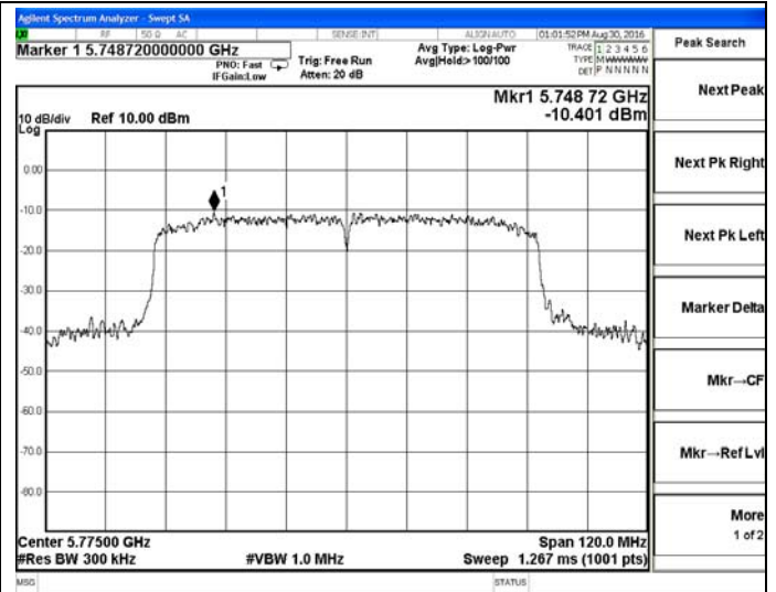
802.11ac80-5775MHz
