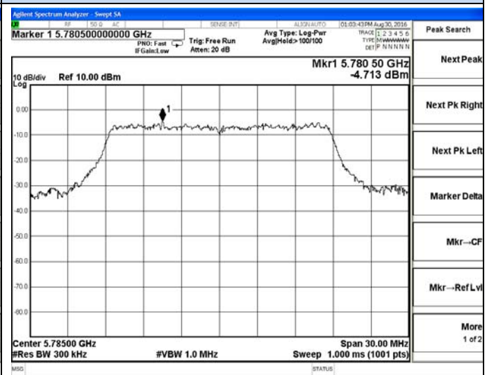
802.11ac20-5785MHz
