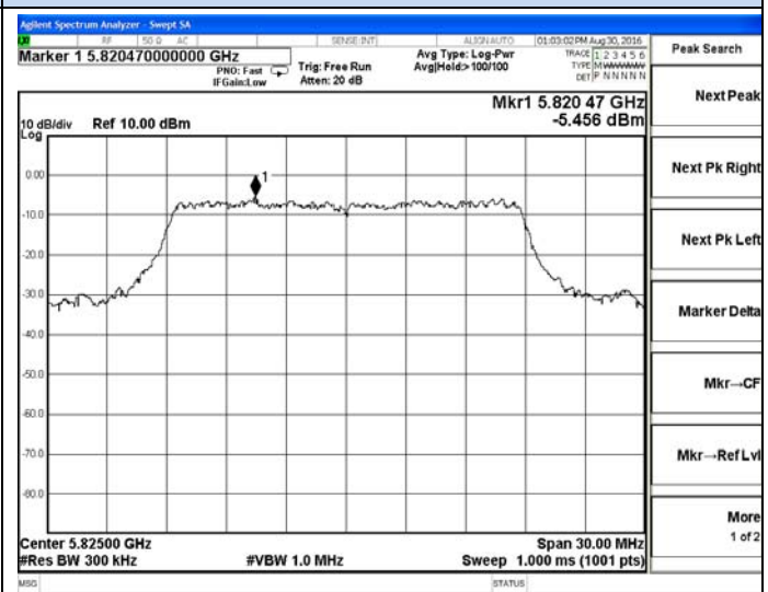
802.11ac20-5825MHz
