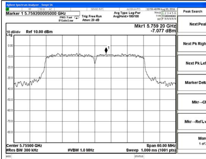
802.11nac40-5755MHz
