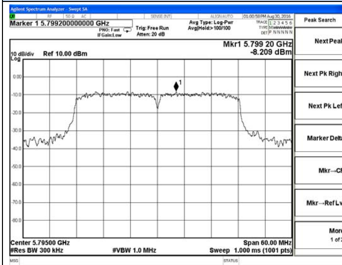
802.11ac40-5795MHz
