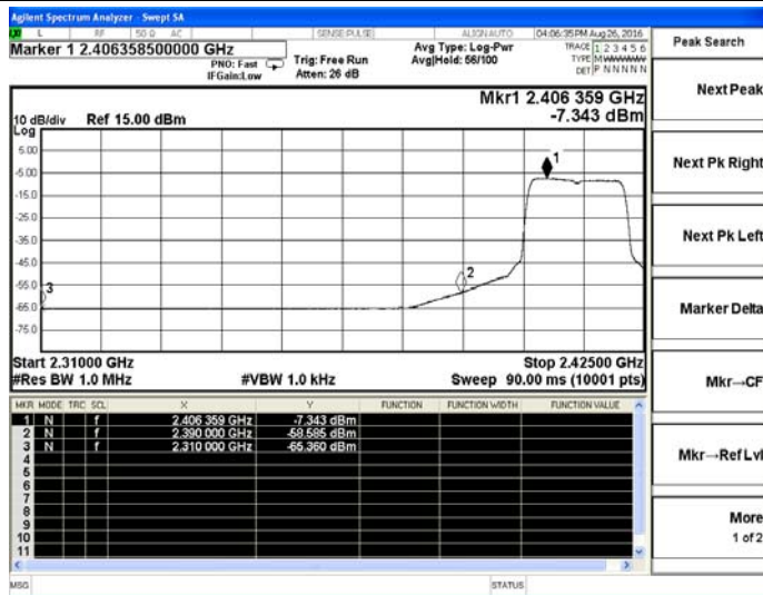
802.11n(HT20)-Low channel(Average)
