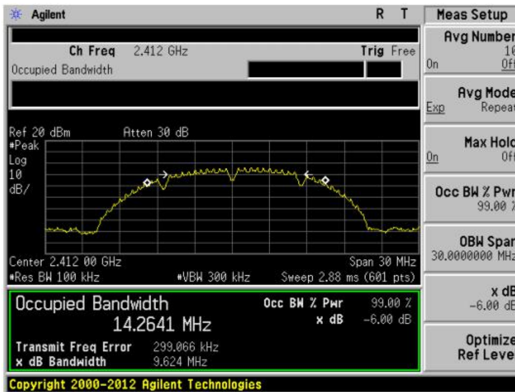
802.11b-CH2412MHZ
