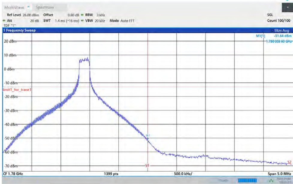
Band66-20MHz-QPSK-132572-100RB#0
